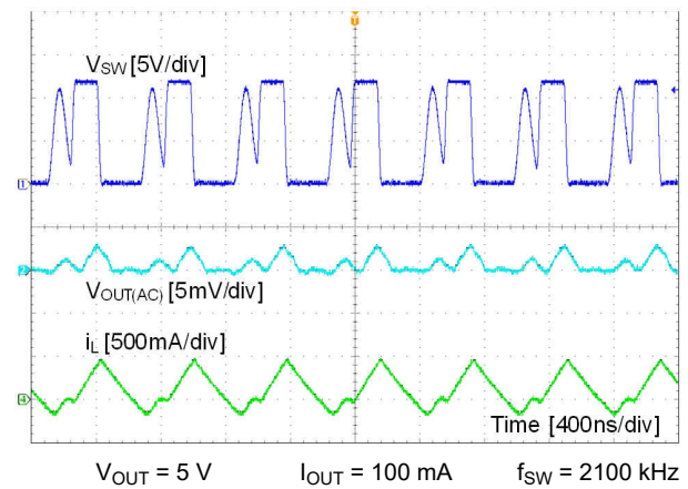
图 8-3. DCM Mode
