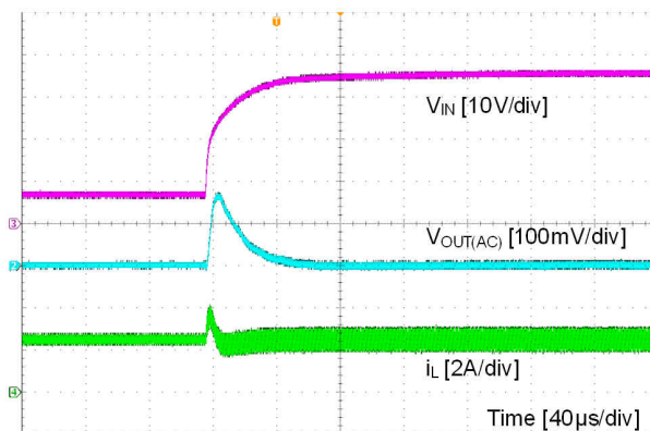
图 8-9. Line Transient
