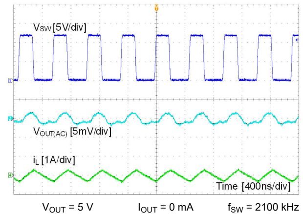
图 8-5. FPWM Mode
