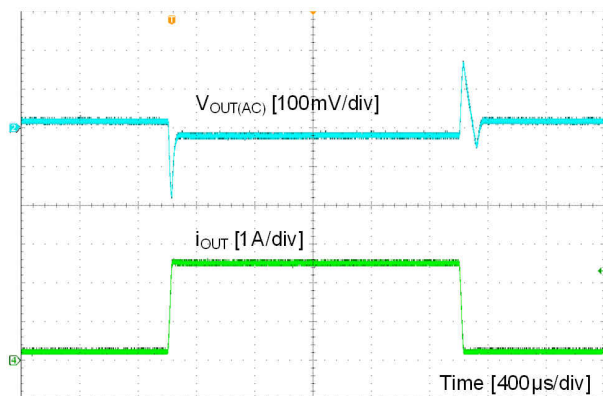
图 8-8. Load Transient
