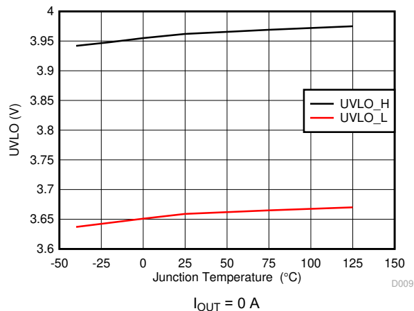
图 6-12. UVLO Threshold
