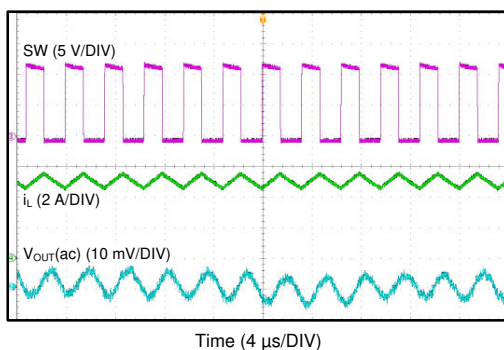
图 7-6. CCM 模式
