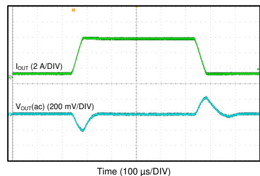
图 7-5. DCM 模式
