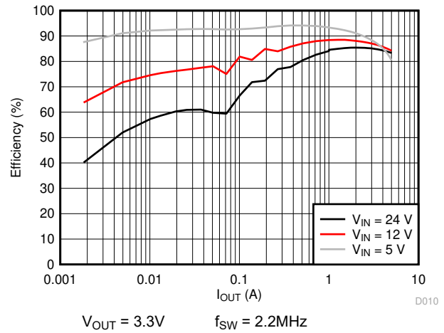
图 5-4. 效率与负载电流之间的关系
