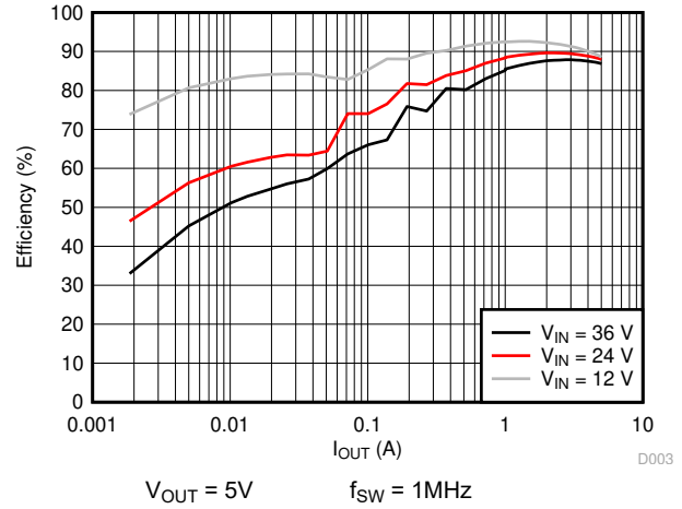
图 5-2. 效率与负载电流之间的关系
