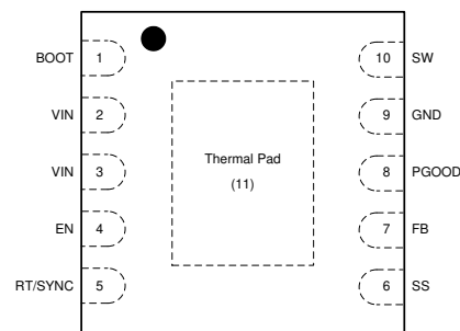
图 4-2. DPR 封装 10 引脚 (WSO) 顶视图
