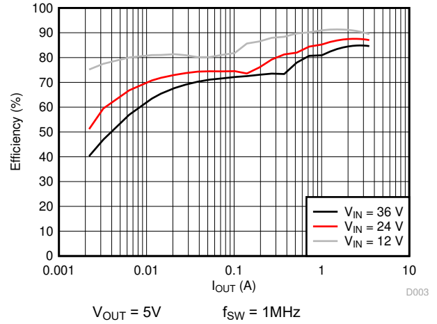
图 5-2. 效率与负载电流间的关系
