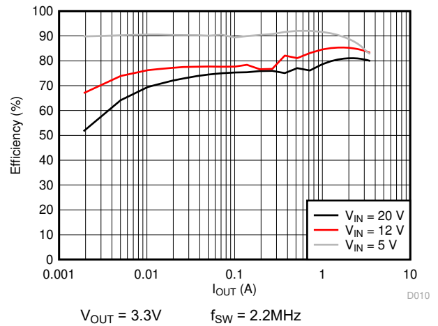
图 5-4. 效率与负载电流间的关系
