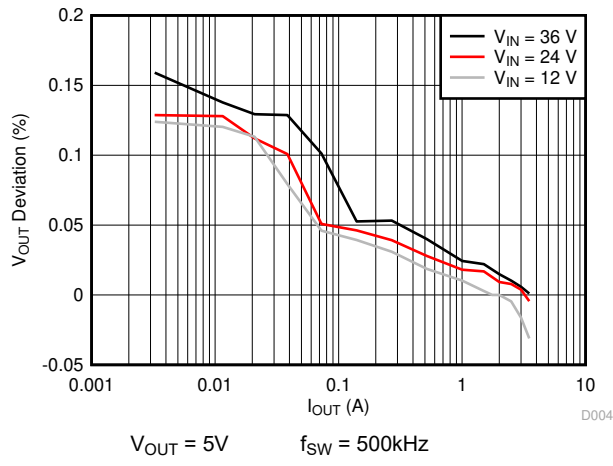
图 5-5. 负载调整率
