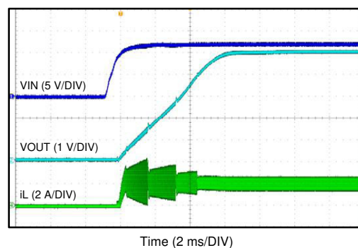
图 7-3. 由 V_{IN} 启动
