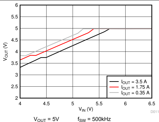
图 5-7. 压降曲线
