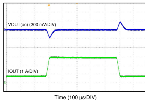
图 7-5. DCM 模式
