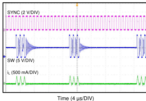
图 6-8. 在睡眠模式下同步
