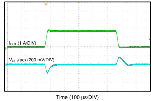
I_{OUT} : 2A \text{ 的 } 10\% \quad \text{压摆率} = 100mA/\mu s \rightarrow 100\%
