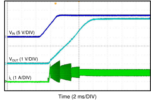
V_{IN} = 12V V_{OUT} = 5V I_{OUT} = 1A 图 7-3. 由 VIN 启动
