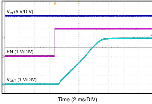
V_{IN} = 12V V_{OUT} = 5V I_{OUT} = 1A 图 7-2. 由 EN 启动
