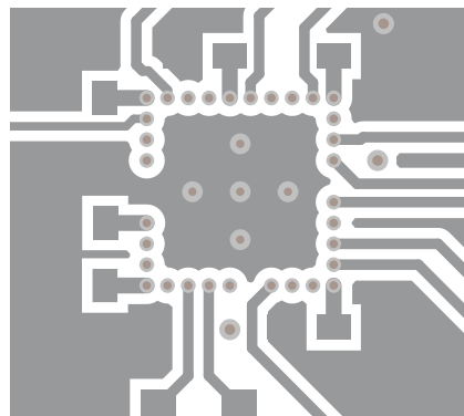
图 10-7. LMKDB1120 和 LMKDB1120FS 布局示例 - 底层
