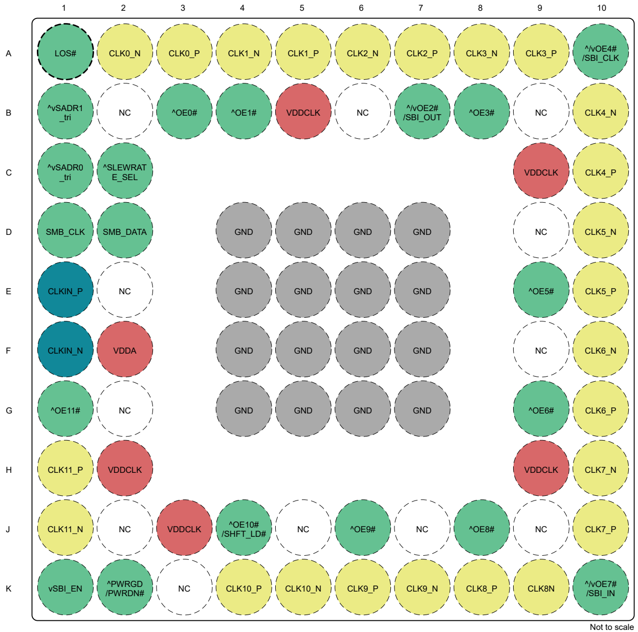
图 5-3. LMKDB1112 5mm x 5mm 封装 64 引脚 LGA ( 顶视图 )
