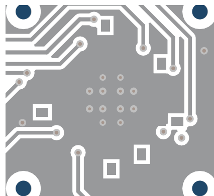
图 10-9. LMKDB1108 和 LMKDB1108FS 布局示例 - 底层
