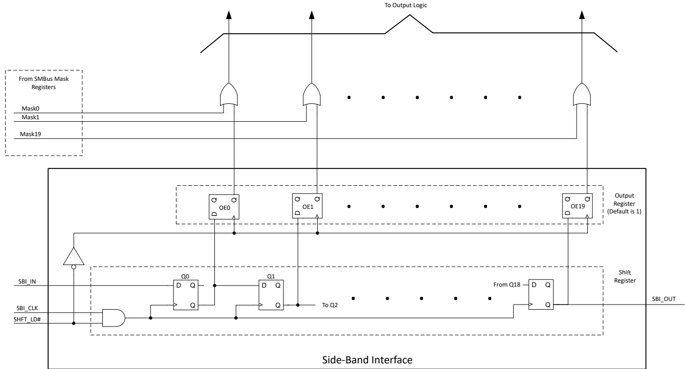
图 8-12. SBI 控制逻辑
