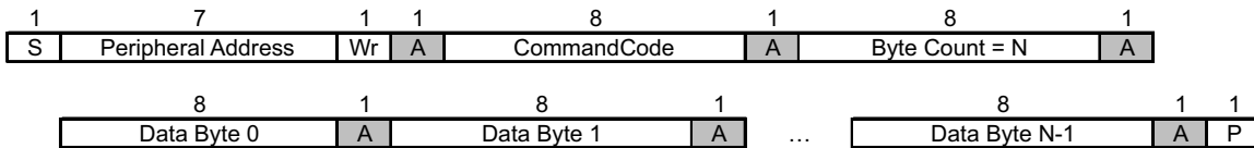
图 8-10. 块写入协议
