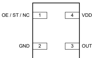
图 5-2. LMK6C 4 引脚 VSON ( 顶视图 )
