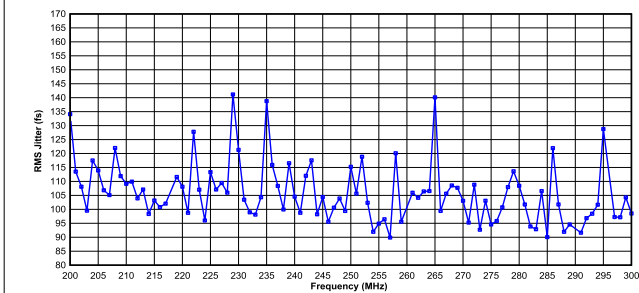
图 6-17. LVPECL、HCSL 的 RMS 抖动与频率 (200MHz 至 300MHz) 间的关系；典型值 3.3V、25°C
