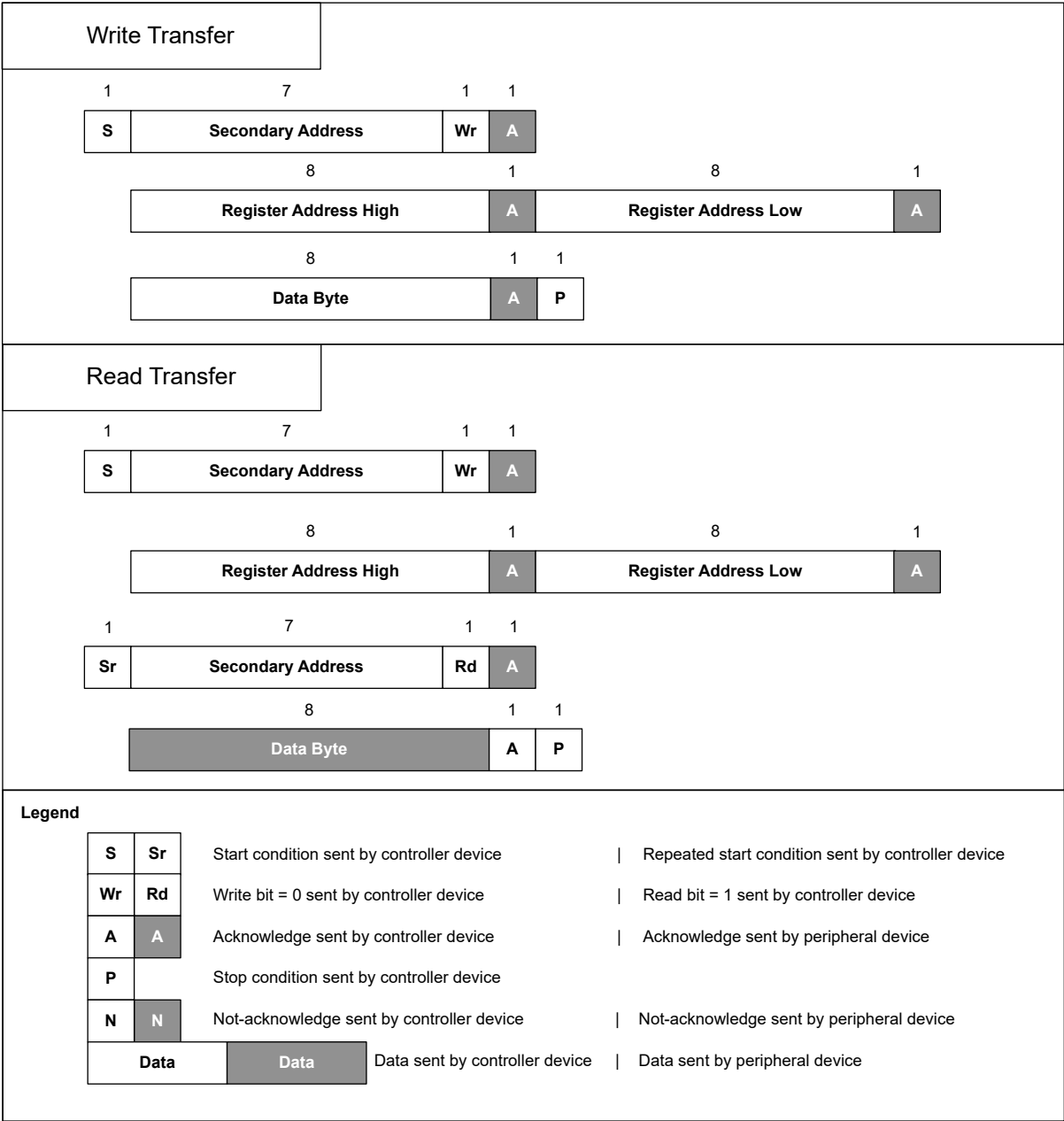
图 8-45. I²C 字节写入和读取传输
