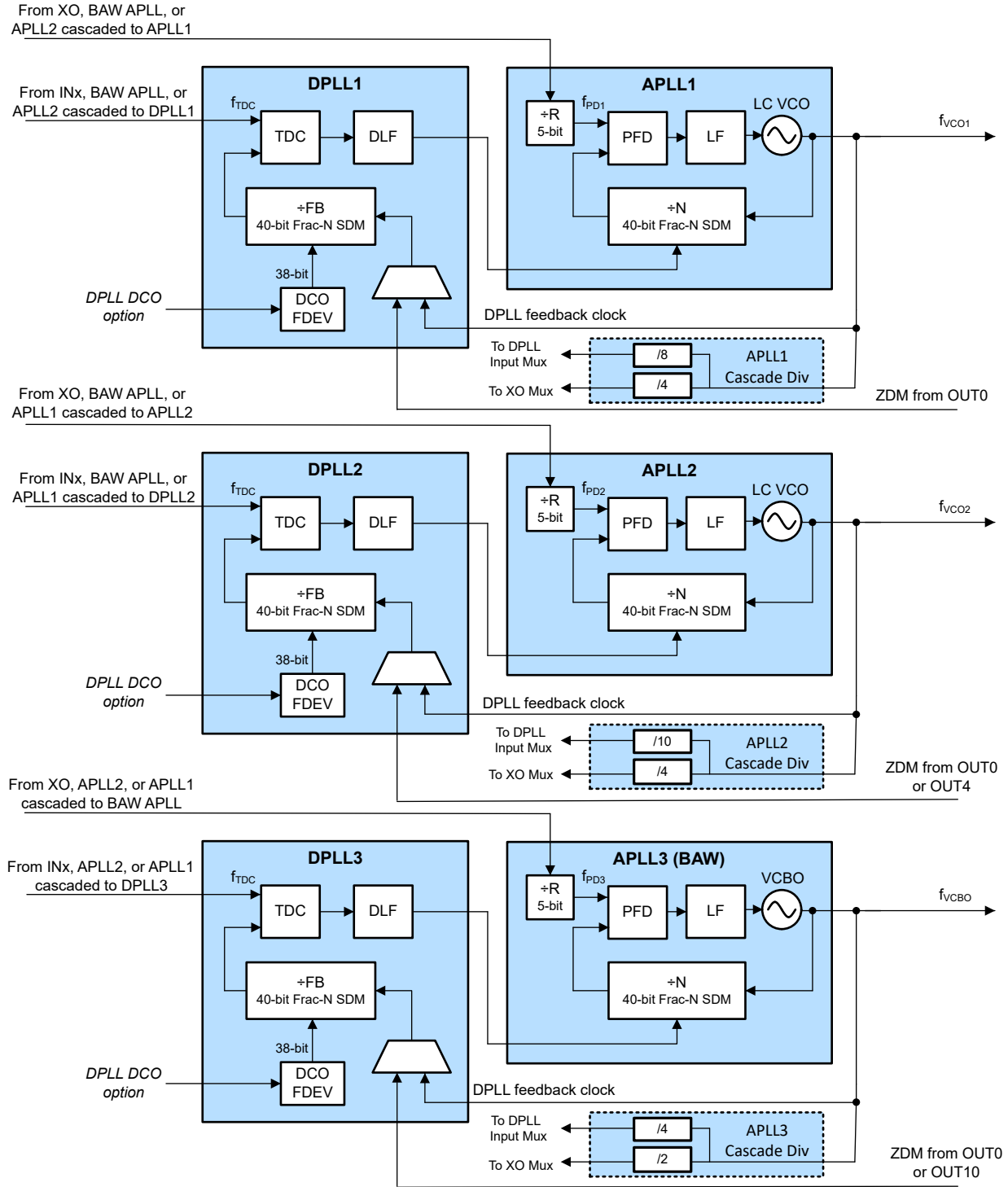
图 8-2. PLL 架构
