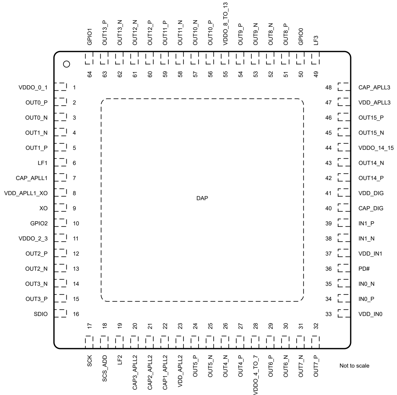
图 5-1. LMK5C33216A RGC 封装 64 引脚 VQFN 顶视图
