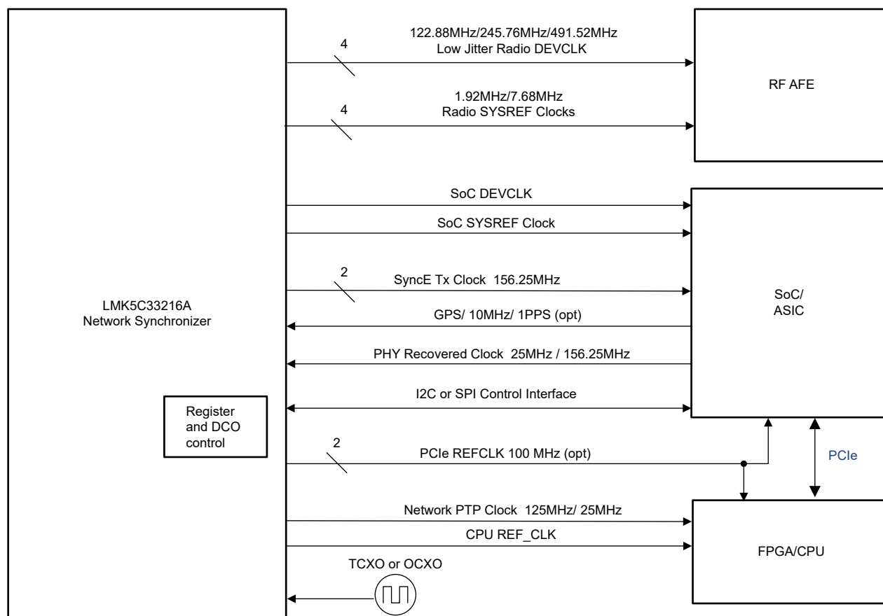
LMK5C33216A 典型系统方框图
