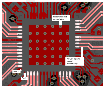
图 9-5. LMK5C33216A 的 PCB 布局示例, 顶层
