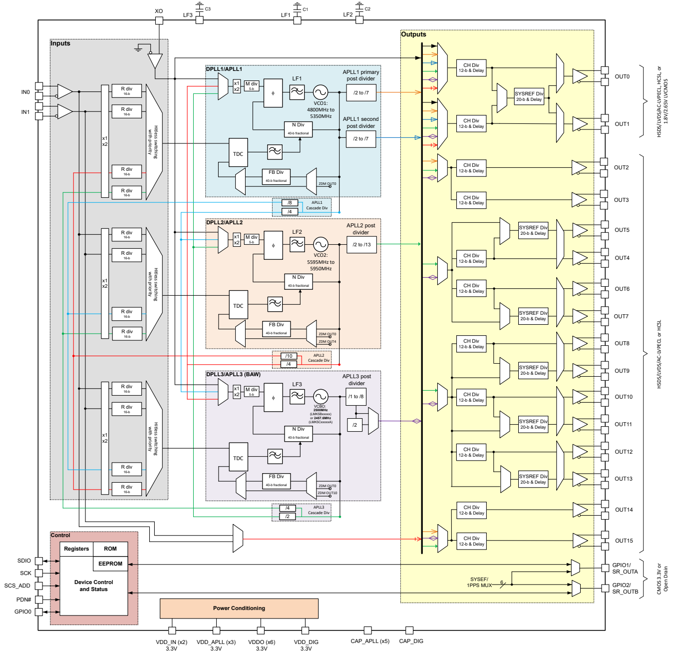
图 8-1. LMK5C33216A 顶层方框图
