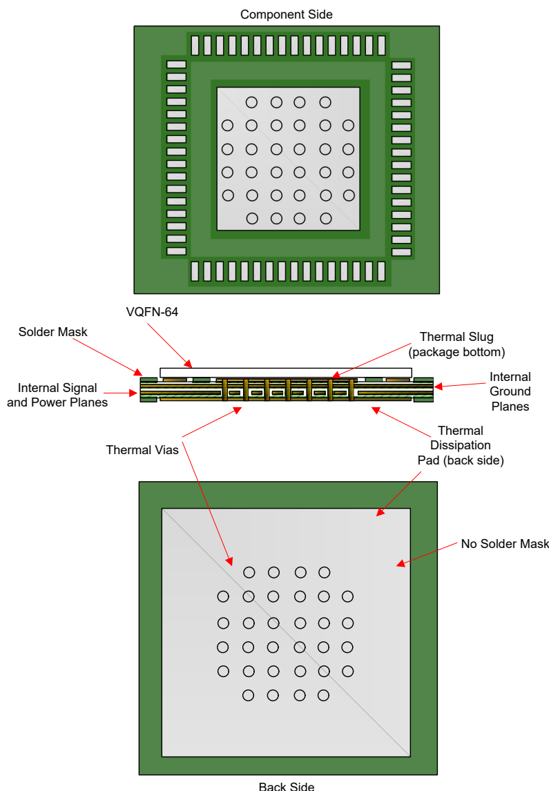
图 8-8. 可实现热可靠性的通用 PCB 接地布局（建议 8 层以上）
