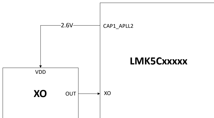
图 8-3. 为 CAP1_APLL2 提供 XO 输入
