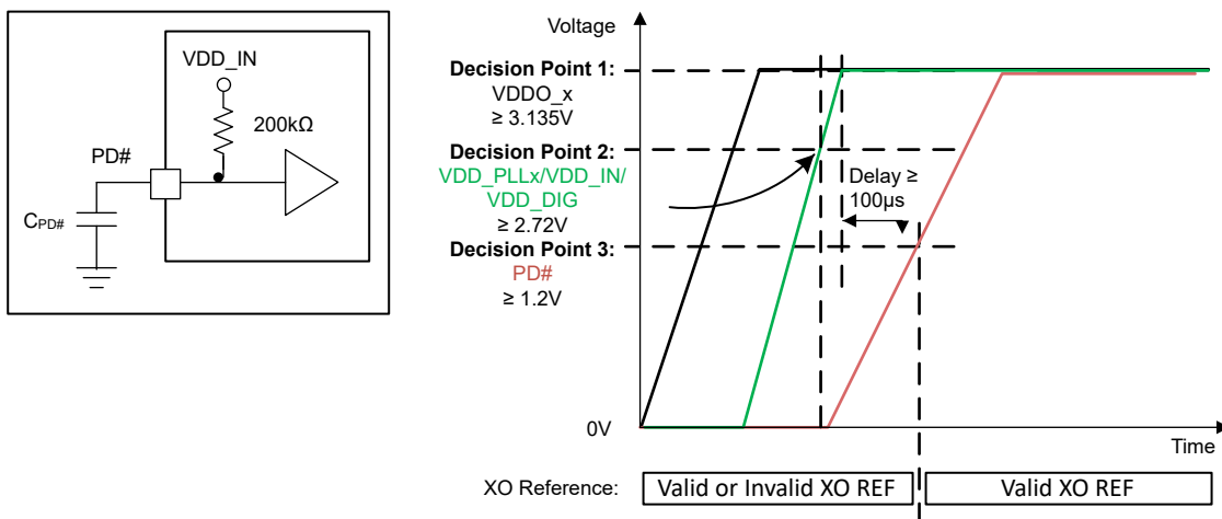
图 8-2. 从双电源轨上电的建议
