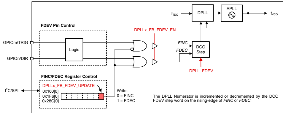
图 7-39. DCO 模式控制选项
