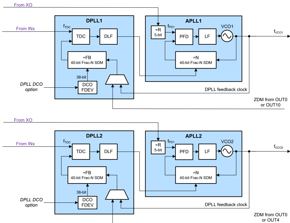
图 7-3. DPLL 操作
