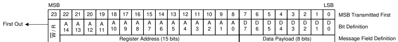
图 7-44. SPI 消息格式
