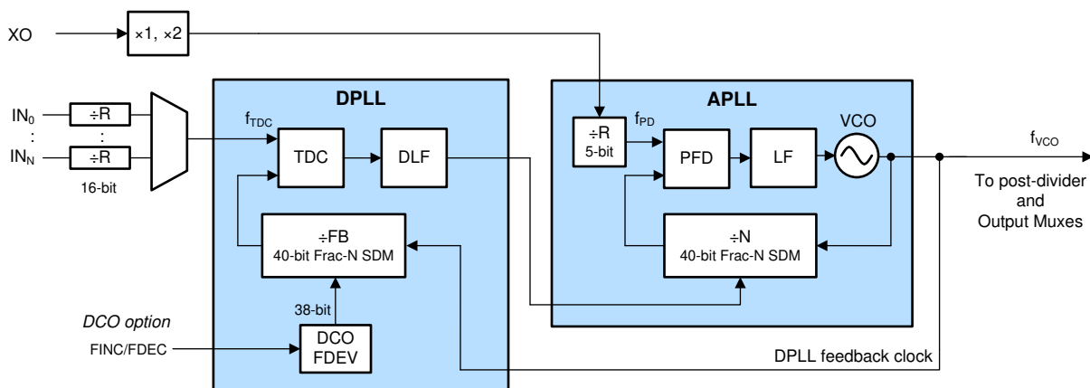
图 7-23. PLL 架构
