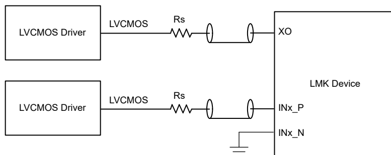
图 7-10. 单端 LVCMOS ( 1.8V、2.5V、3.3V ) 至基准 (INx_P) 或 XO 输入 (XO)
