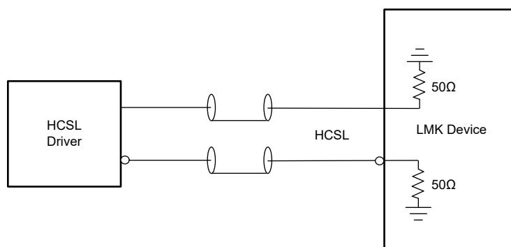
图 7-14. HCSSL (负载端接) 至基准 (INx)
