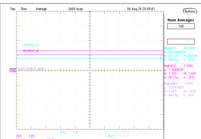
图 6-14. 2.5V/3.3V 电源条件下的 LMK1D210xL 直流输出共模，差分 低电平 (AMP_SELA/AMP_SELB = 悬空)
