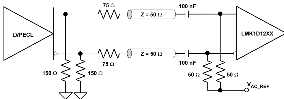
图 9-5. LVPECL 时钟驱动器连接到 LMK1D121x 输入
