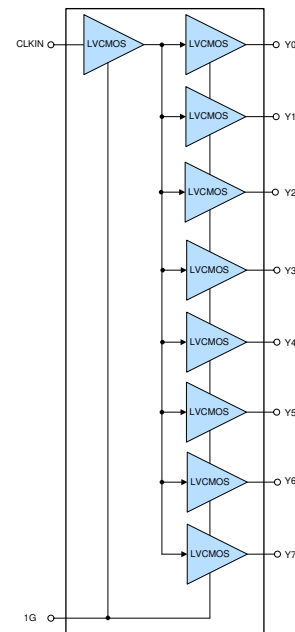
功能方框图
