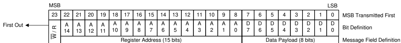
图 8-39. SPI 消息格式
