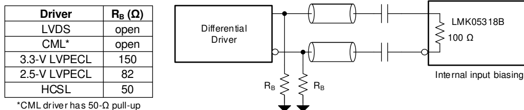
图 8-14. 差分交流耦合至基准 (PRIREF/SECREF) 或 XO 输入
