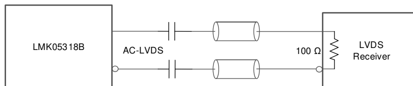
图 8-27. AC-LVDS 输出至带内部端接/偏置的 LVDS 接收器
