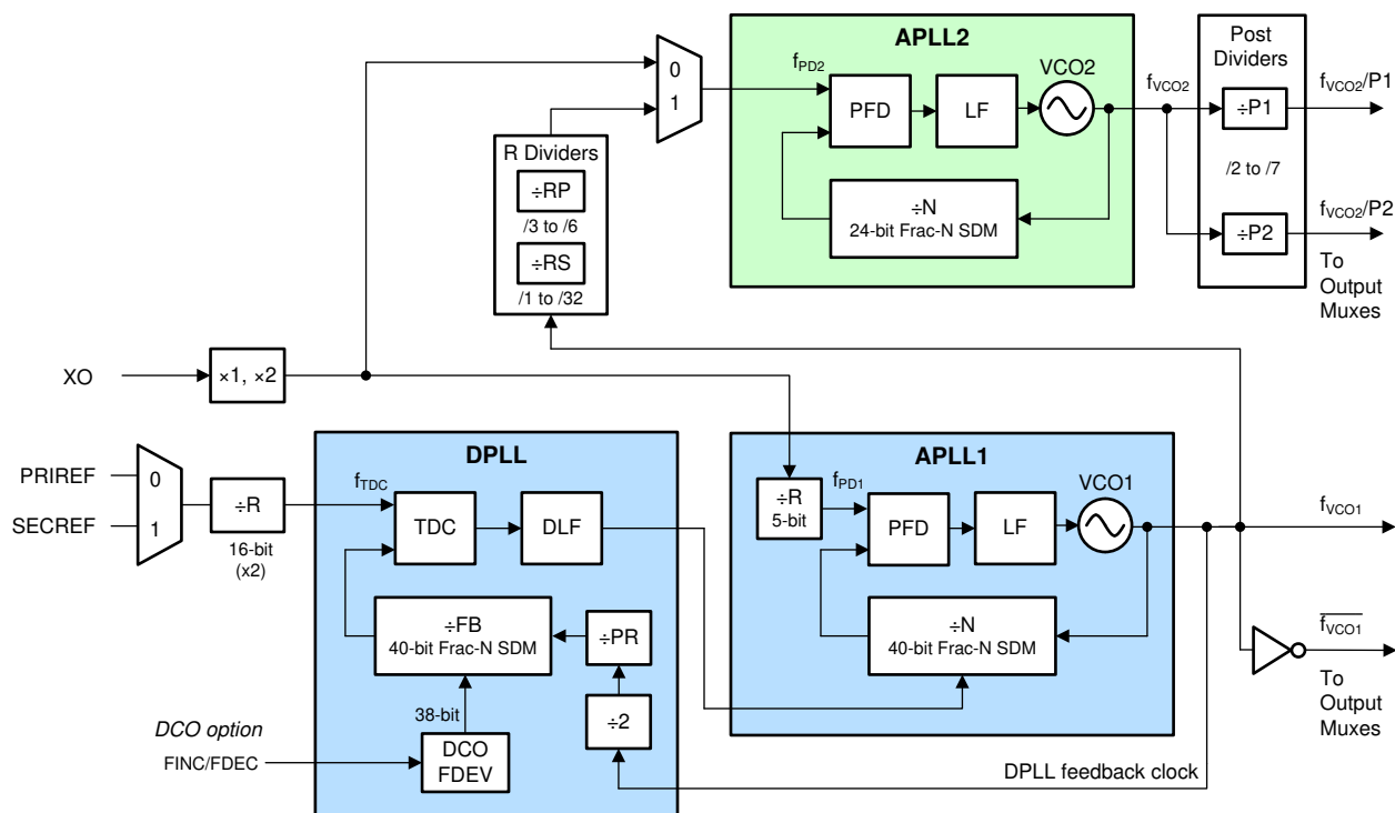
图 8-22. PLL 架构
