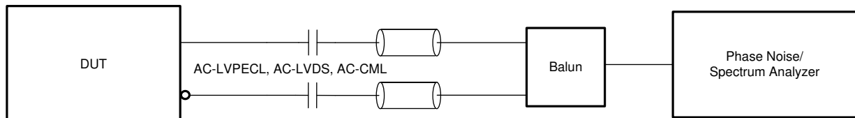
图 7-4. AC-LVPECL、AC-LVDS、AC-CML 输出相位噪声测试配置
