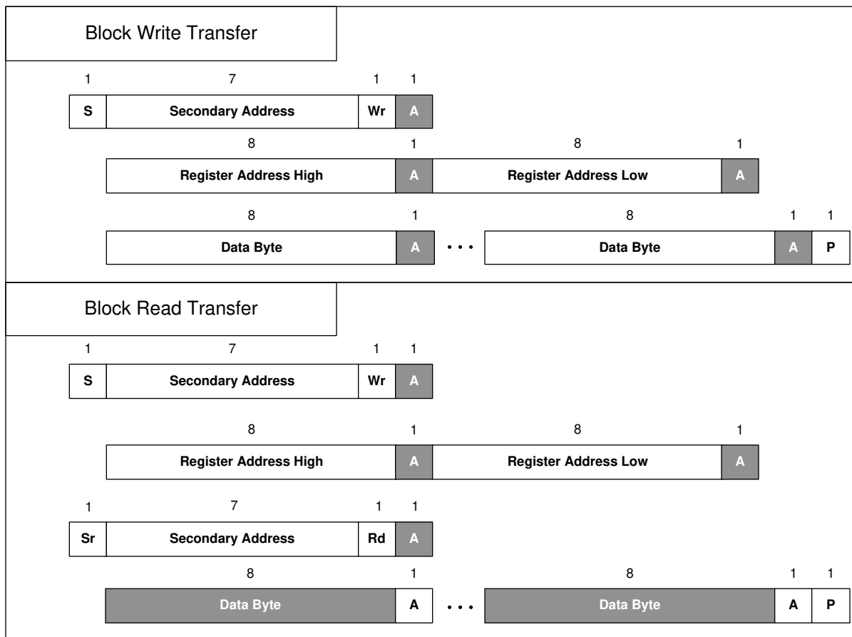
图 8-38. I 2 C 块寄存器传输
