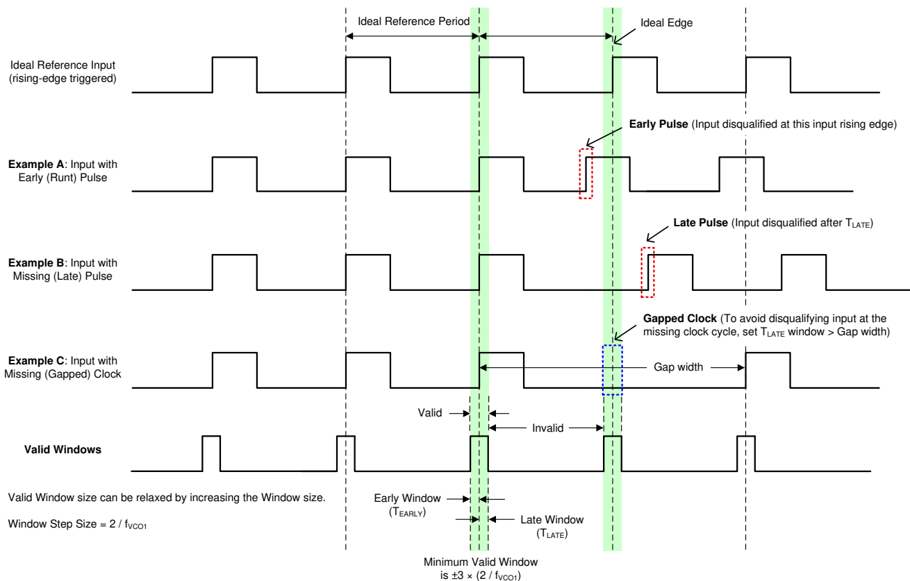
图 8-17. 早期和晚期窗口检测器示例
