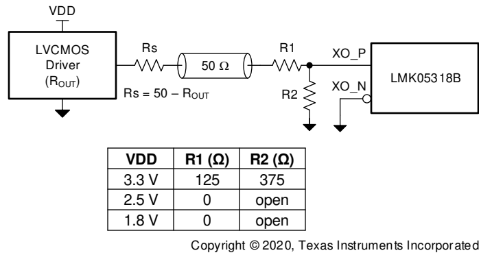
图 8-8. 单端 LVC MOS ( 1.8V、2.5V、3.3V ) 至 XO 输入 (XO_P)
