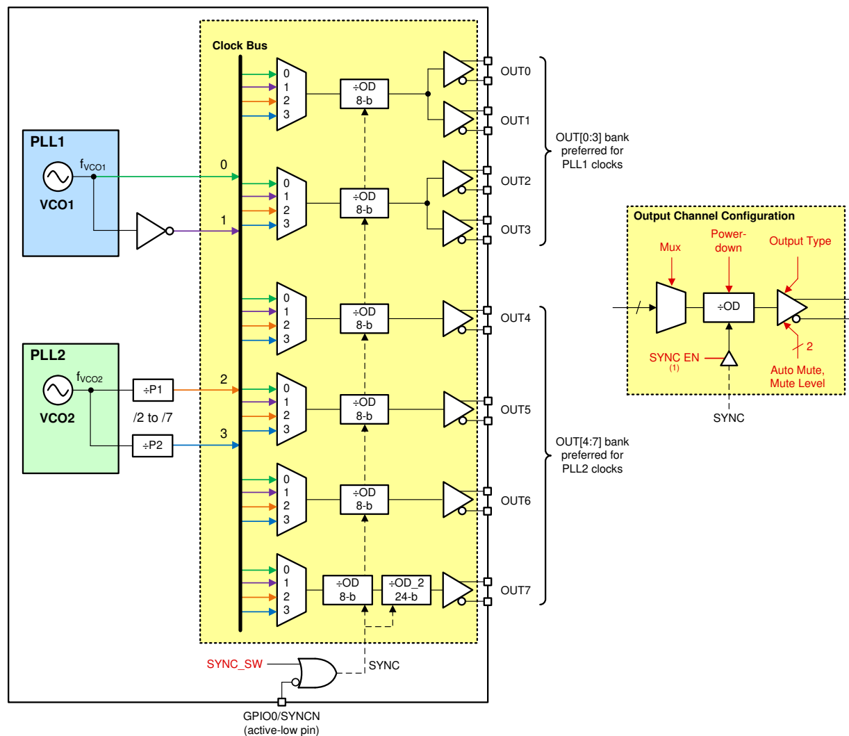
图 8-24. 输出时钟分配
