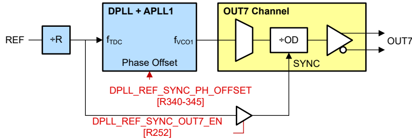
图 8-31. 1PPS PRIREF 至 OUT7 同步图
