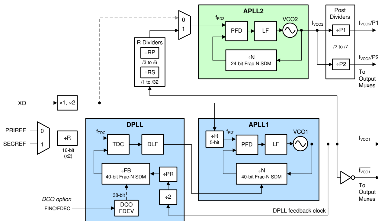
图 8-3. 具有级联 APLL2 的 DPLL 模式
