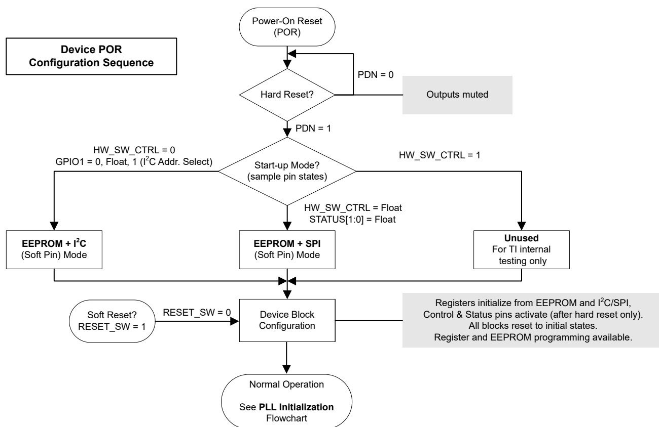
图 8-32. 器件 POR 配置序列
