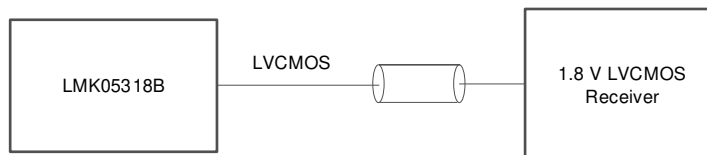
图 8-26. 1.8V LVC MOS 输出至 1.8V LVC MOS 接收器
