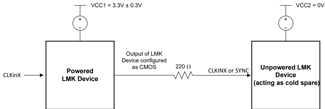
图 9-7. Cold Sparing Devices Setup
