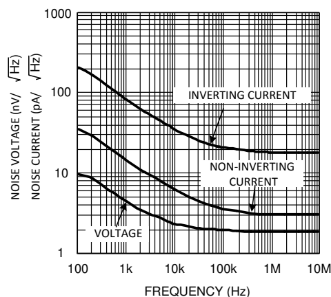
图 5-14. Noise
