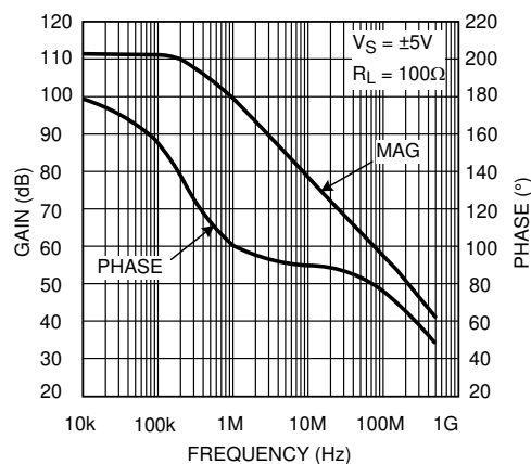
图 5-16. Transimpedance
