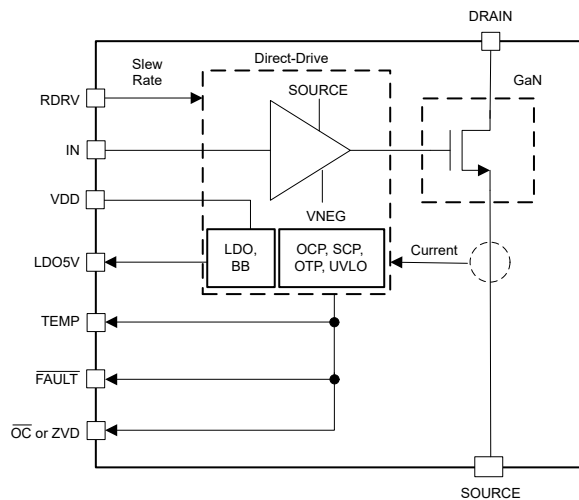
简化版方框图
