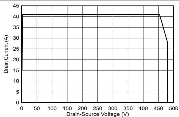
图 5-12. 最大安全工作区
