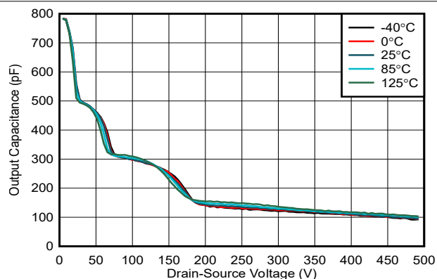
图 5-8. 输出电容与漏源电压之间的关系
