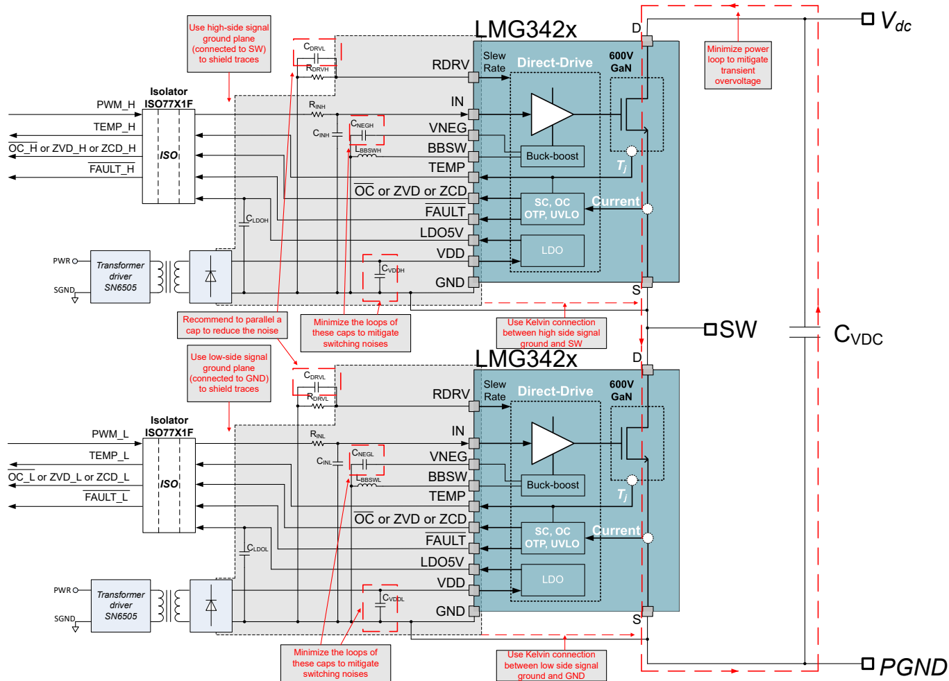
图 8-9. 典型原理图与布局注意事项
