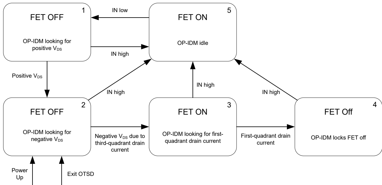
图 7-6. 可操作的理想二极管模式 (OP-IDM) 状态机
