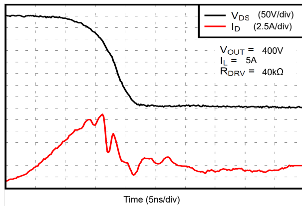
图 8-5. 应用示例中的导通波形
