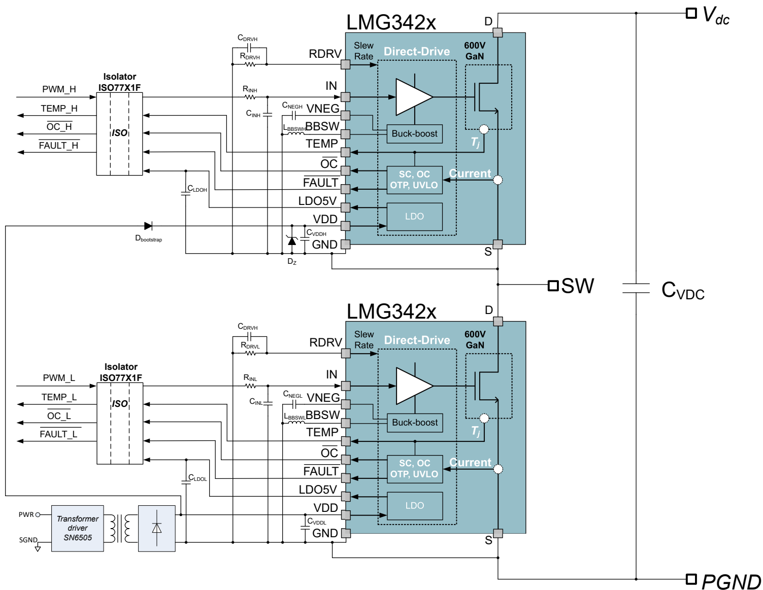
图 8-2. 具有自举功能的典型半桥应用
