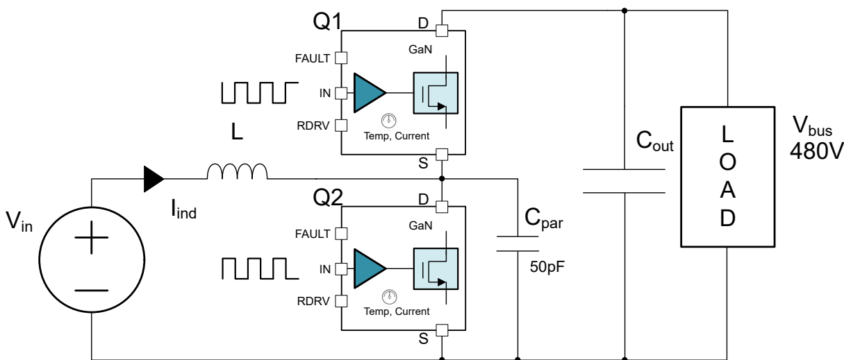
图 6-3. 安全工作区曲线所用电路
