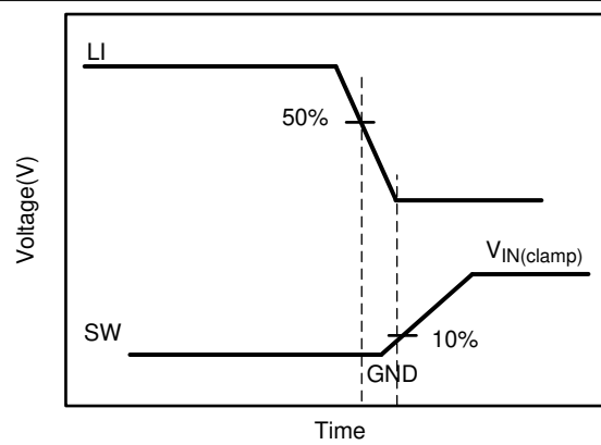
图 6-5. 低侧栅极驱动器关断
