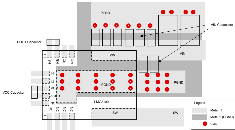
图 8-7. 外部元件放置方式 (多层 PCB)
