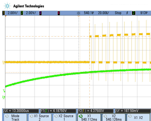
图 7-6. 启动时间
