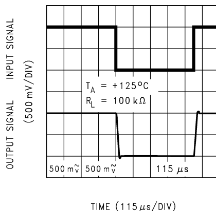
图 6-16. 同相大信号脉冲响应
