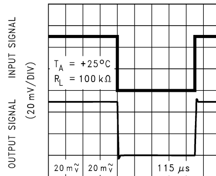
图 6-20. 同相小信号脉冲响应
