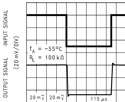
图 6-19. 同相小信号脉冲响应
