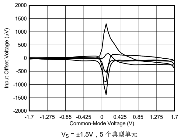
图 6-10. 输入失调电压与共模电压间的关系
