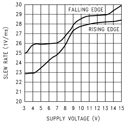
图 6-15. 压摆率与电源电压间的关系
