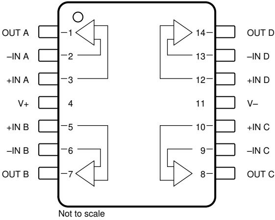
图 4-3. LMC6044 : D 封装 , 14 引脚 SOIC 和 N 封装 , 14 引脚 PDIP ( 顶视图 )
