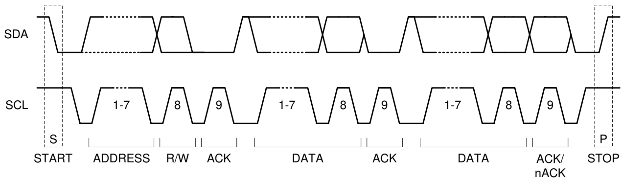
图 8-31. I 2 C 启动/停止/确认协议
