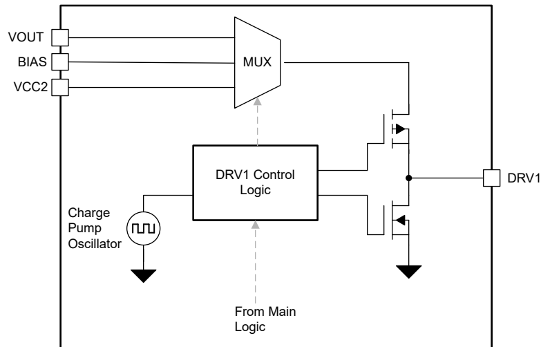
图 8-23. 功能方框图 - DRV1 引脚
