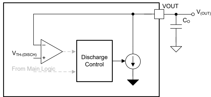
图 8-14. 功能方框图输出放电
