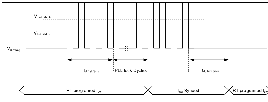
图 8-21. 时序图 SYNC 功能
