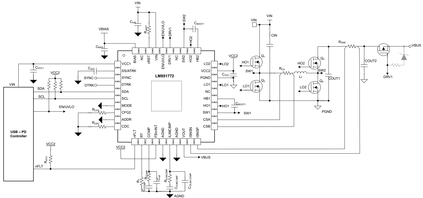
图 10-26. 具有电源路径的 USB PD 源的简化原理图
