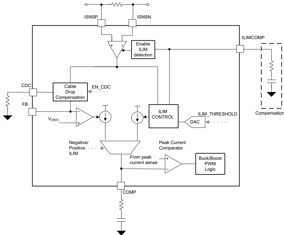
图 8-16. 电流监测功能方框图
