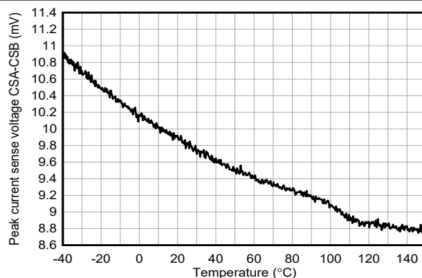
图 6-30. 平均电流限制阈值电压与温度间的关系 ILIM_THRESHOLD = 0x14
