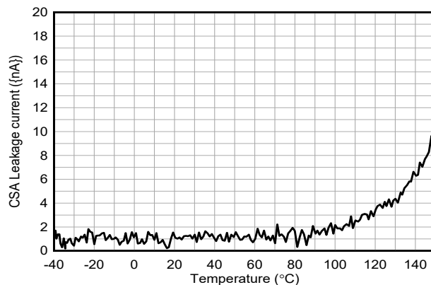
图 6-26. CSA 输入电流与温度间的关系
