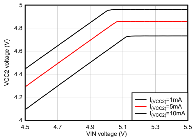
图 6-13. VCC2 LDO 输出电压与 VIN 电压间的关系 V_{(BIAS)} = 0\text{V}
