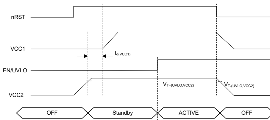
图 8-10. VCC 稳压器计时示意图 V_{BIAS} > V_{T+(Sel,BIAS)}
