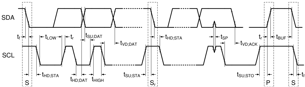
图 8-32. I 2 C 数据传输时序
