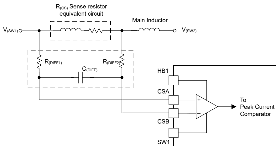
图 8-15. 峰值电流传感器的简化版原理图
