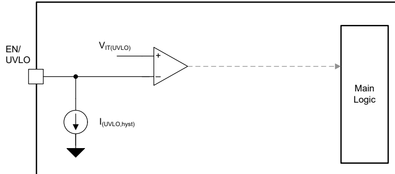
图 8-11. 功能方框图 UVLO
