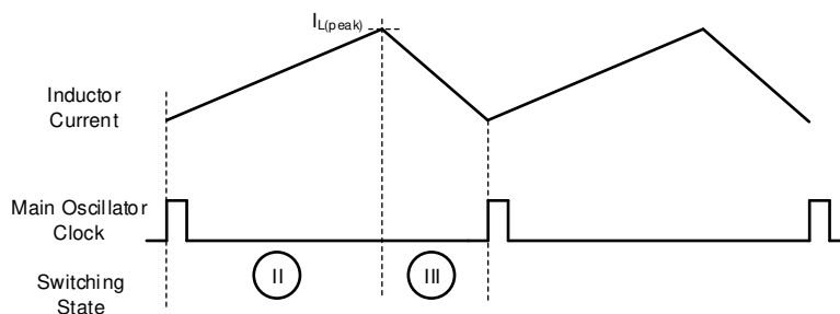
图 8-2. 连续电流降压运行模式下的电感器电流
