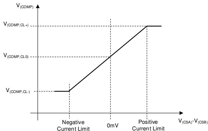
图 8-12. 峰值电流检测电压与 V_{COMP} 间关系的控制函数
