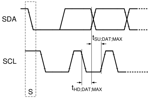
图 8-33. 最长上升和下降时间的 I 2 C 数据传输时序
