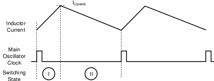
图 8-3. 连续电流升压运行模式下的电感器电流
