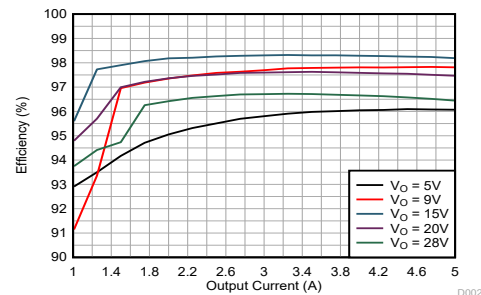
效率与输出电流的关系， V_1 = 12V ，PSM
