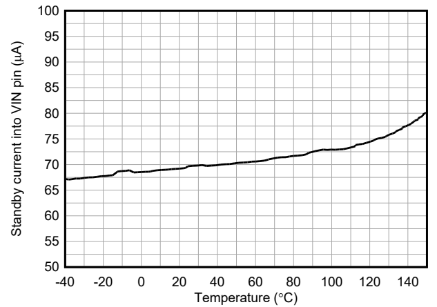
图 6-10. 流入 VIN 的待机电流与温度的关系 V_{(BIAS)} = 3.5\text{V} , V_{(VIN)} = 12\text{V}
