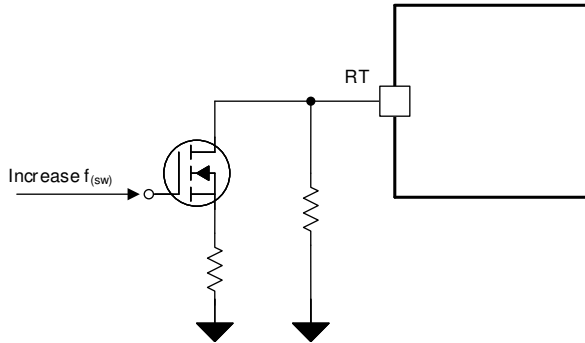
图 8-18. 跳频示例
