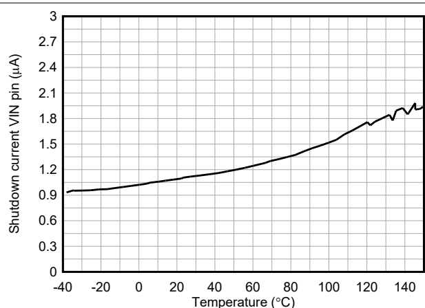
图 6-6. 流入 VIN 的关断电流与温度间的关系 V_{EN/UVLO} = 0\text{V} , V_{(VIN)} = 12\text{V} , V_{(BIAS)} = 0\text{V}
