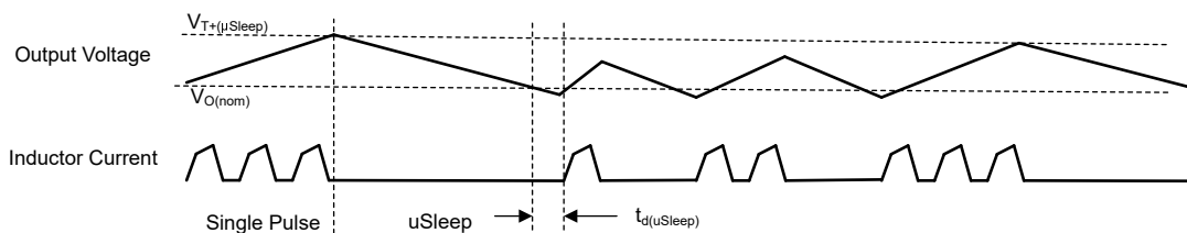
图 8-6. 省电模式的时序图 ( \mu Sleep 启用 )
