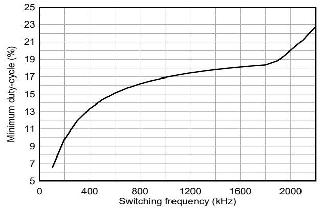
图 6-22. PSM 运行的降压最小占空比与开关频率间的关系 ( SYNC_OUT = 启用 )
