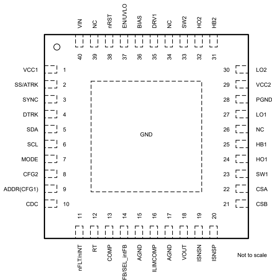
图 5-1. LM851772-Q1 RHA 封装, 40 引脚 VQFN (顶视图)
