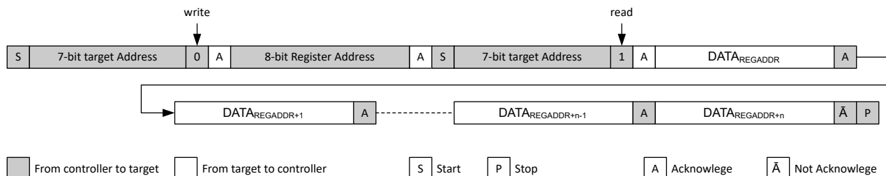
图 8-35. 从定义的寄存器地址开始进行顺序读取
