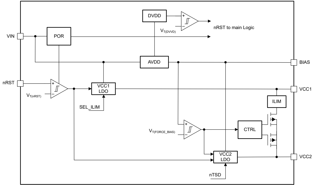
图 8-8. 参考系统功能方框图
