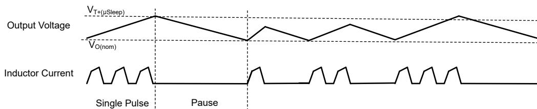
图 8-5. 省电模式的时序图 ( \mu Sleep 禁用 )
