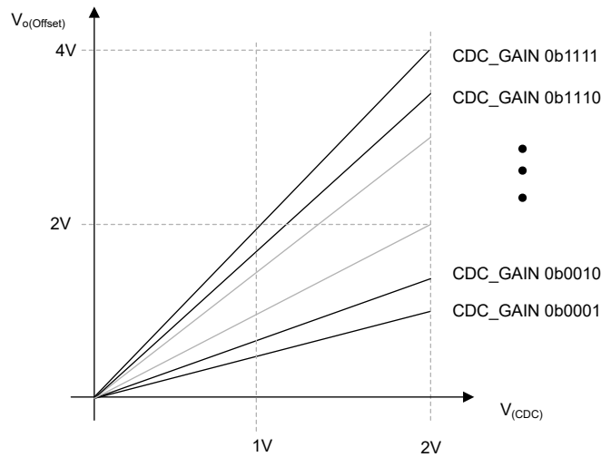
图 8-26. Vo 偏移电压与 CDC 电压的关系
