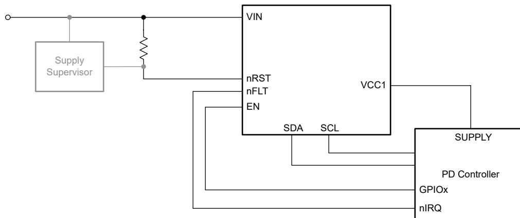
图 8-9. 简化版原理图
