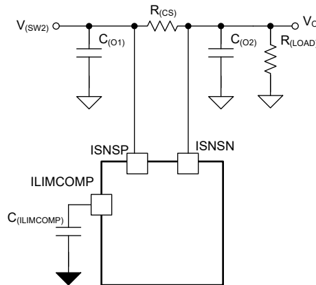
图 8-17. 具有阻性负载的电流限制元件简化版原理图
