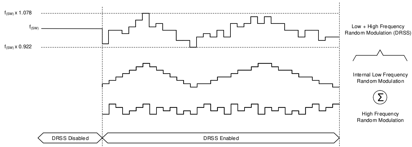
图 8-24. 双随机展频
