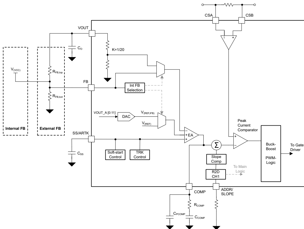
图 8-13. EA 功能方框图
