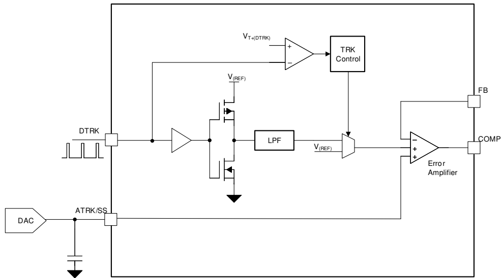
图 8-22. 输出电压跟踪功能方框图
