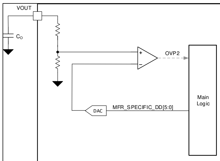
图 8-28. OVP2 功能方框图
