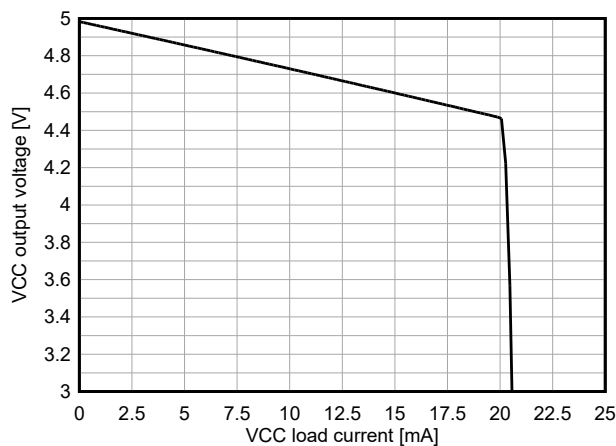
图 6-11. VCC2 LDO 输出电压与 VCC2 负载电流间的关系 V_{(VIN)} = 12\text{V} , V_{(BIAS)} = 0\text{V}
