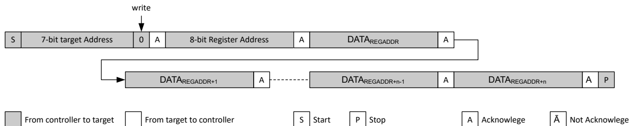
图 8-37. 在定义的寄存器地址开始进行顺序写入
