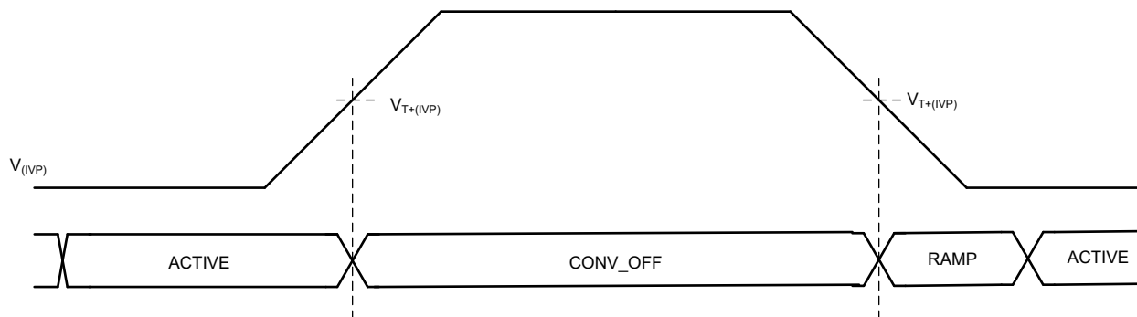
图 8-29. IVP 运行时序图
