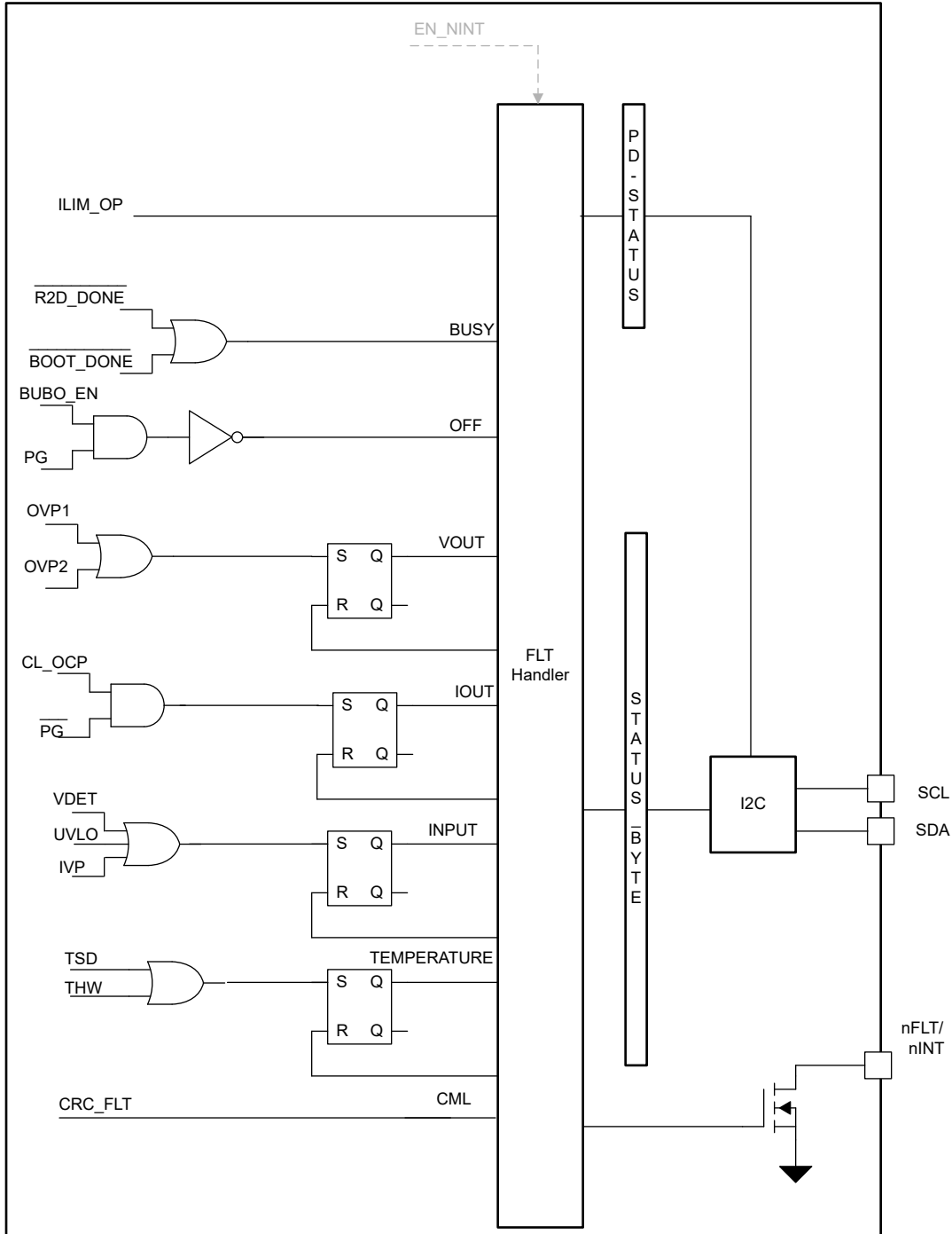
图 8-27. 功能方框图故障处理程序
