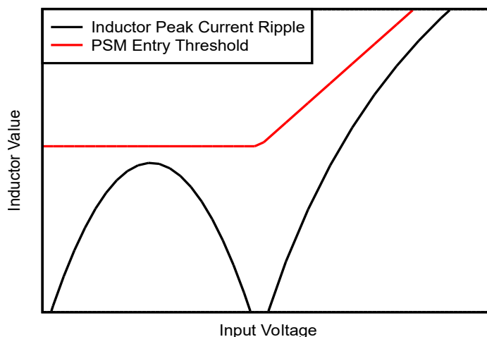
图 8-7. PSM 进入阈值与纹波电流随输入电压变化的通用曲线图
