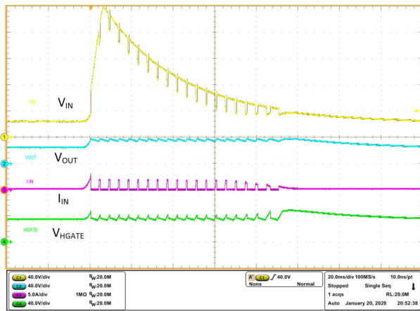
图 10-21. 未抑制的负载突降 200V - 输出钳位
