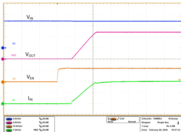
图 10-7. 负载为 60 \Omega 时的浪涌电流
