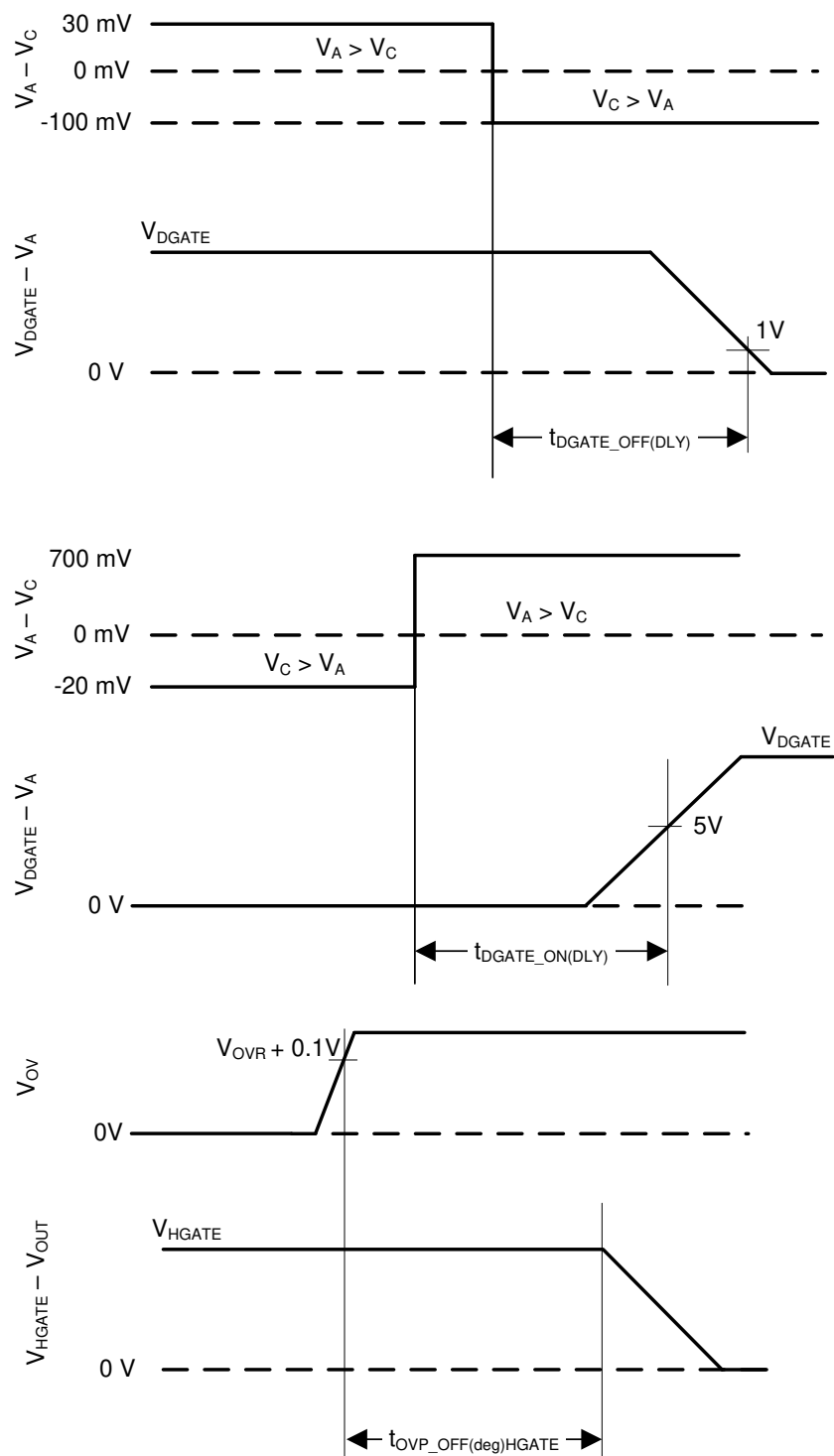
图 8-1. 时序波形
