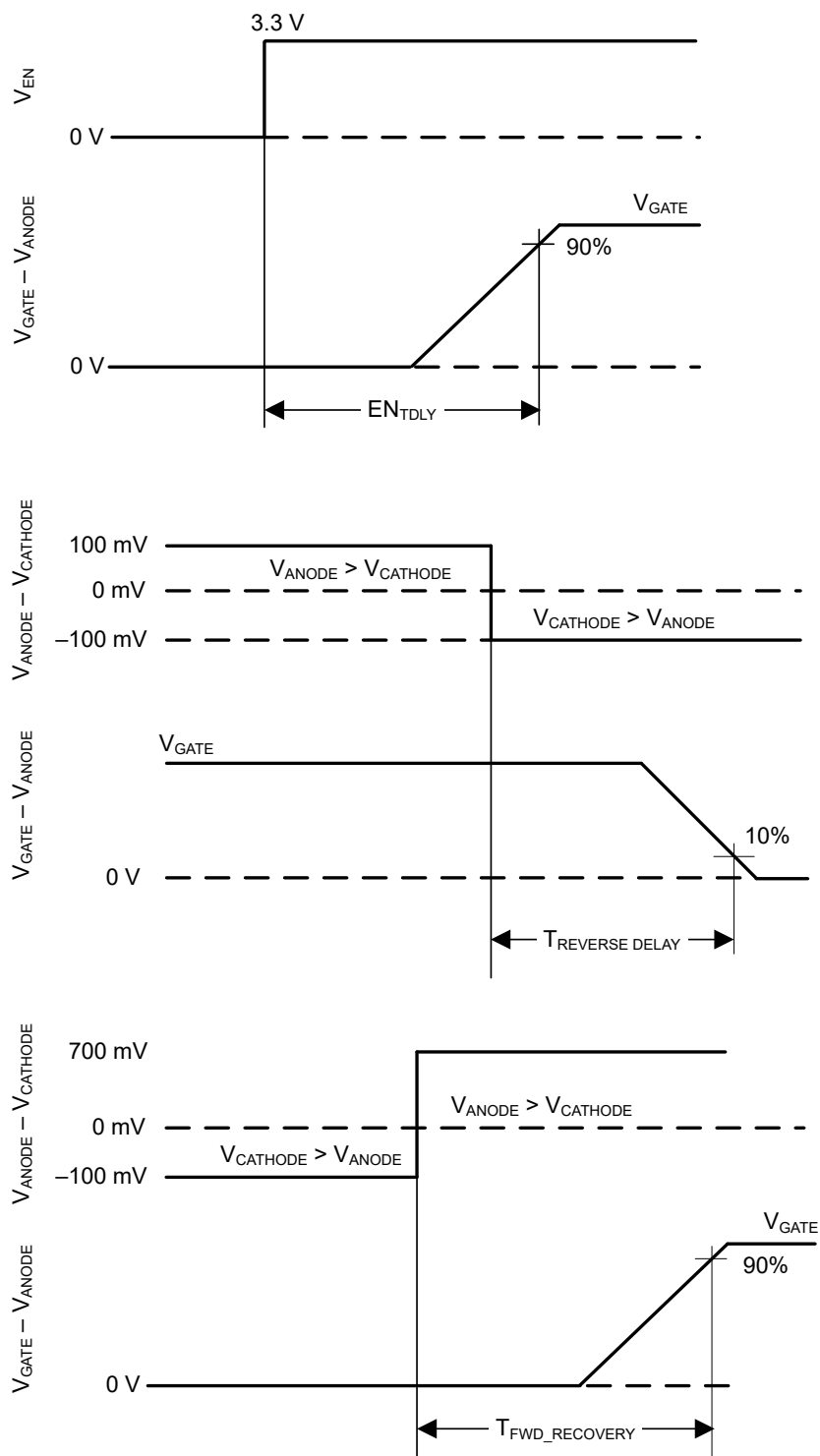
图 7-1. 时序波形
