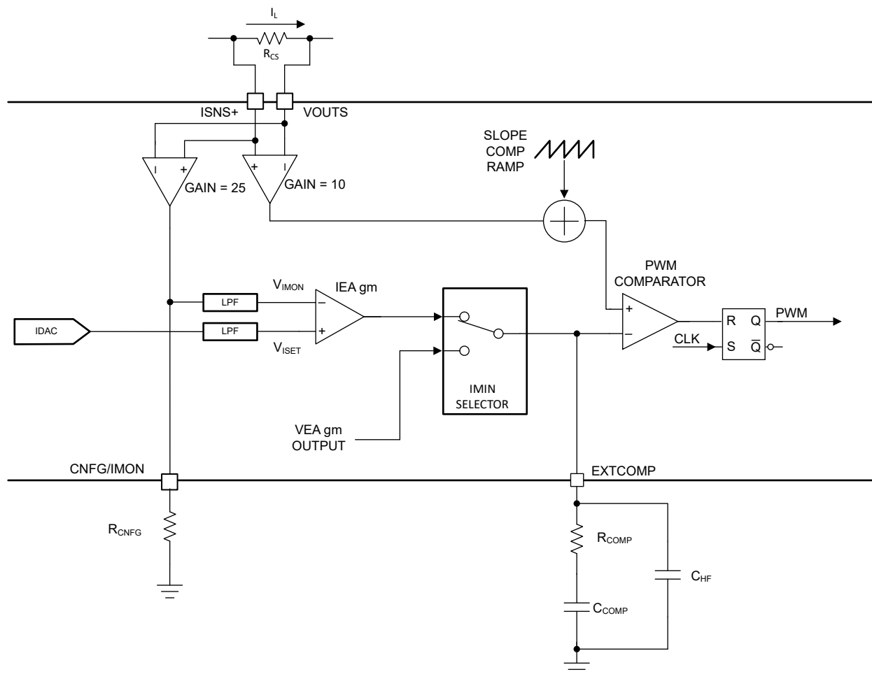
图 7-6. 电流环路功能方框图
