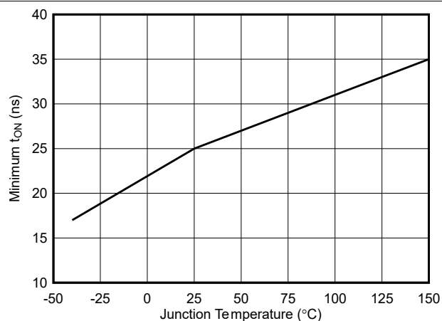
图 6-14. 最短导通时间与温度间的关系
