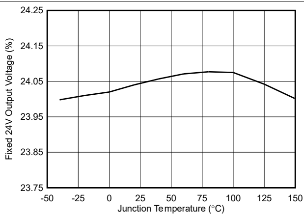
图 6-10. 固定输出电压与温度间的关系, V_{OUT} = 24\text{V}
