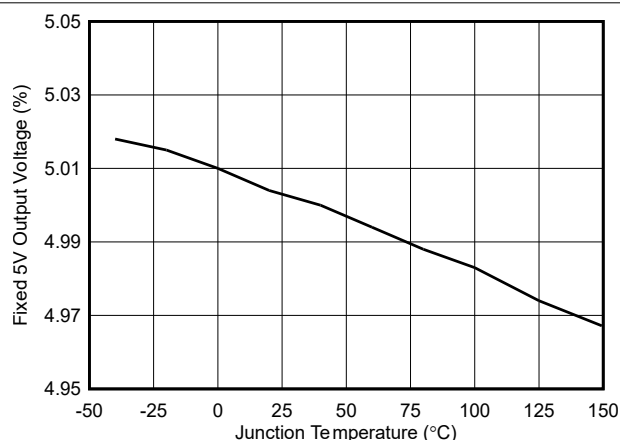
图 6-9. 固定输出电压与温度间的关系, V_{OUT} = 5\text{V}
