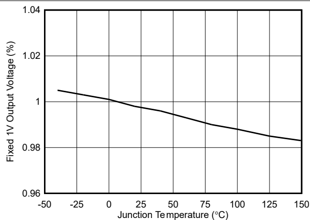
图 6-7. 固定输出电压与温度间的关系, V_{OUT} = 1\text{V}
