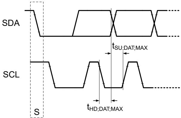
图 7-11. 最长上升和下降时间的 I 2 C 数据传输时序
