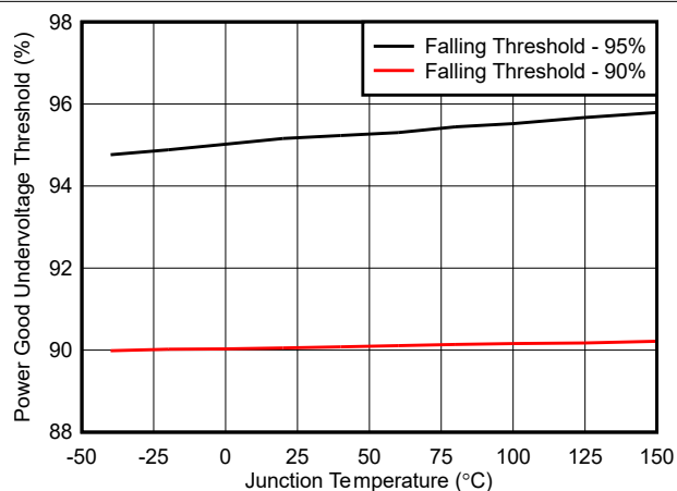
图 6-12. PG 欠压阈值与温度间的关系
