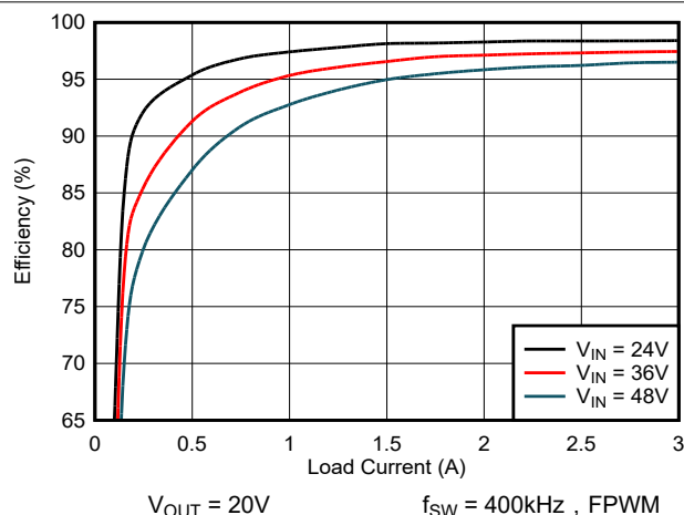
图 9-16. 效率与 I_{OUT} 之间的关系
