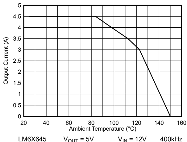
图 8-5. 热降额 - 400kHz
