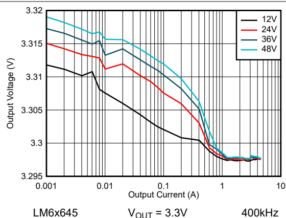
图 8-22. LM6x645 线路和负载调节 - 自动模式
