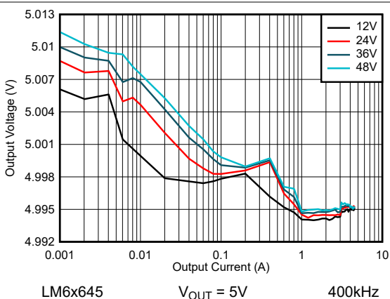
图 8-21. LM6x645 线路和负载调节 - 自动模式
