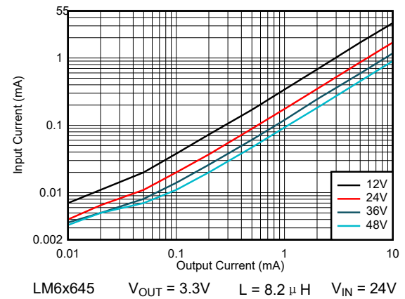
图 8-64. 输入电源电流 - 自动模式
