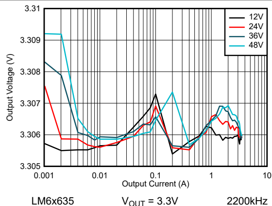
图 8-20. LM6x635 线路和负载调节 - 自动模式
