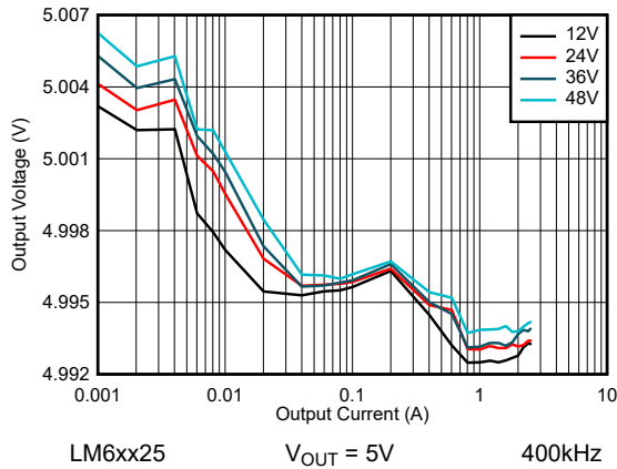
图 8-13. LM6xx25 线路和负载调节 - 自动模式
