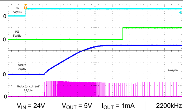
图 8-71. 启动 — 自动
