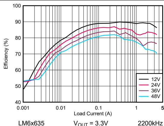
图 8-10. LM6x635 效率 - 自动模式
