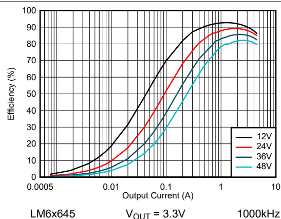
图 8-34. LM6x645 效率 - FPWM 模式
