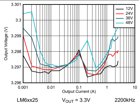
图 8-16. LM6xx25 线路和负载调节 - 自动模式
