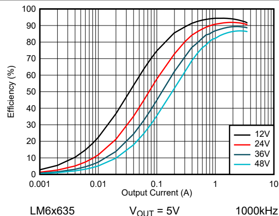
图 8-32. LM6x635 效率 - FPWM 模式
