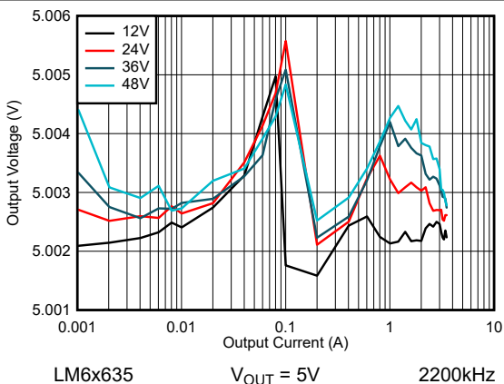
图 8-19. LM6x635 线路和负载调节 - 自动模式
