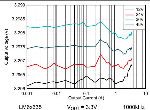
图 8-42. LM6x635 线路和负载调节 - FPWM 模式
