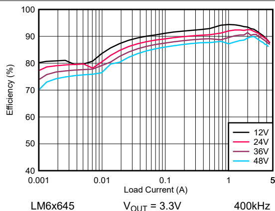
图 8-12. LM6x645 效率 - 自动模式
