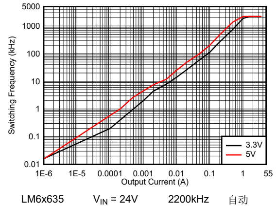
图 8-50. LM6x635 开关频率与负载电流间的关系
