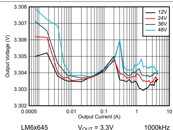
图 8-45. LM6x645 线路和负载调节 - 自动模式
