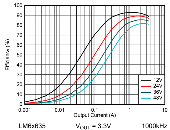
图 8-30. LM6x635 效率 - FPWM 模式
