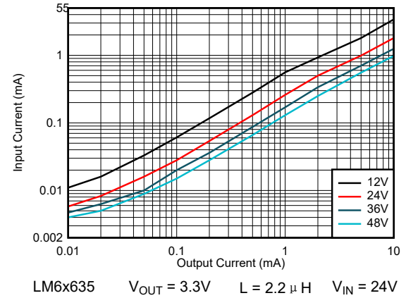
图 8-62. 输入电源电流 - 自动模式
