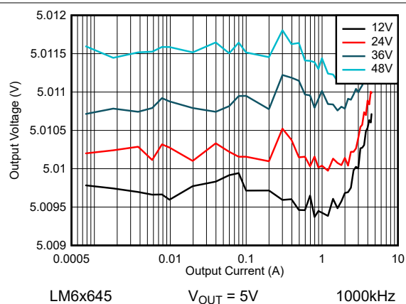
图 8-48. LM6x645 线路和负载调节 - FPWM 模式
