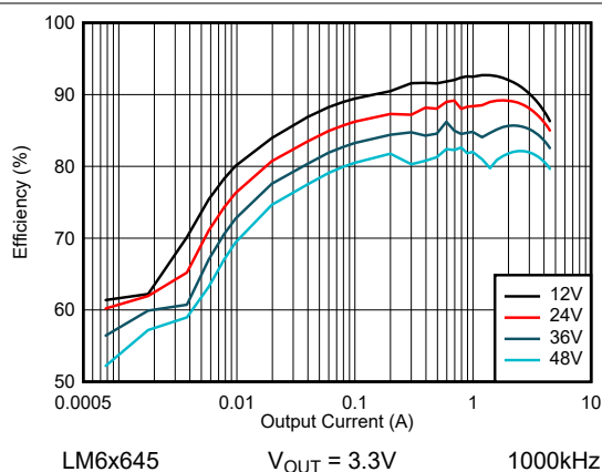
图 8-33. LM6x645 效率 - 自动模式
