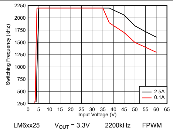
图 8-52. LM6xx25 开关频率与输入电压间的关系
