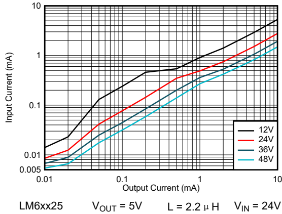
图 8-61. 输入电源电流 - 自动模式
