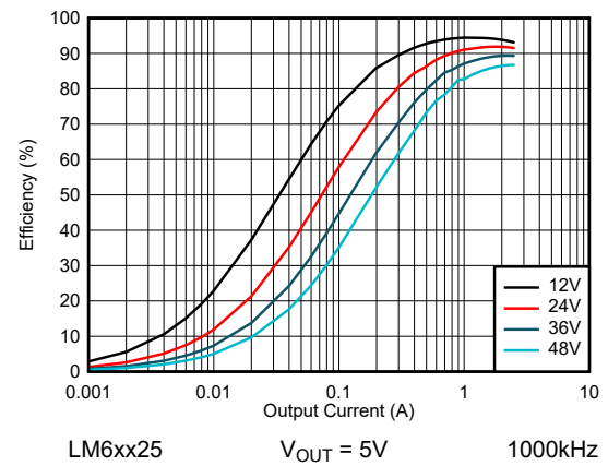
图 8-28. LM6xx25 效率 - FPWM 模式
