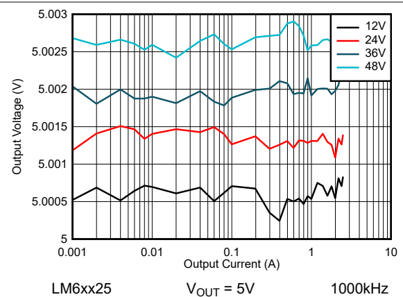
图 8-40. LM6xx25 线路和负载调节 - FPWM 模式
