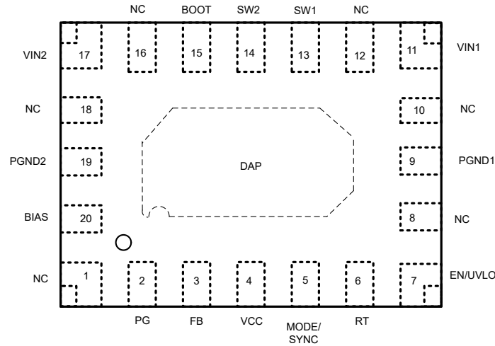
图 5-1. 20 引脚 RZT、WQFN-FCRLF 封装 (顶视图)
