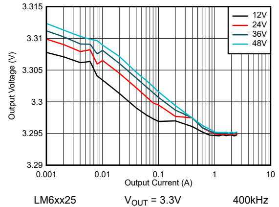
图 8-14. LM6xx25 线路和负载调节 - 自动模式
