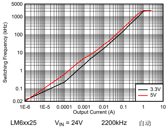
图 8-49. LM6xx25 开关频率与负载电流间的关系
