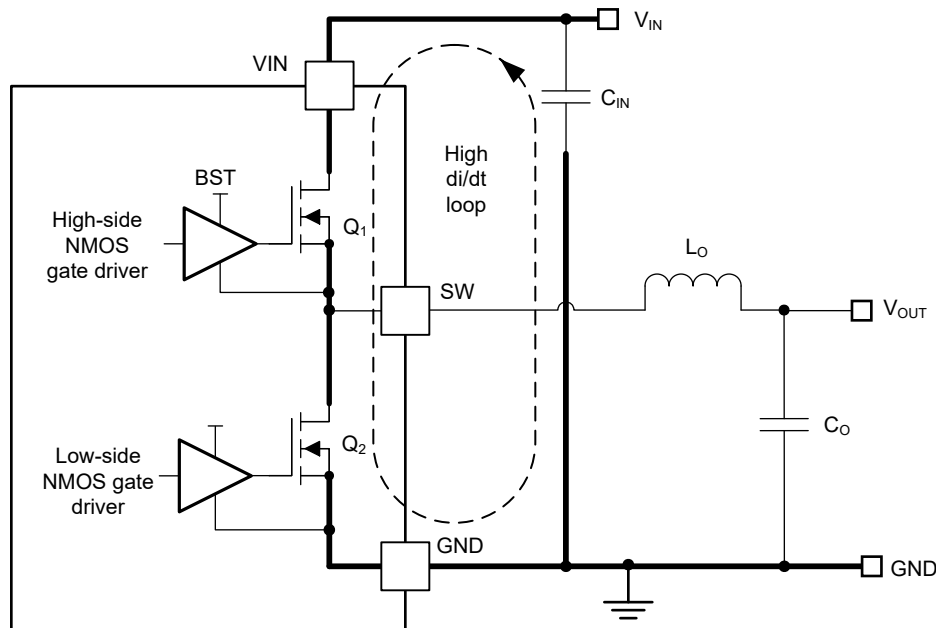
图 8-79. 具有快速边沿的电流环路
