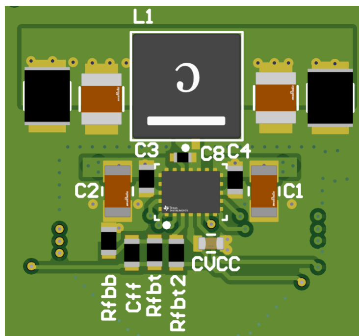
图 8-81. PCB 图像
