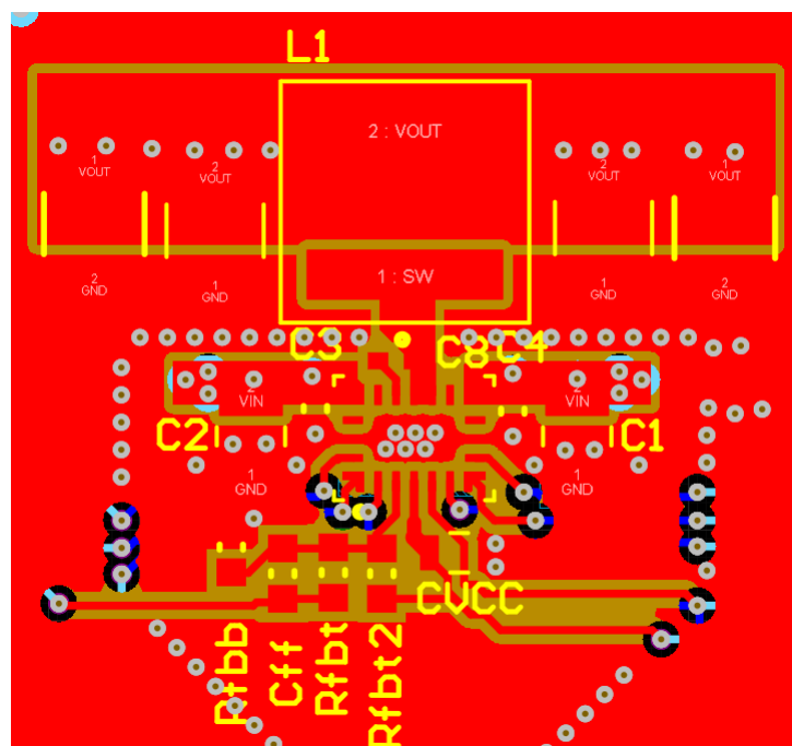
图 8-80. 布局示例
