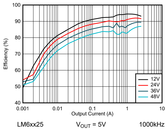
图 8-27. LM6xx25 效率 - 自动模式
