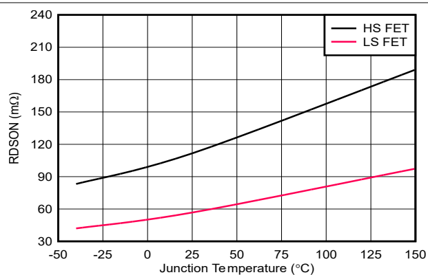
图 6-10. LS 和 HS FET RDSON
