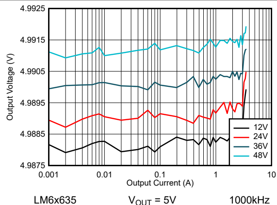
图 8-44. LM6x635 线路和负载调节 - FPWM 模式
