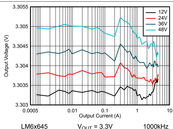
图 8-46. LM6x645 线路和负载调节 - FPWM 模式
