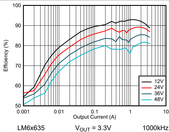
图 8-29. LM6x635 效率 - 自动模式
