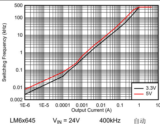
图 8-51. LM6x645 开关频率与负载电流间的关系
