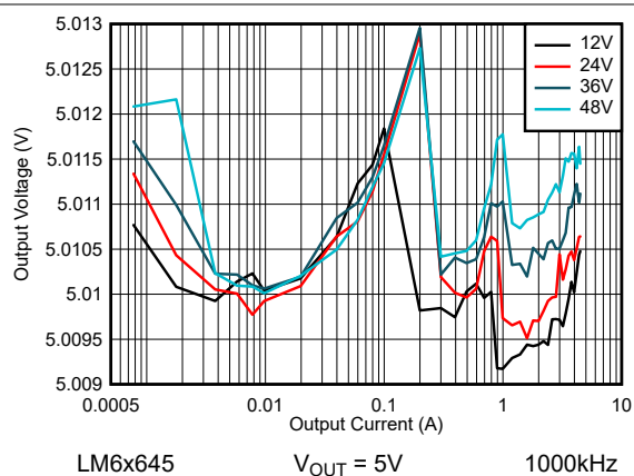
图 8-47. LM6x645 线路和负载调节 - 自动模式
