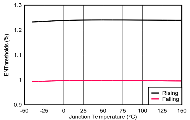
图 6-6. 启用 UVLO
