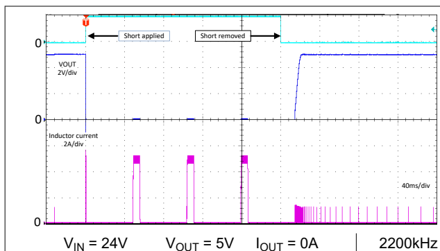
图 8-73. 输出短路电路和恢复 - 自动
