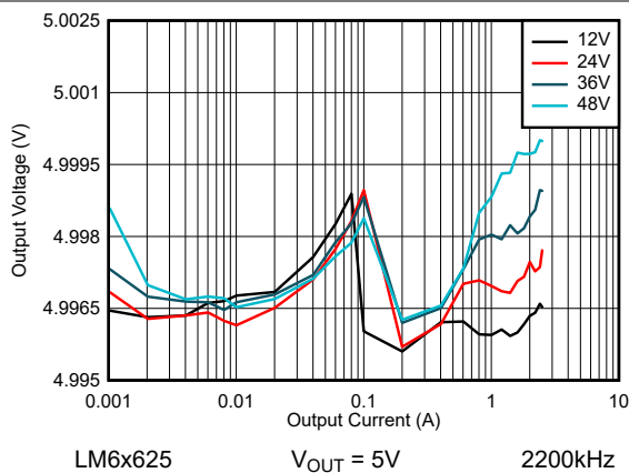
图 8-15. LM6xx25 线路和负载调节 - 自动模式
