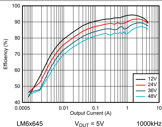
图 8-35. LM6x645 效率 - 自动模式
