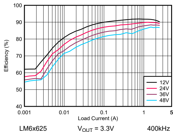
图 8-8. LM6x625 效率 - 自动模式
