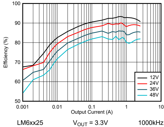
图 8-25. LM6xx25 效率 - 自动模式
