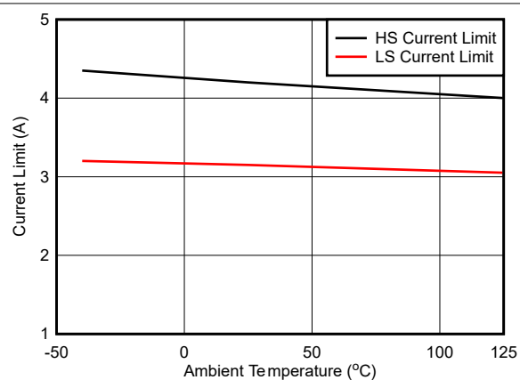
图 6-9. 2.5A 电流限制
