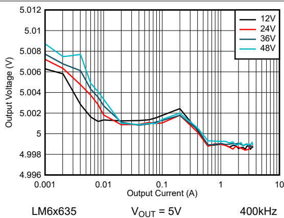
图 8-17. LM6x635 线路和负载调节 - 自动模式
