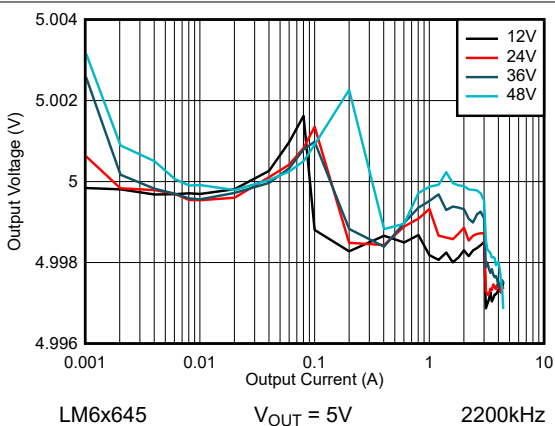
图 8-23. LM6x645 线路和负载调节 - 自动模式
