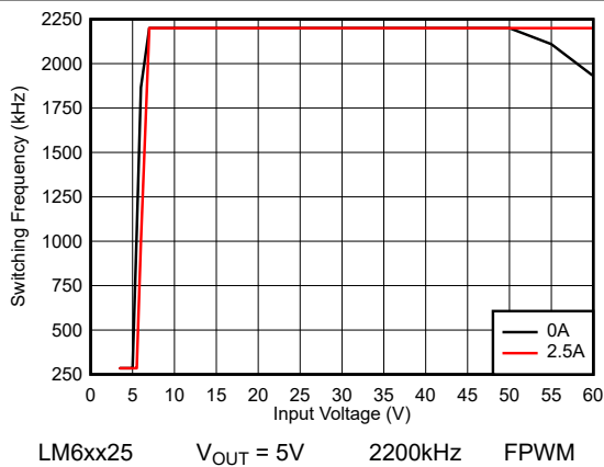
图 8-53. LM6xx25 开关频率与输入电压间的关系
