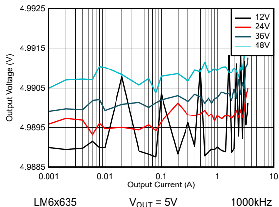
图 8-43. LM6x635 线路和负载调节 - 自动模式
