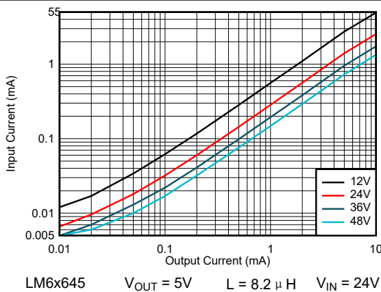
图 8-65. 输入电源电流 - 自动模式
