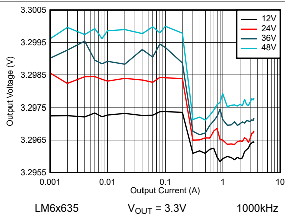
图 8-41. LM6x635 线路和负载调节 - 自动模式
