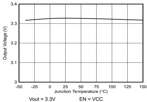
图 6-5. 固定 3.3V 输出
