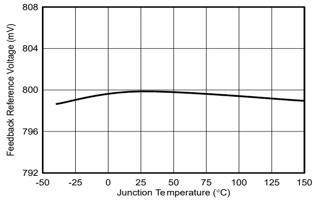
图 6-1. 反馈电压
