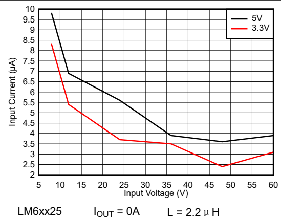
图 8-66. 空载输入电源电流 - 自动模式
