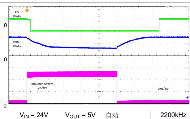
图 8-74. 电流限值瞬态
