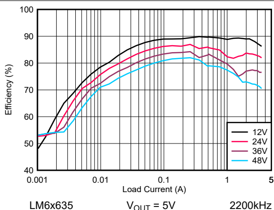
图 8-9. LM6x635 效率 - 自动模式
