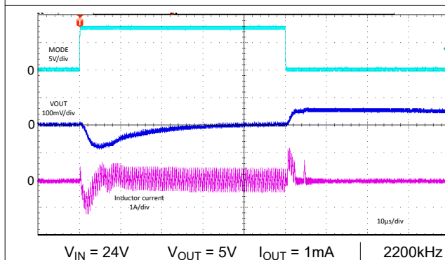
图 8-75. 模式变化瞬态
