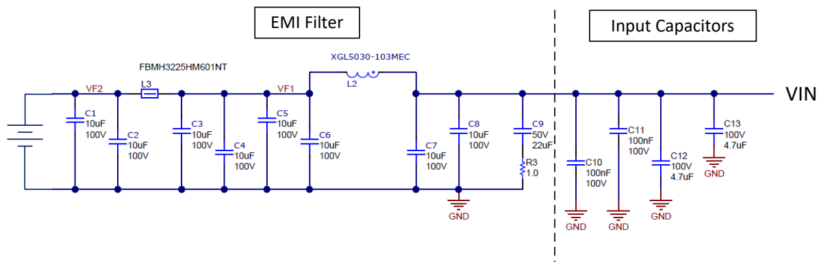
图 8-78. 适用于 400kHz 的 EMI 输入滤波器
