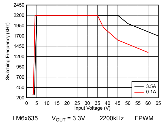
图 8-54. LM6x635 开关频率与输入电压间的关系
