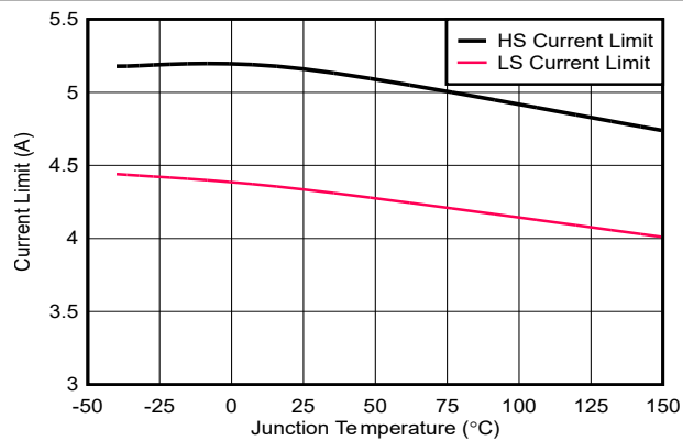
图 6-8. 3.5A 电流限制
