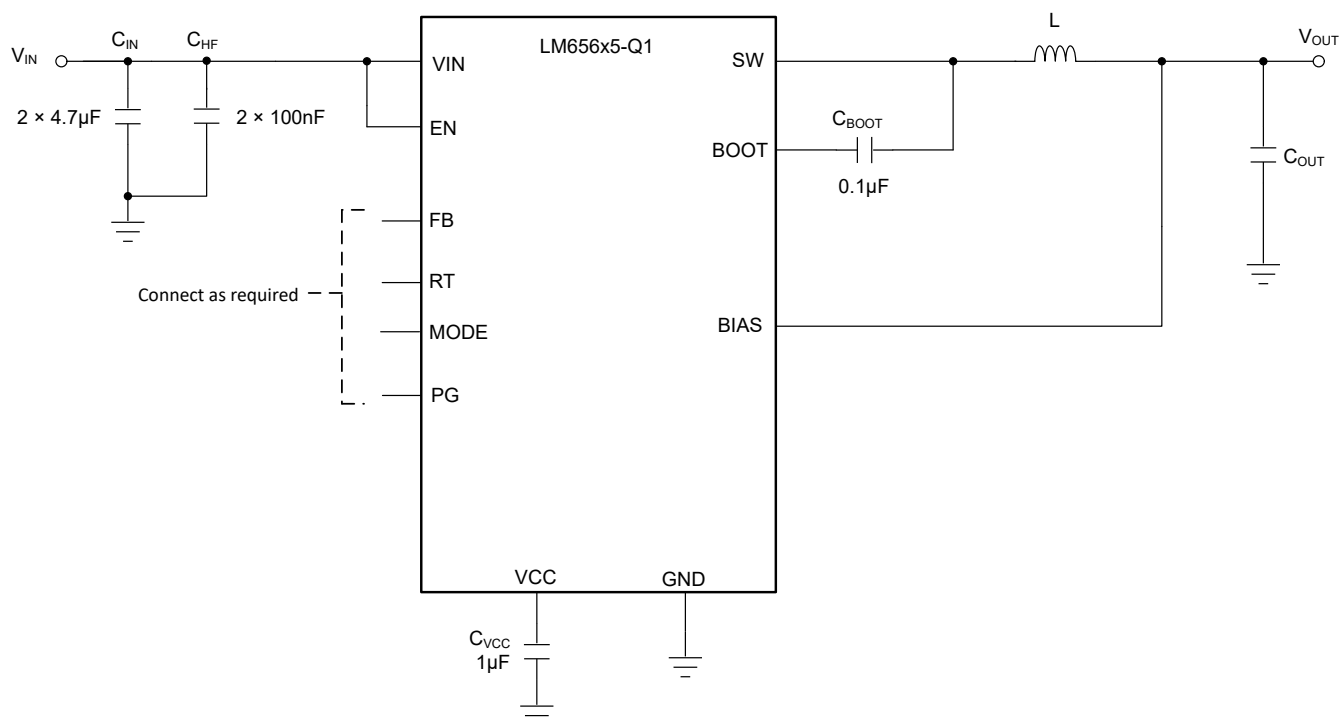
图 8-2. 采用 LM656x5 的固定输出电压模式示例应用电路
