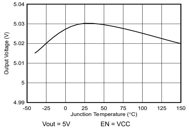
图 6-4. 固定 5V 输出
