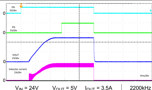
图 8-72. 启动/关断 — FPWM
