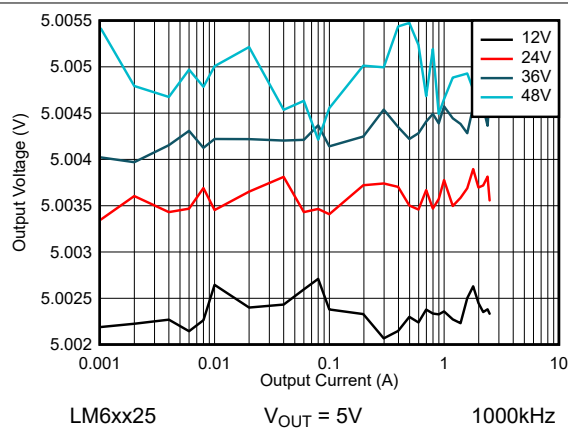
图 8-39. LM6xx25 线路和负载调节 - 自动模式
