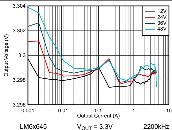
图 8-24. LM6x645 线路和负载调节 - 自动模式
