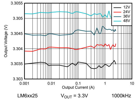
图 8-38. LM6xx25 线路和负载调节 - FPWM 模式
