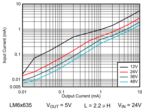
图 8-63. 输入电源电流 - 自动模式
