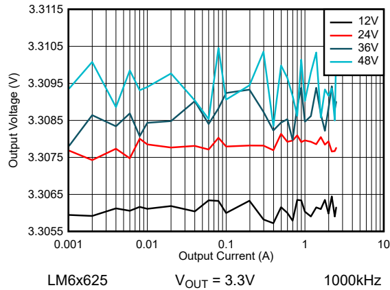
图 8-37. LM6x625 线路和负载调节 - 自动模式
