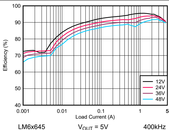
图 8-11. LM6x645 效率 - 自动模式
