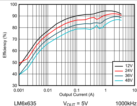
图 8-31. LM6x635 效率 - 自动模式
