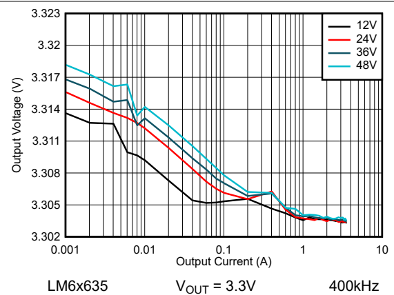
图 8-18. LM6x635 线路和负载调节 - 自动模式
