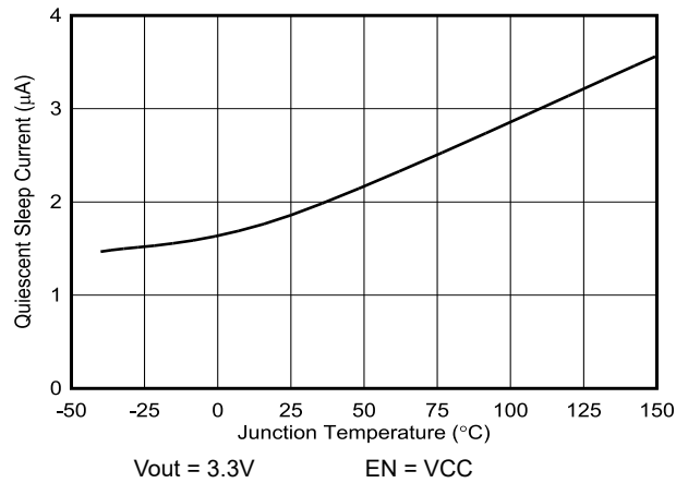
图 6-3. 睡眠静态电流 3.3V 输出
