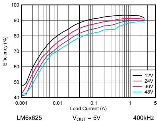
图 8-7. LM6x625 效率 - 自动模式
