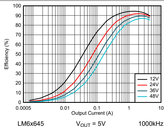
图 8-36. LM6x645 效率 - FPWM 模式
