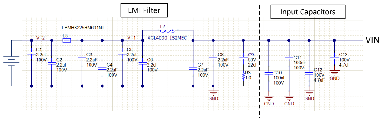
图 8-77. 适用于 2200kHz 的 EMI 输入滤波器
