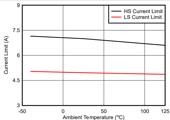
图 6-7. 4.5A 电流限制
