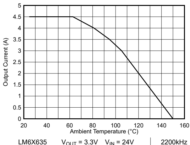
图 8-6. 热降额 - 2200kHz
