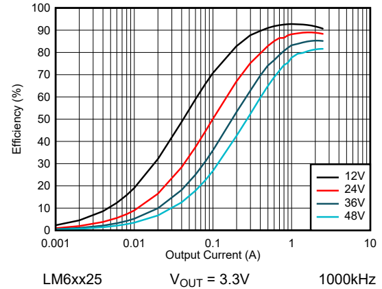
图 8-26. LM6xx25 效率 - FPWM 模式
