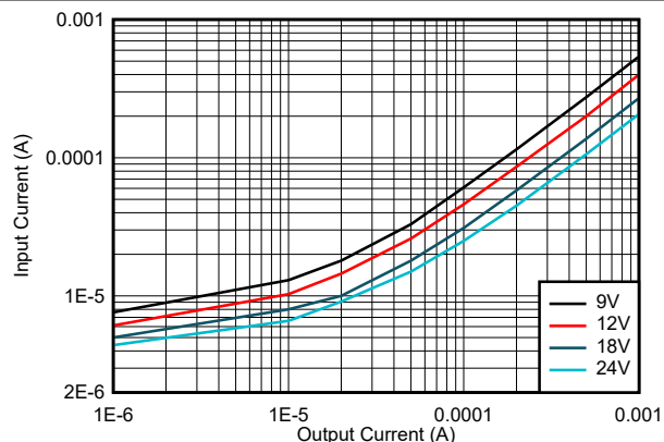
图 8-13. 输入电流
