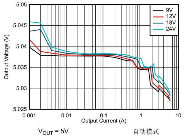
图 8-11. 线路和负载调节 - 2100kHz
