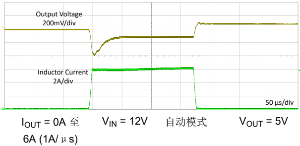
图 8-25. 负载瞬态 (AUTO)
