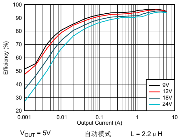
图 8-8. 效率- 2100kHz
