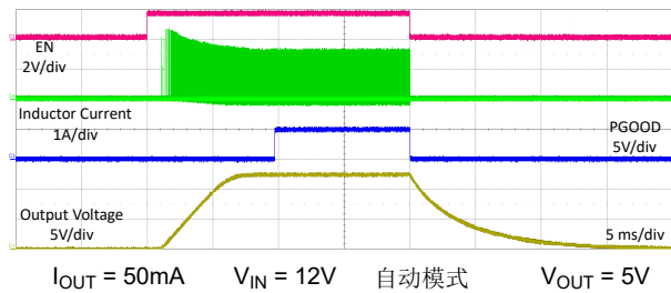
图 8-26. 启动
