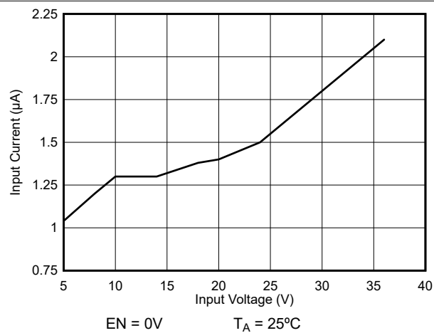
图 6-1. 关断电流
