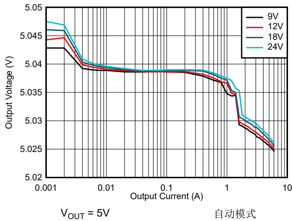
图 8-10. 线路和负载调节 - 1000kHz
