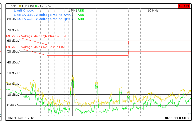
图 8-19. 传导 EMI - 400kHz
