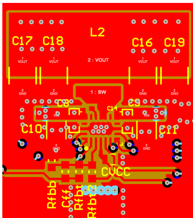
图 8-31. 布局示例
