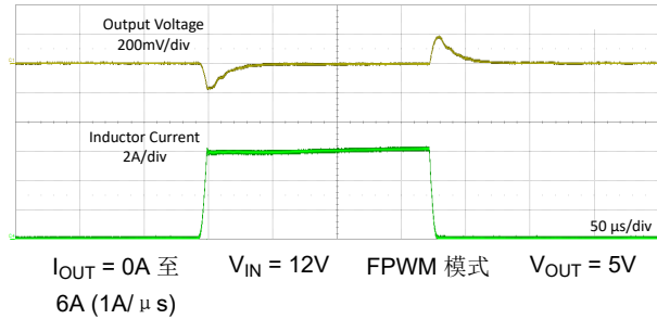
图 8-24. 负载瞬态 (FPWM)
