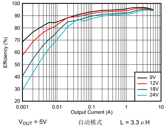
图 8-6. 效率- 400kHz
