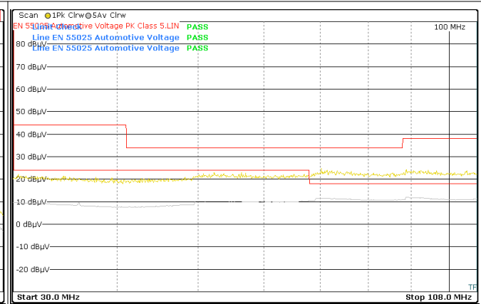
图 8-19. 传导 EMI - 400kHz
