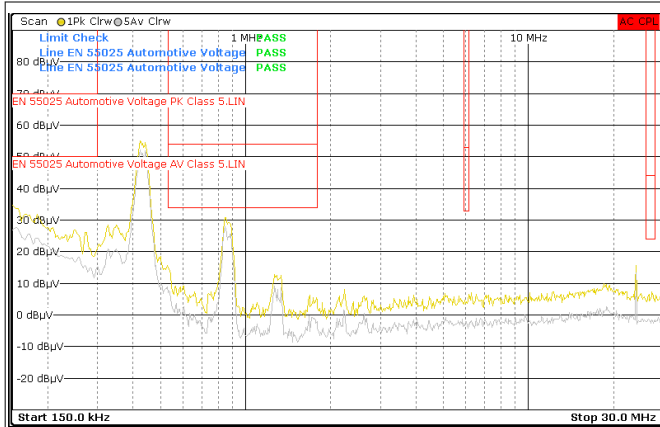
图 8-18. 传导 EMI - 400kHz
