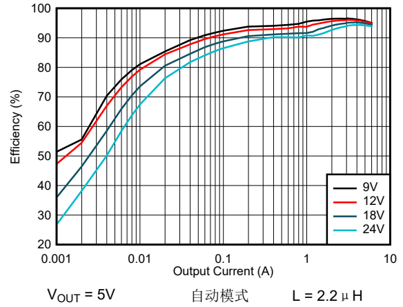
图 8-7. 效率- 1000kHz
