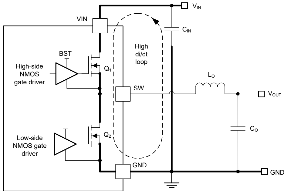
图 8-30. 具有快速边沿的电流环路
