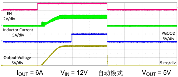
图 8-27. 启动
