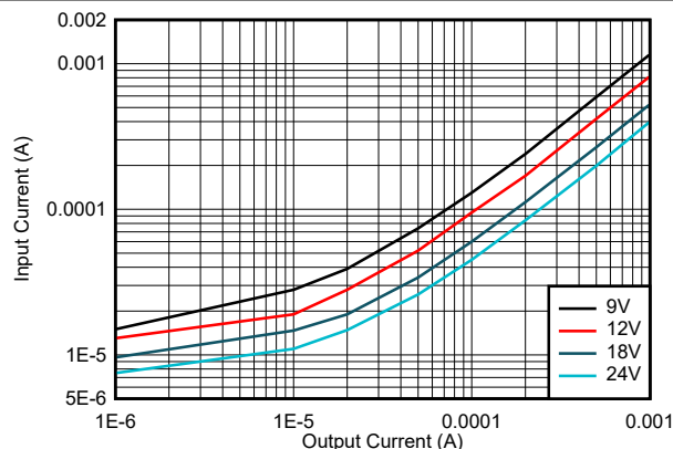
图 8-12. 输入电流
