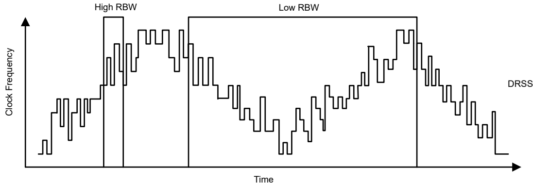
图 7-8. 双随机展频实现
