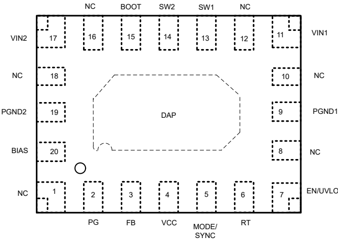
图 5-1. 20 引脚 RZT、WQFN-FCRLF 单相封装 ( 顶视图 )
