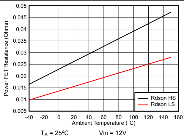
图 6-2. 功率 MOSFET 电阻
