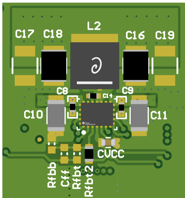
图 8-32. PCB 图像
