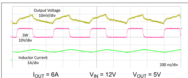
图 8-22. PWM 中的典型开关波形
