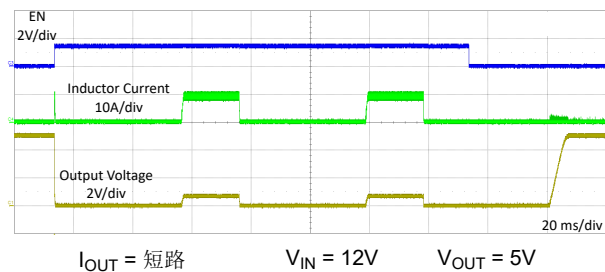
图 8-28. 短路
