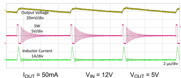
图 8-23. PFM 中的典型开关波形
