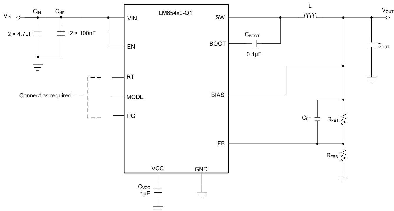
图 8-1. LM654x0-Q1 可调输出电压模式下的示例应用电路
