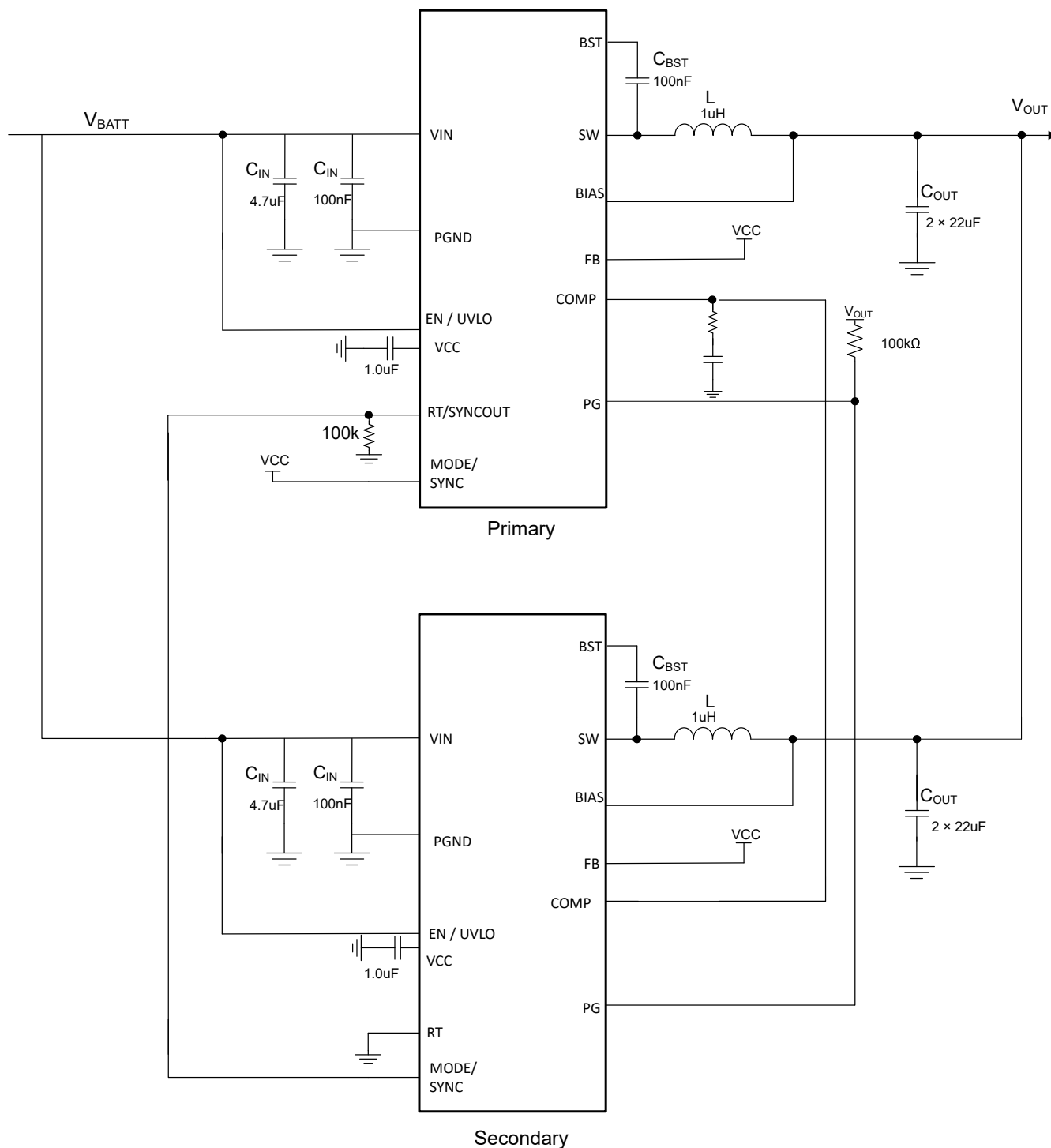
图 7-7. 典型固定 5V Vout 2100kHz 双相原理图
