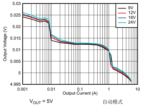
图 8-9. 线路和负载调节 - 400kHz
