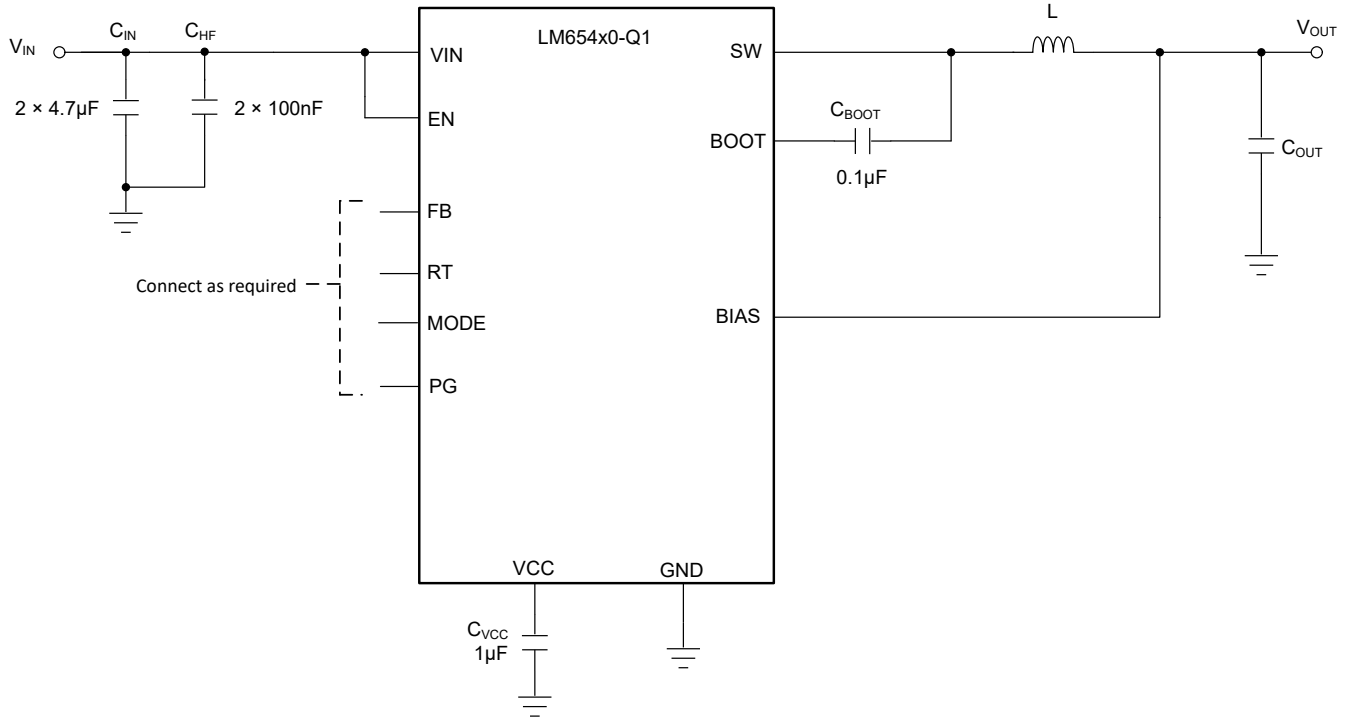
图 8-2. 采用 LM654X0-Q1 的固定输出电压模式示例应用电路
