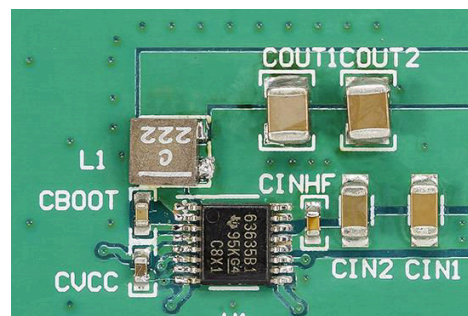
典型设计示例， I_{OUT} = 2.5A ， f_{SW} = 2200kHz
