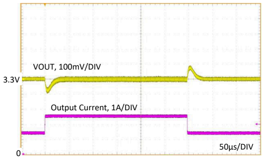
LM63625 V_{OUT} = 3.3V f_{SW} = 2100kHz 1.5A 至 2.5A, 2µs 自动
