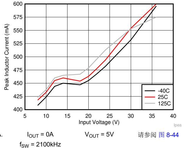
图 6-4. LM63615 的 I_{PEAK-MIN}
