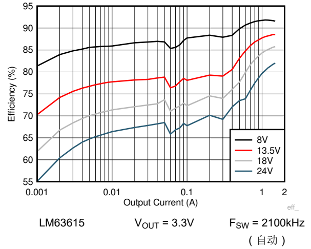
图 8-15. 效率
