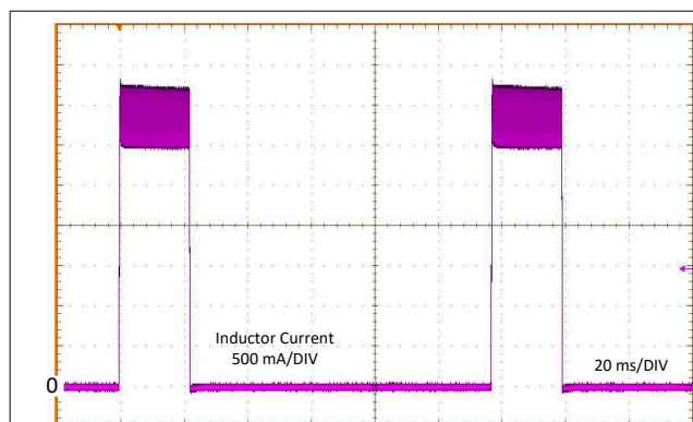
图 7-12. 短路模式下的电感器电流突发；LM63625
