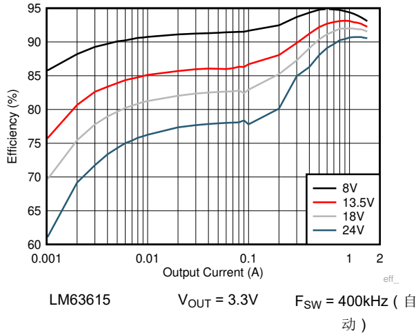
图 8-14. 效率
