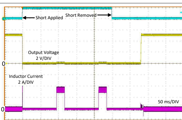
图 7-13. 短路瞬态和恢复；LM63625
