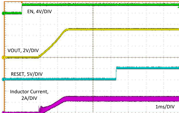
图 7-2. 精密使能行为
