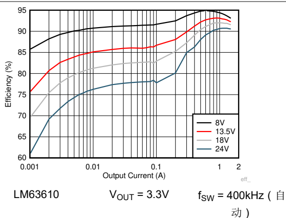
图 8-7. 效率
