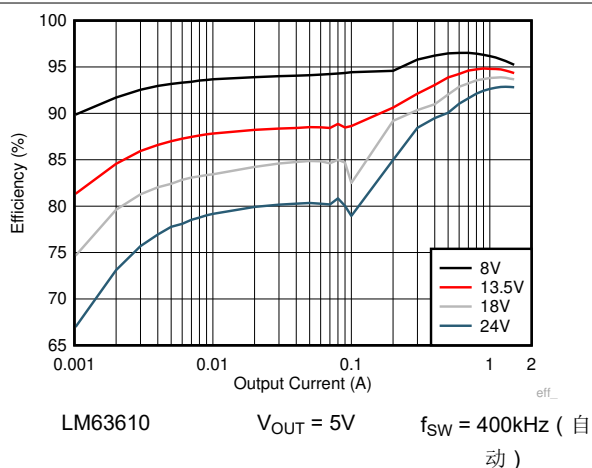
图 8-5. 效率
