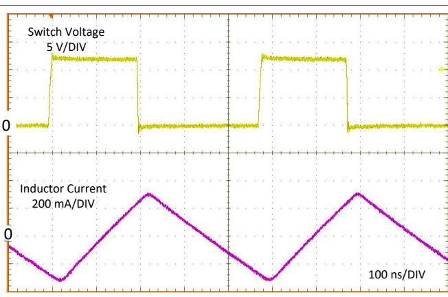
图 7-6. 典型 PWM 开关波形 FPWM ， V_{IN} = 12V ， V_{OUT} = 5V ， I_{OUT} = 0A ， f_{sw} = 2100kHz
