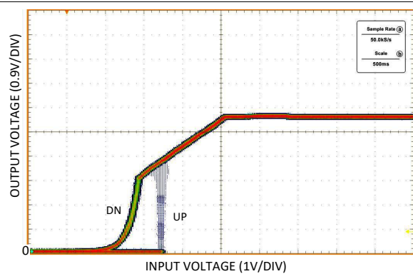
图 6-2. UVLO 阈值
