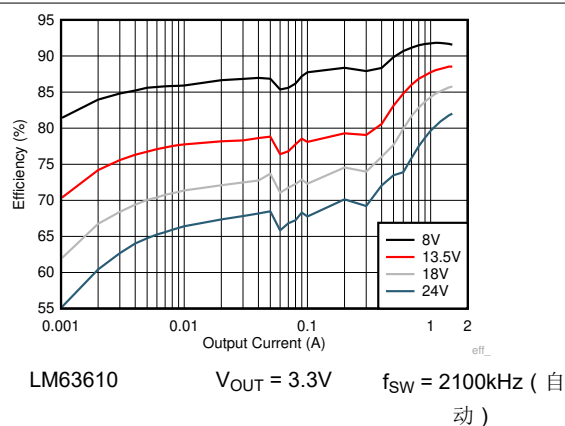
图 8-8. 效率
