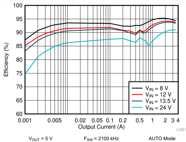
图 9-7. LM62435-Q1 Efficiency
