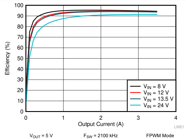
图 9-8. LM62435-Q1 Efficiency
