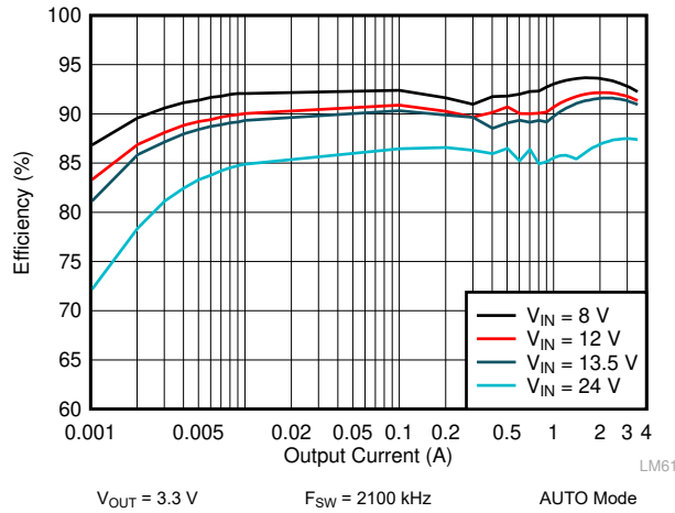
图 9-5. LM62435-Q1 Efficiency
