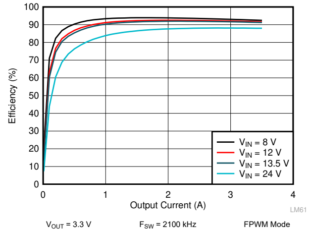
图 9-6. LM62435-Q1 Efficiency
