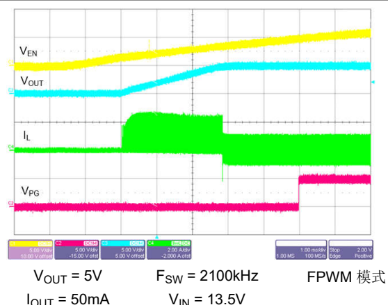
图 8-32. 在 50mA 负载下启动
