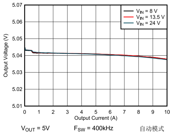
图 8-13. 负载调整率和线性调整率
