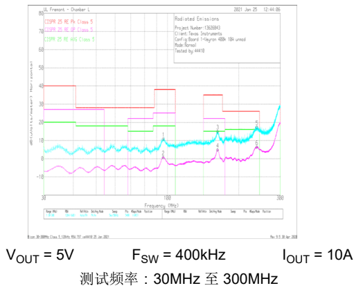
图 8-47. 辐射 EMI 双锥水平与 CISPR25 5 类限值
