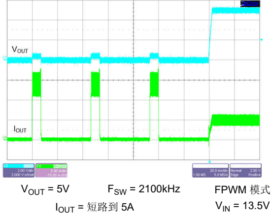
图 8-35. 短路恢复
