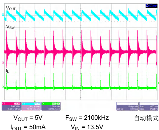
图 8-29. 开关波形和 V_{OUT} 纹波
