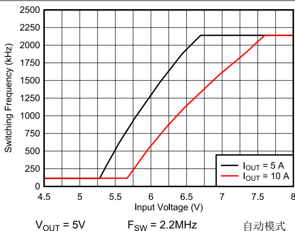
图 8-27. 频率压降
