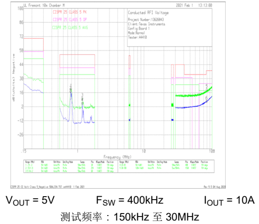
图 8-46. 传导 EMI 与 CISPR25 5 类限值 (绿色: 峰值信号, 蓝色: 平均信号)
