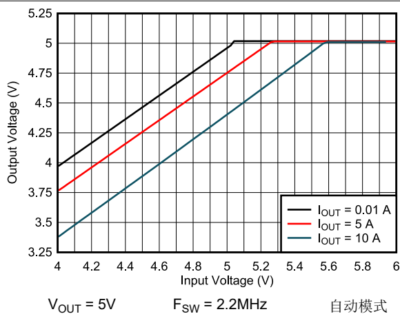
图 8-23. 压降
