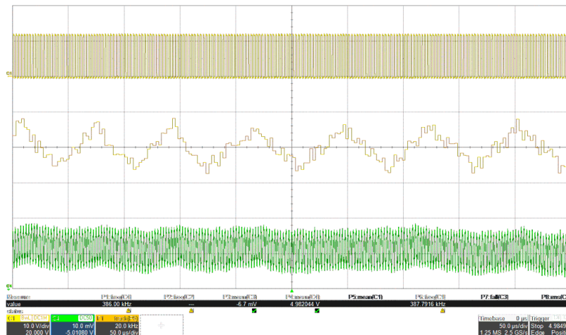
图 7-12. 具有纹波消除功能的输出纹波显示 V_{\text{sw}} (顶部)、 F_{\text{sw}} (中间)、 V_{\text{out}} (底部)
