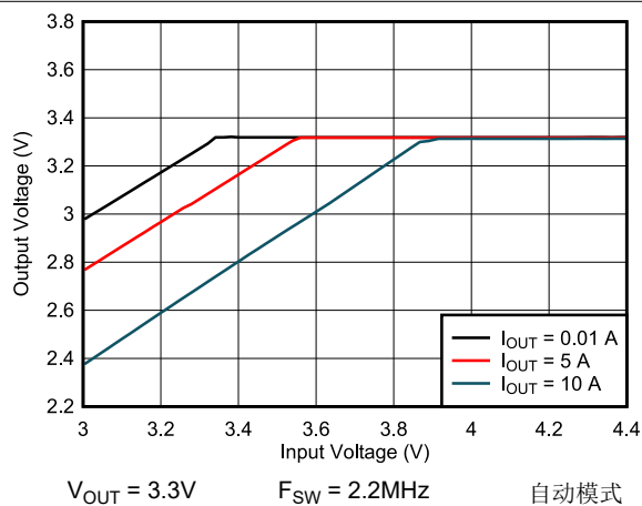
图 8-24. 压降
