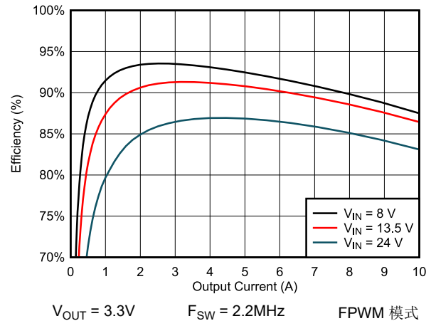
图 8-12. 效率
