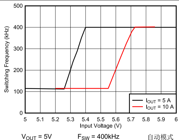
图 8-25. 频率压降
