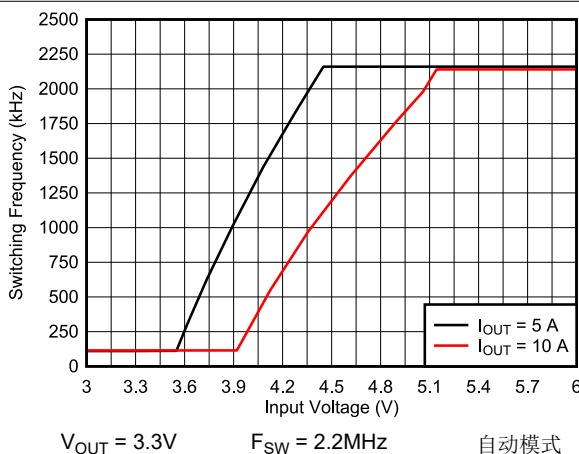
图 8-28. 频率压降
