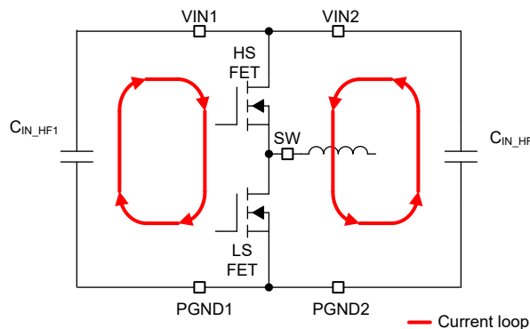
图 8-58. 输入电流环路
