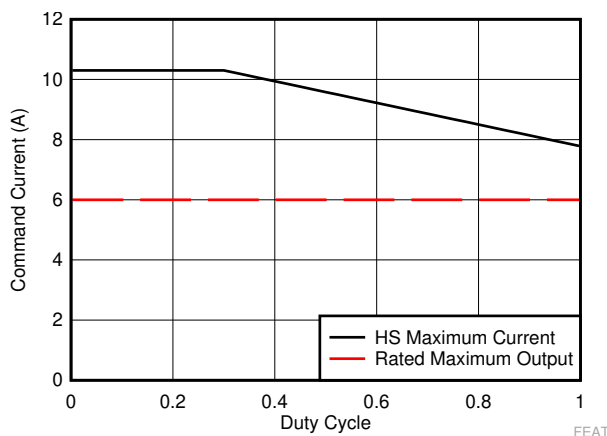
图 7-15. 允许流经 HS FET 的最大电流 - LM62460-Q1 占空比的函数
