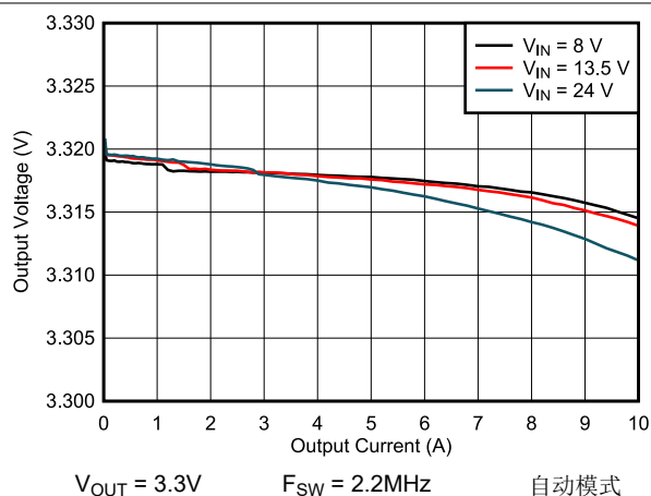
图 8-19. 负载调整率和线性调整率
