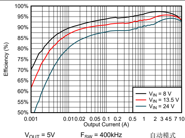
图 8-5. 效率
