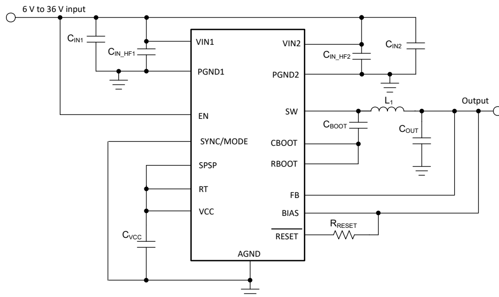
图 8-2. 示例应用电路 - 400kHz 固定输出
