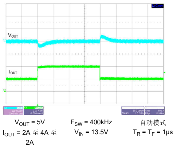
图 8-39. 负载瞬态
