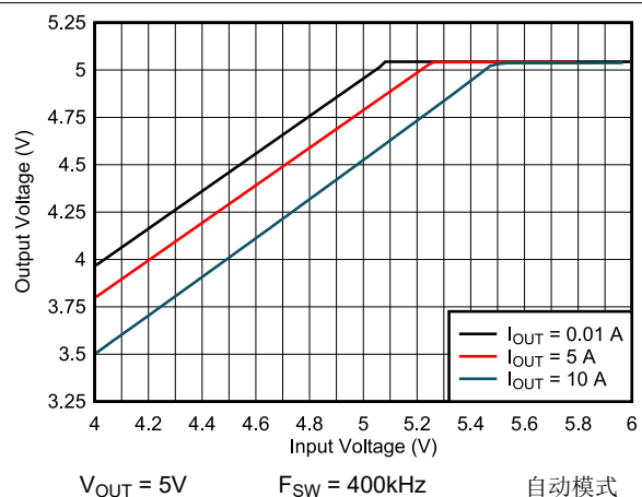
图 8-21. 压降
