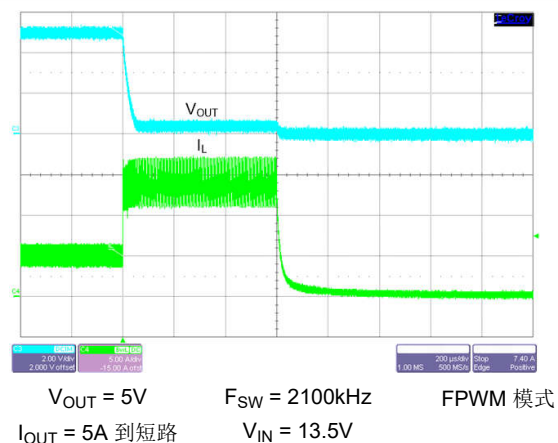
图 8-34. 短路保护
