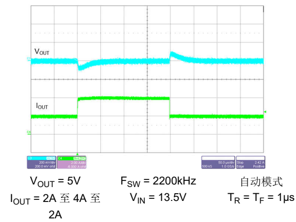
图 8-44. 负载瞬态
