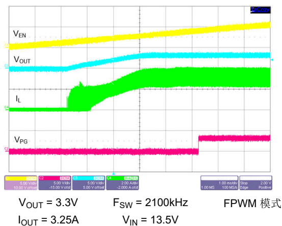
图 8-33. 在 3.25A 负载下启动
