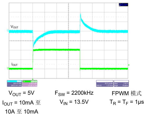
图 8-43. 负载瞬态
