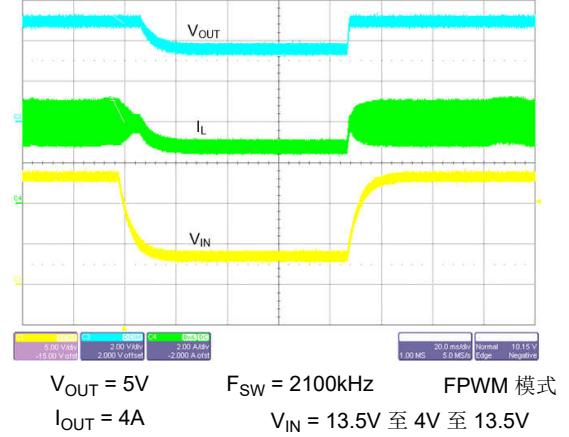
图 8-36. 从压降中恢复
