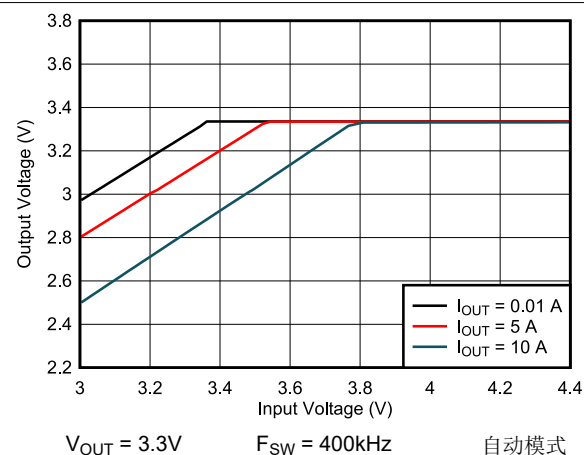
图 8-22. 压降
