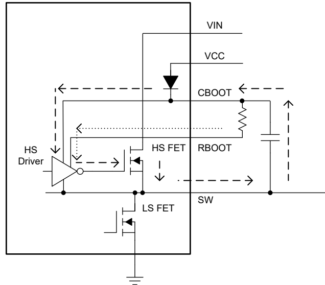
图 7-10. 显示 RBOOT 功能的简化电路
