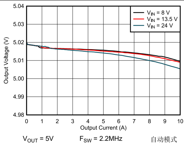
图 8-17. 负载调整率和线性调整率
