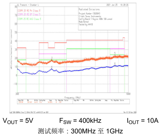
图 8-49. 辐射 EMI 对数水平与 CISPR25 5 类限值
