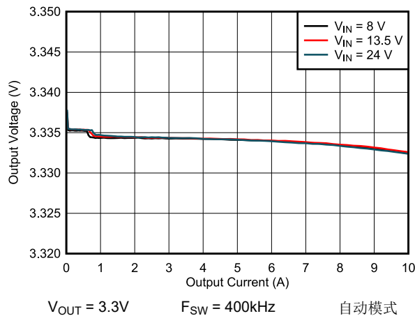
图 8-15. 负载调整率和线性调整率
