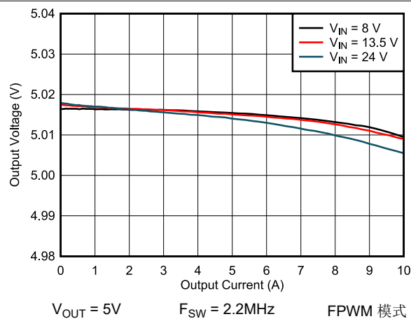
图 8-18. 负载调整率和线性调整率
