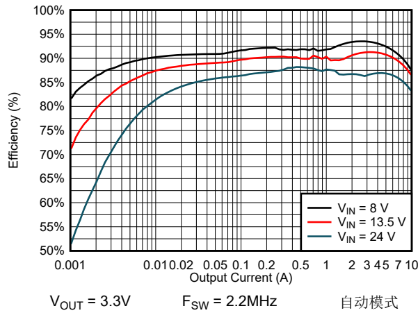
图 8-11. 效率
