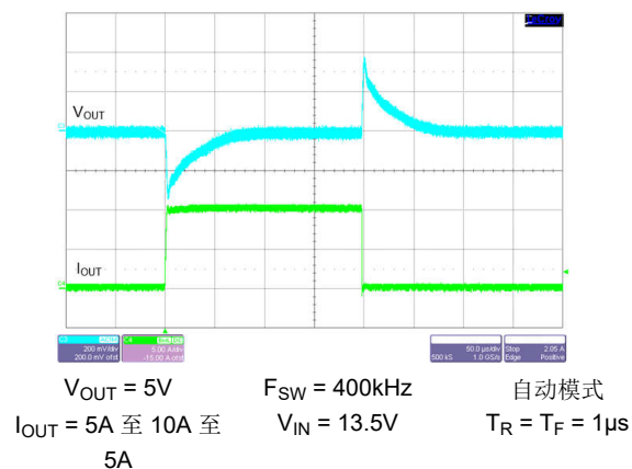
图 8-40. 负载瞬态
