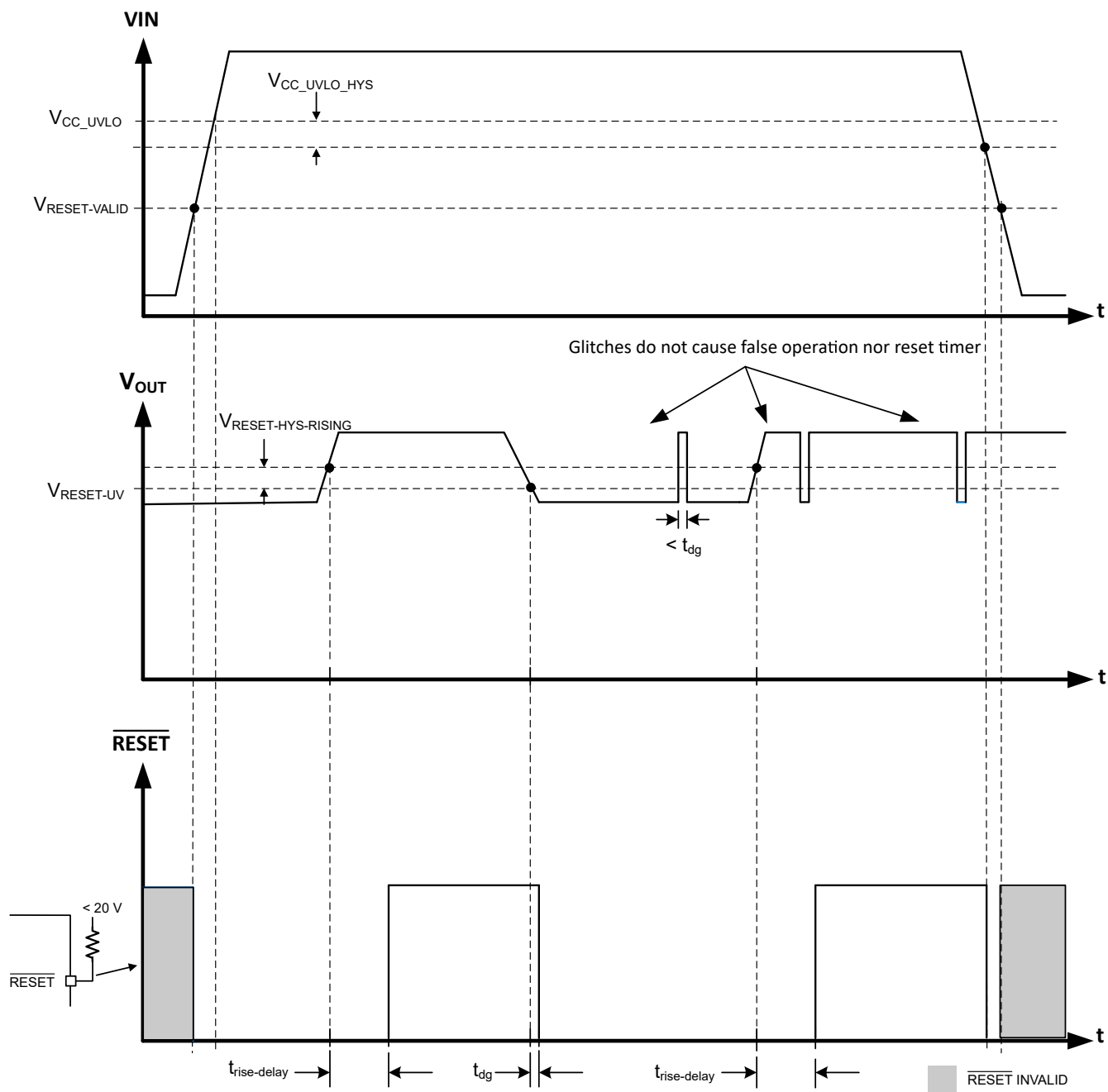
图 7-8. RESET 时序图 (不包括 OV 事件)
