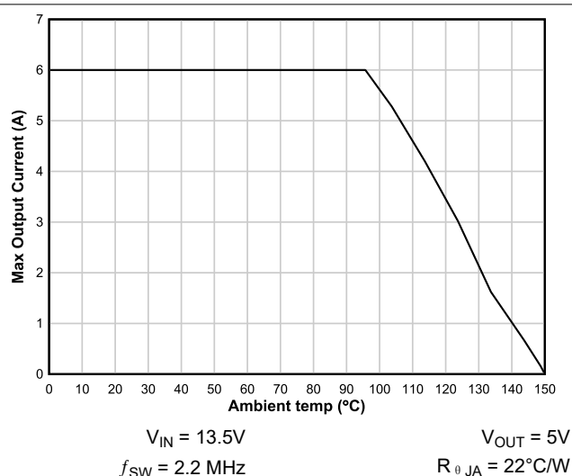
图 8-4. 最大输出电流与环境温度间的关系
