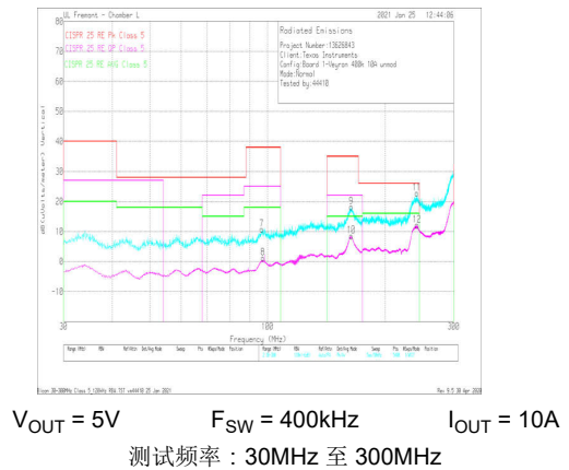
图 8-48. 辐射 EMI 双锥垂直与 CISPR25 5 类限值
