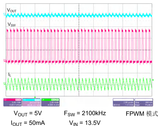
图 8-30. 开关波形和 V_{OUT} 纹波
