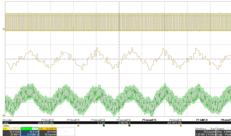
图 7-11. 没有纹波消除功能的输出纹波显示 V_{\text{sw}} (顶部)、 F_{\text{sw}} (中间)、 V_{\text{out}} (底部)
