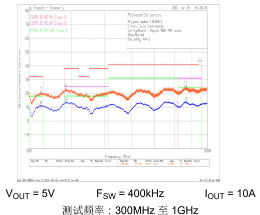
图 8-50. 辐射 EMI 对数垂直与 CISPR25 5 类限值
