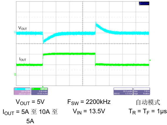
图 8-45. 负载瞬态
