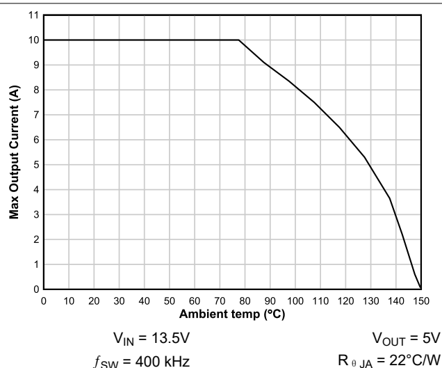
图 8-3. 最大输出电流与环境温度间的关系
