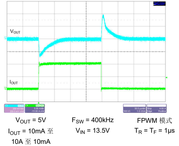
图 8-38. 负载瞬态
