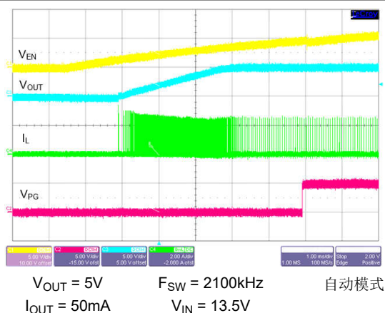
图 8-31. 在 50mA 负载下启动
