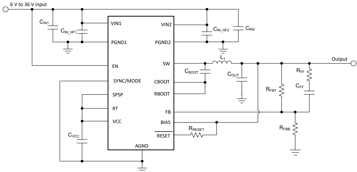
图 8-1. 示例应用电路 - 400kHz 可调节输出
