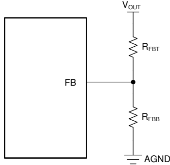
图 7-1. 设置可调版本的输出电压
