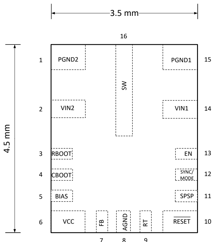
图 5-1. 16 引脚 VQFN-HR RPH 封装 ( 顶视图 )
