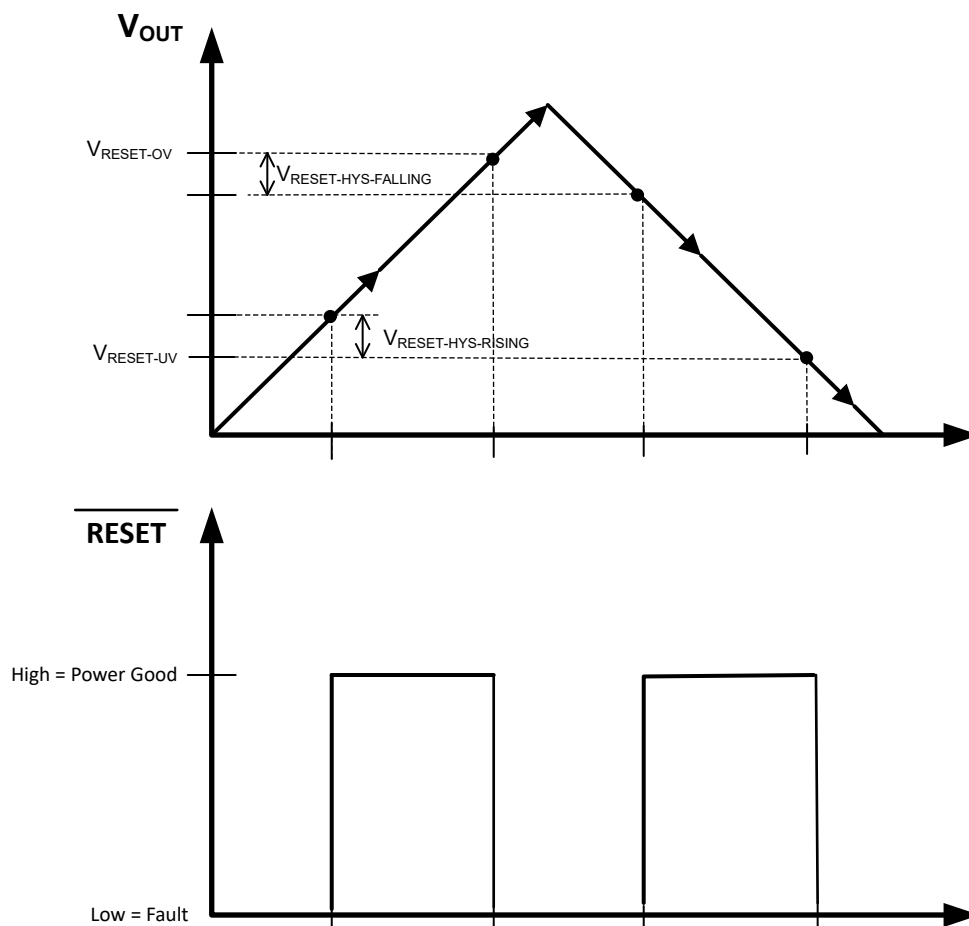
图 7-7. \overline{RESET} 静态电压阈值
