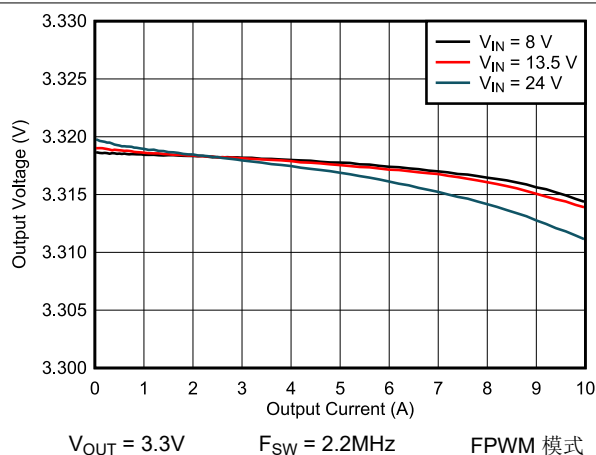
图 8-20. 负载调整率和线性调整率
