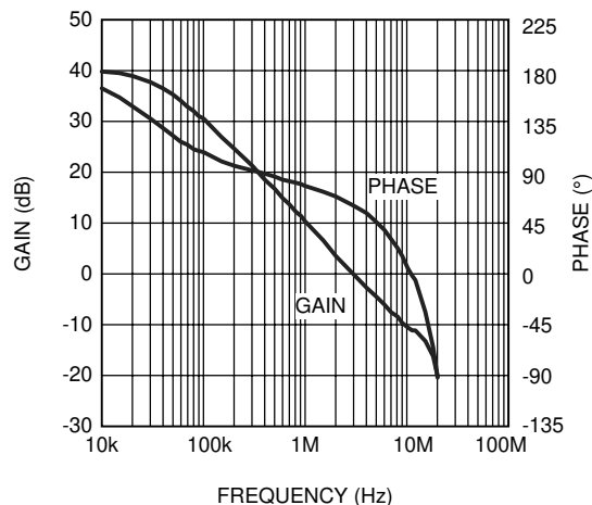
图 5-6. 误差放大器增益/相位 A_{VCL} = 101
