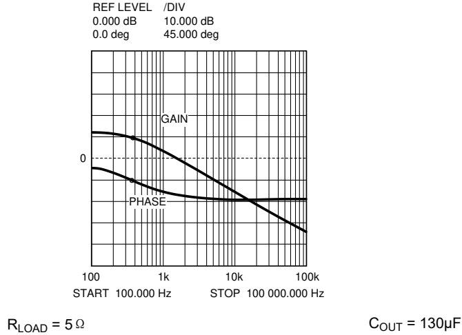
图 7-5. 调制器的增益和相位
