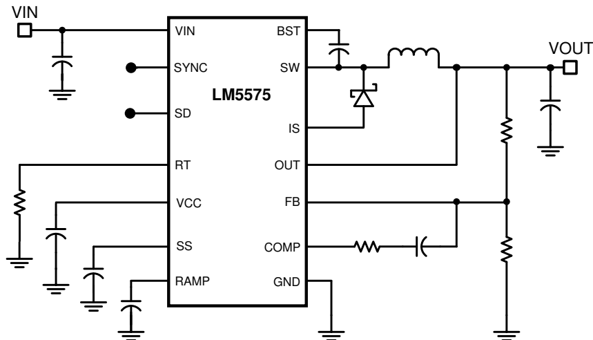
简化版原理图
