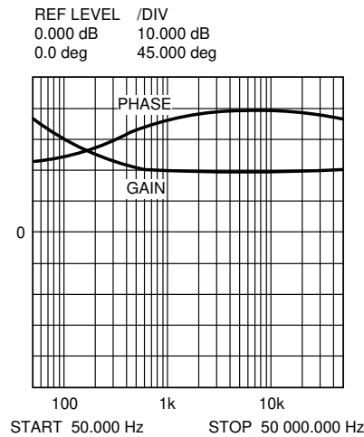
图 7-6. 误差放大器增益与相位
