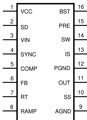
图 4-1. PWP 封装，16 引脚 HTSSOP (带外露散热焊盘) (顶视图)
