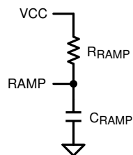
图 6-6. V_{OUT} > 7.5V 时, R_{RAMP} 连接 V_{CC}
