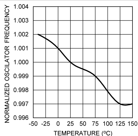
图 5-2. 振荡器频率与温度间的关系 F_{OSC} = 200\text{kHz}
