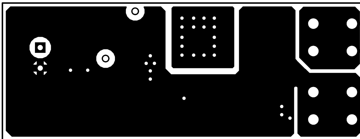
图 7-12. 焊接侧
