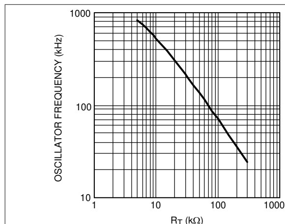
图 7-8. 振荡器频率与 R_T 间的关系
