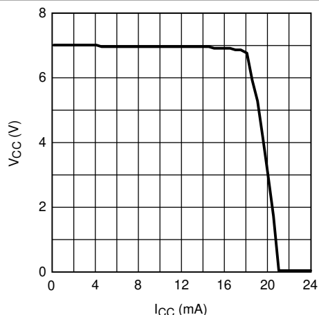
图 5-4. V_{CC} 与 I_{CC} 间的关系 V_{IN} = 12\text{V}
