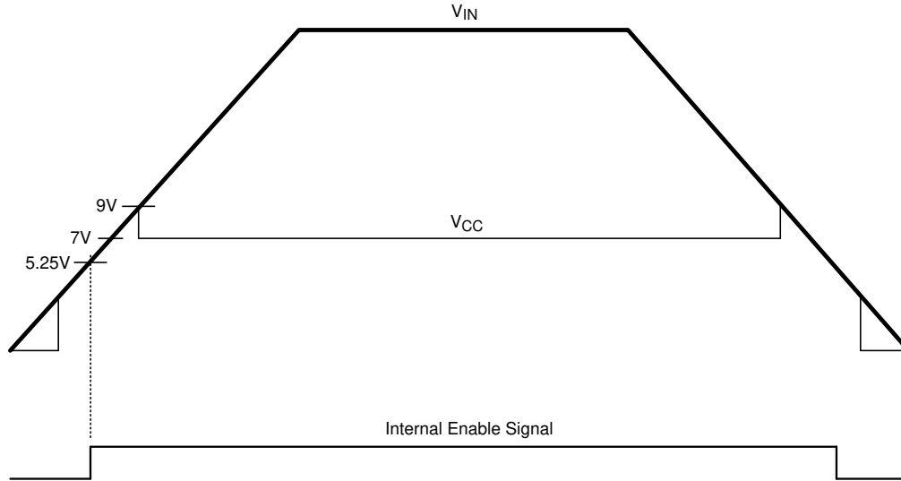
图 6-1. V_{IN} 和 V_{CC} 时序
