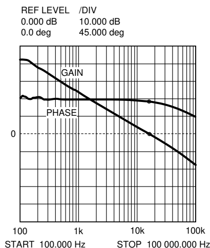
图 7-7. 总体环路增益与相位
