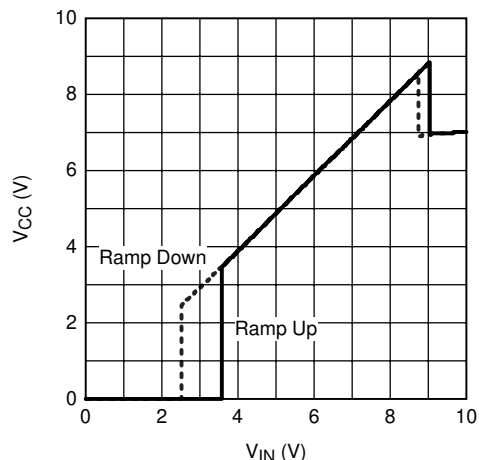
图 5-5. V_{CC} 与 V_{IN} 间的关系 R_L = 7\text{k}\Omega
