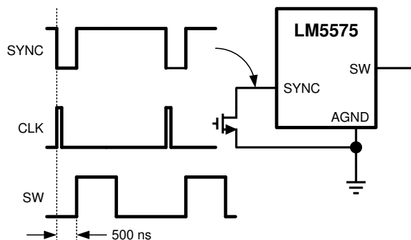
图 6-2. 与外部时钟同步
