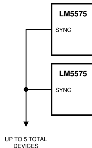
图 6-3. 从多个设备同步
