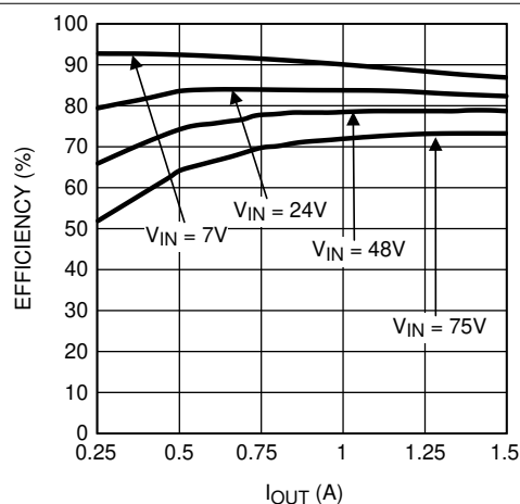
图 7-9. 电路板效率与 I_{OUT} 和 V_{IN} 间的关系
