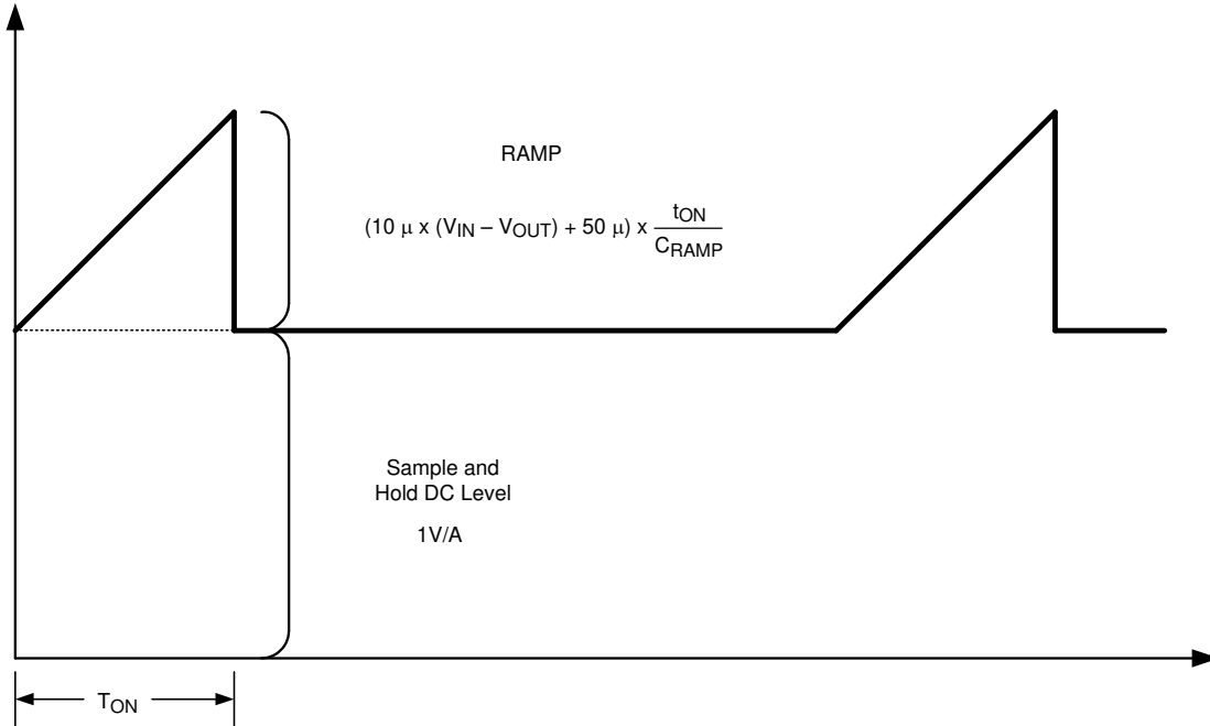
图 6-5. 电流检测信号的组成
