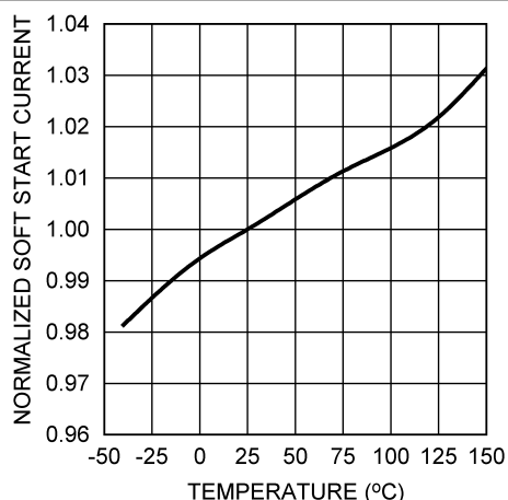
图 5-3. 软启动电流与温度间的关系
