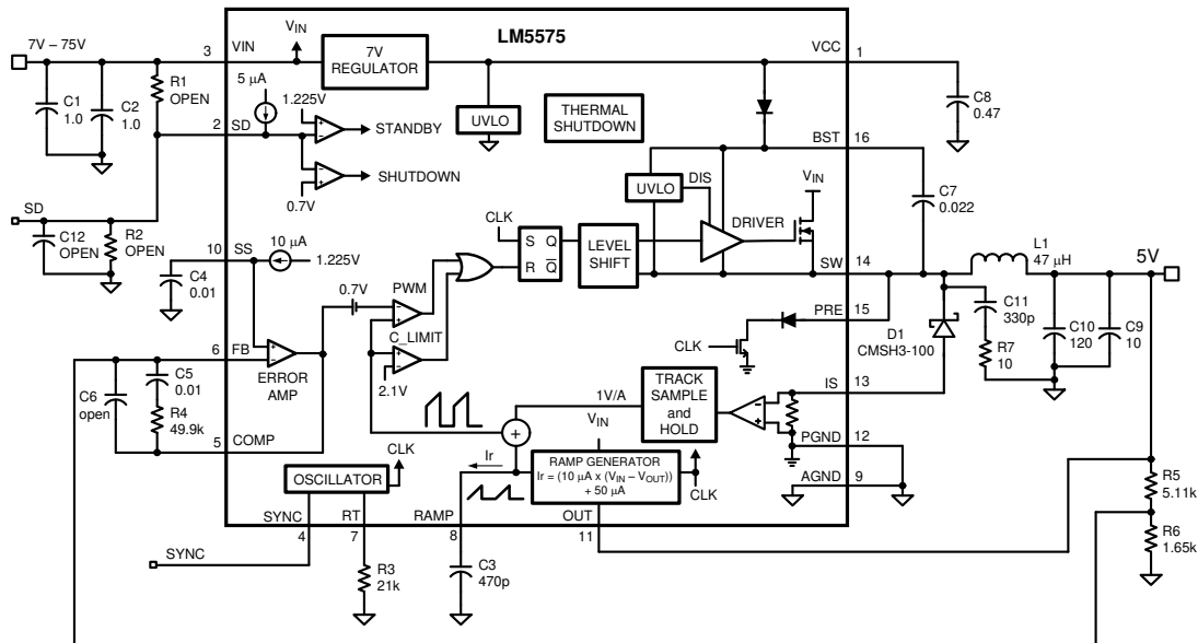
图 7-3. 典型应用电路
