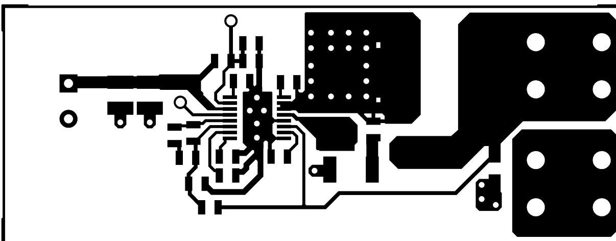
图 7-11. 组件侧
