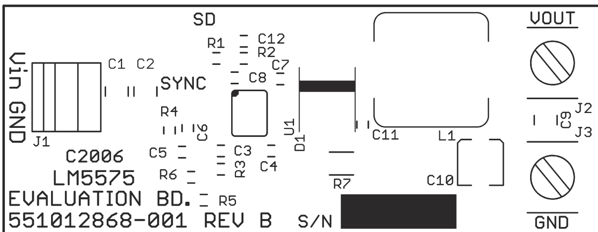
图 7-10. 丝印
