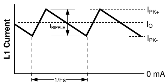
图 7-4. 电感器电流波形
