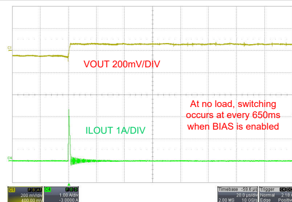
图 9-9. PFM 模式、 V_{SUPPLY} = 48V 、 I_{LOAD} = 0A 条件下的空载运行
