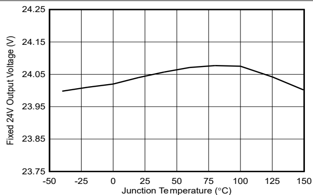
图 6-8. 固定输出电压与温度间的关系, V_{OUT} = 24V
