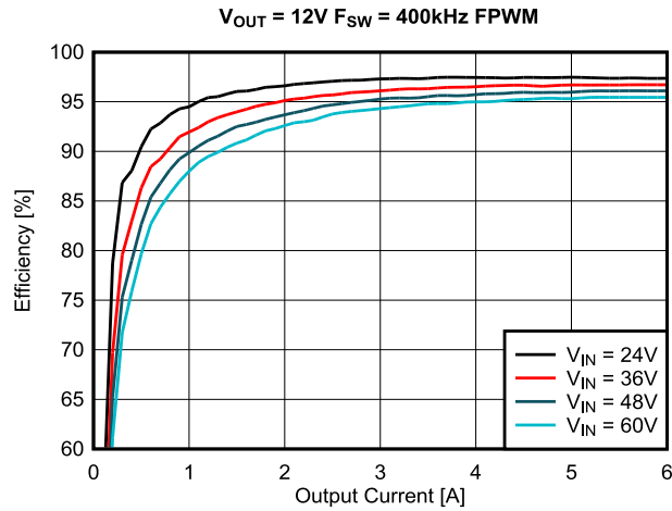
图 9-4. FPWM 模式效率，线性标度
