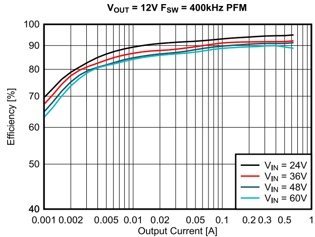
图 9-5. PFM 模式效率，对数标度
