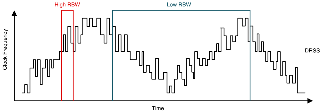
图 7-2. 双随机展频实现
