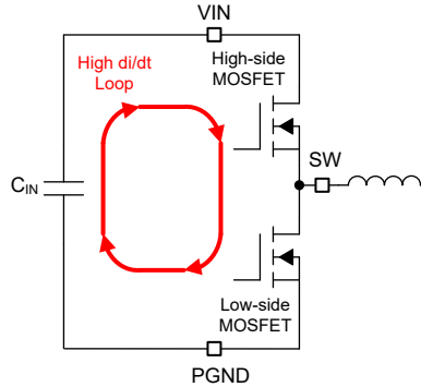
图 9-14. 输入电流环路
