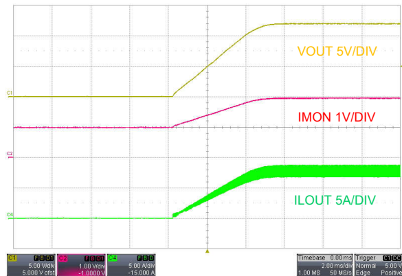
图 9-6. 启动，EN 开启， V_{SUPPLY} = 48V ， I_{LOAD} = 8A 电阻负载
