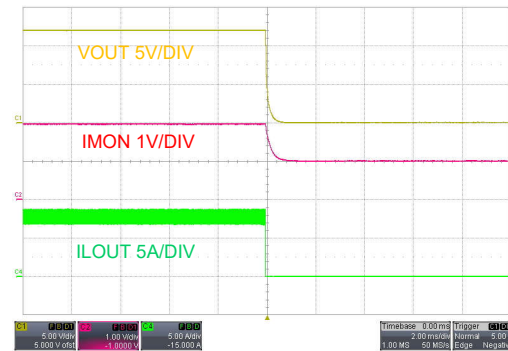
图 9-7. 关断，EN 关闭， V_{SUPPLY} = 48V ， I_{LOAD} = 8A 电阻负载
