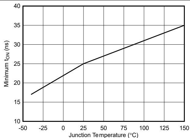
图 6-12. 最短导通时间与温度间的关系
