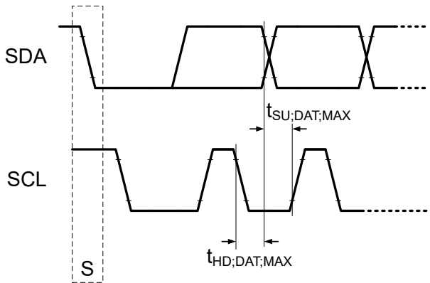
图 7-10. 最长上升和下降时间的 I 2 C 数据传输时序
