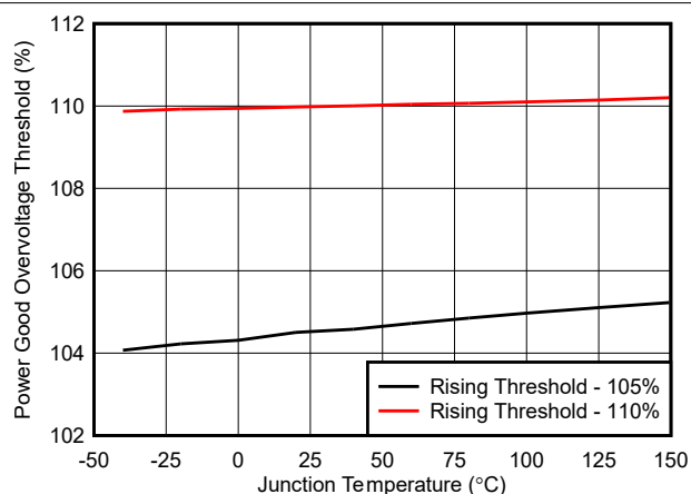
图 6-10. PG 过压阈值与温度间的关系
