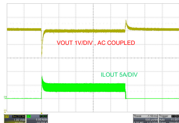
图 9-11. V_{\text{SUPPLY}} = 48\text{V} 、PFM、从 0A 变为 4A 时的负载瞬态响应
