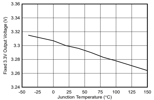
图 6-6. 固定输出电压与温度间的关系, V_{OUT} = 3.3\text{V}
