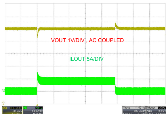
图 9-10. V_{\text{SUPPLY}} = 48\text{V} 、FPWM、从 0A 变为 4A 时的负载瞬态响应
