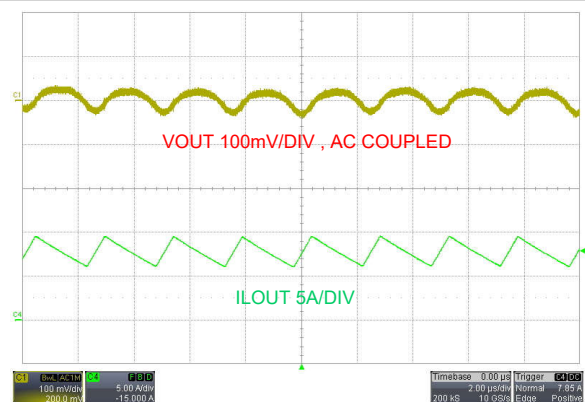
图 9-8. 输出纹波， V_{SUPPLY} = 48V ， I_{LOAD} = 8A
