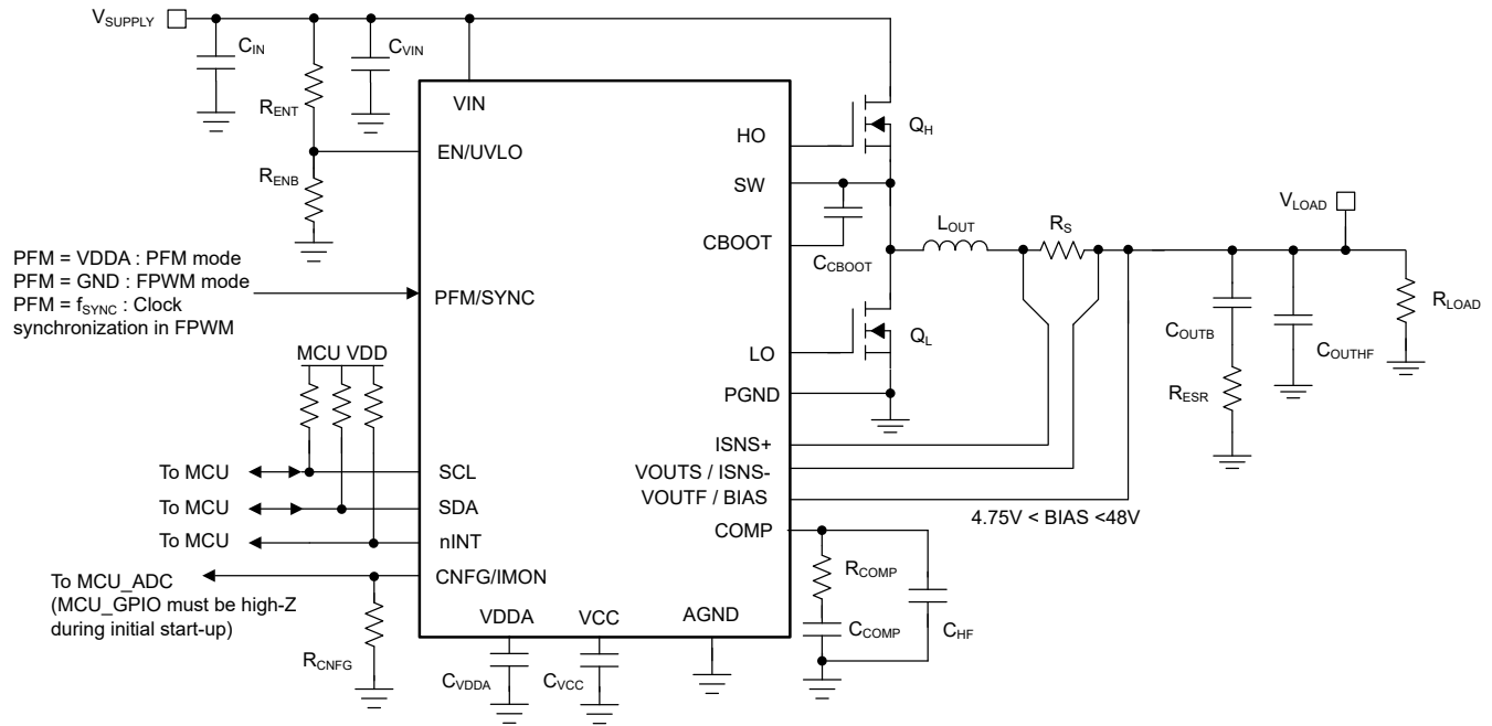
图 9-3. 具有 I 2 C 接口的应用电路
