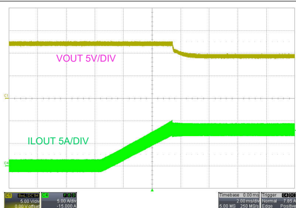
图 9-12. CV 至 CC 模式转换, V_{\text{SUPPLY}} = 48\text{V} , V_{\text{LOAD}} = 12\text{V} 至 9\text{V}
