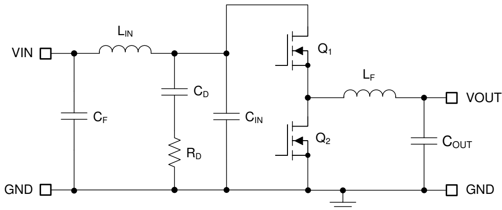
图 9-2. 具有 \pi 级 EMI 滤波器的降压稳压器
