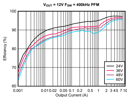
LM5192 效率
