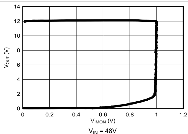
图 5-18. 充电瞬态期间的恒流恒压运行
