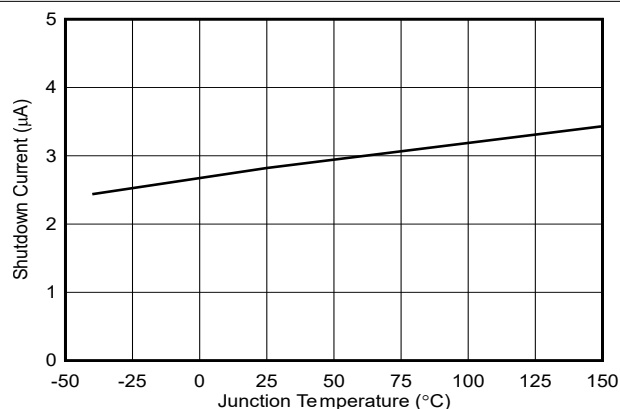
图 5-1. 关断电流与温度间的关系
