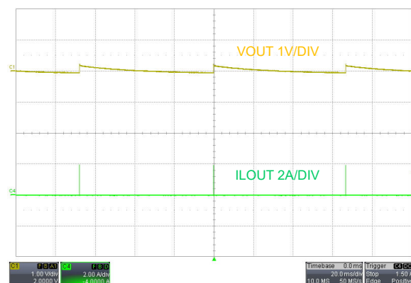
图 7-10. PFM 模式、 V_{SUPPLY} = 48V 、 I_{LOAD} = 0A 条件下的空载运行
