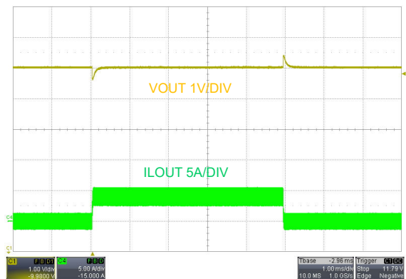
图 7-11. V_{\text{SUPPLY}} = 48\text{V} 、FPWM、从 0A 变为 4A 时的负载瞬态响应
