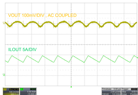
图 7-9. 输出纹波， V_{SUPPLY} = 48V ， I_{LOAD} = 8A
