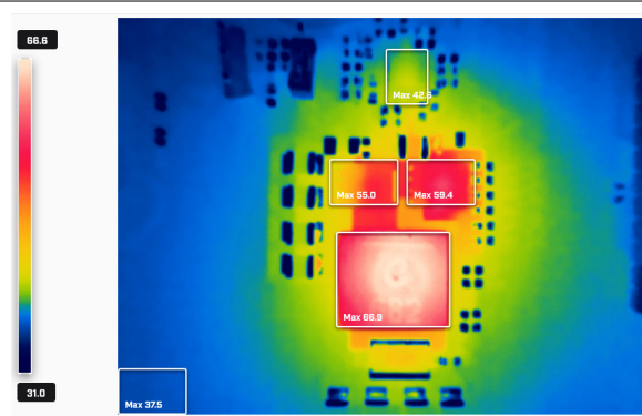
图 7-14. V_{\text{SUPPLY}} = 48\text{V} , I_{\text{LOAD}} = 8\text{A} , T_A = 25^\circ\text{C} , 无气流
