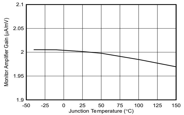
图 5-16. 监测放大器增益与温度间的关系
