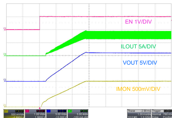
图 7-7. 启动，EN 开启， V_{SUPPLY} = 48V ， I_{LOAD} = 8A 电阻负载
