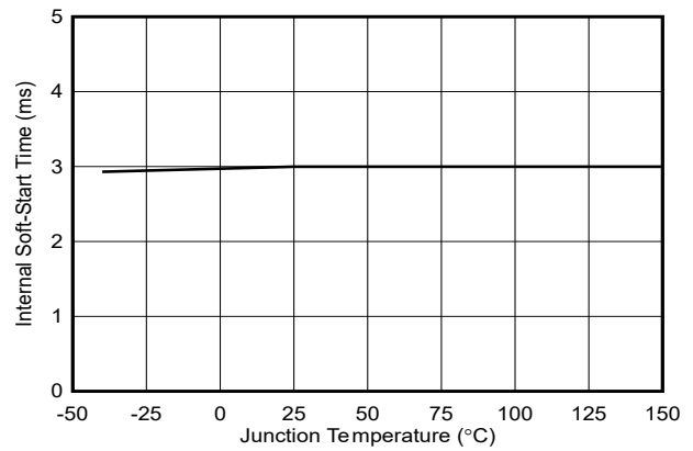
图 5-14. 软启动时间与温度间的关系
