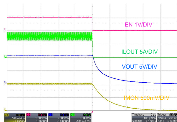
图 7-8. 关断，EN 关闭， V_{SUPPLY} = 48V ， I_{LOAD} = 8A 电阻负载
