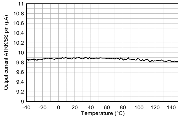
图 5-15. 软启动电流与温度间的关系
