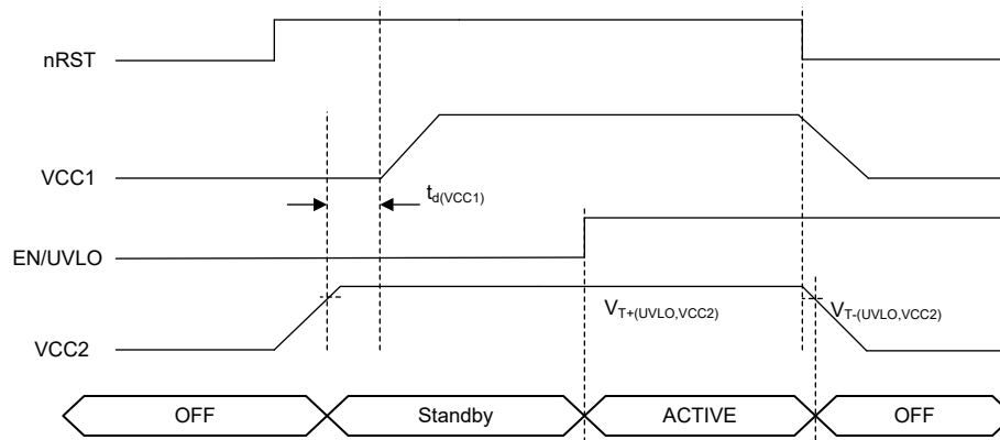
图 7-16. VCC 稳压器时序图
