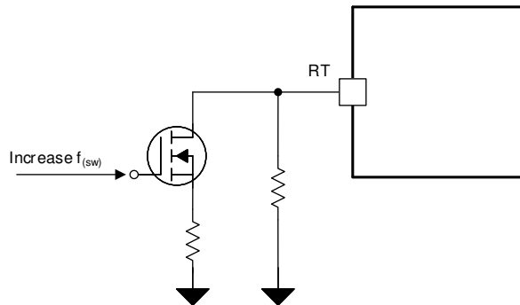
图 7-23. 跳频示例
