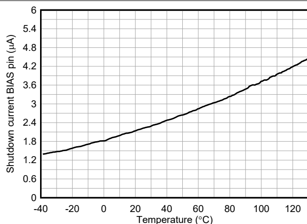
图 5-7. 流入 BIAS 的关断电流与温度间的关系 V_{EN/UVLO} = 0V , V_{(VIN)} = 3.5V , V_{(BIAS)} = 12V
