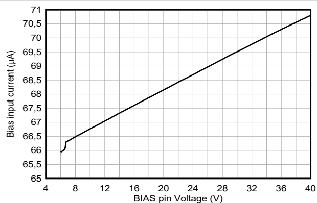
图 5-8. 流入 BIAS 的静态电流与 BIAS 引脚电压间的关系 V_{(VIN)} = 3.5V
