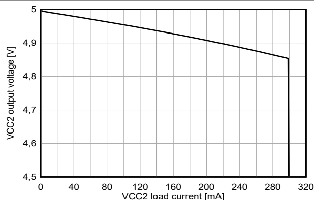
图 5-11. VCC2 LDO 输出电压与 VCC2 负载电流间的关系 V_{(VIN)} = 12V , V_{(BIAS)} = 0V
