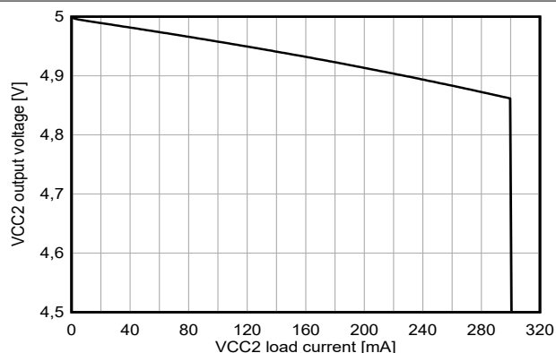
图 5-12. VCC2 LDO 输出电压与 VCC2 负载电流间的关系 V_{(VIN)} = 3.5V , V_{(BIAS)} = 12V
