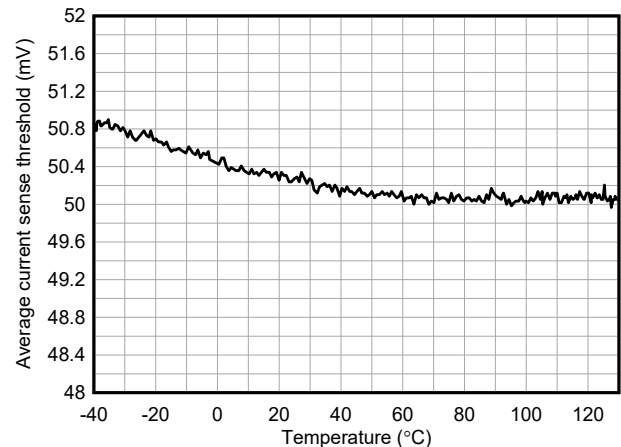
图 5-28. 平均电流限制阈值电压与温度间的关系 ILIM\_THRESHOLD = 0x64
