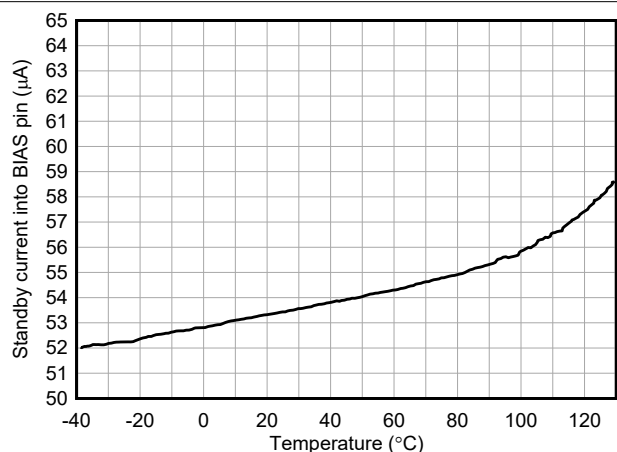
图 5-10. 流入 BIAS 的待机电流与温度间的关系 V_{(VIN)} = 3.5V , V_{(VIN)} = 12V
