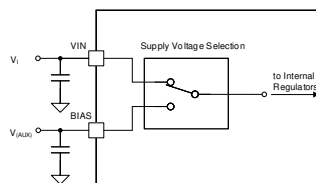
图 7-13. VSMART 电源方案 2
