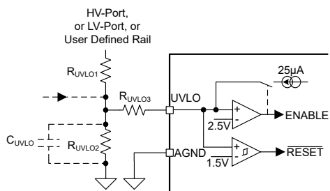
图 6-32. UVLO 及额外迟滞编程
