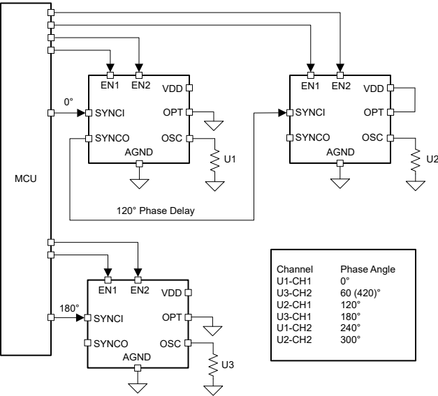
图 6-26. 使用外部时钟移位的六相 60° 交错配置
