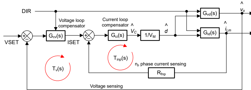
图 7-5. 电压环路和电流环路方框图
