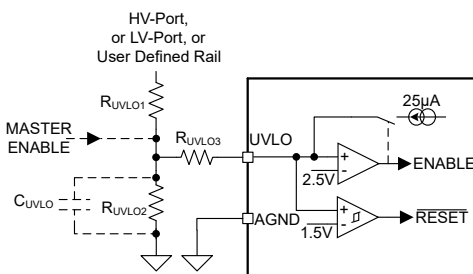
图 6-31. UVLO 编程
