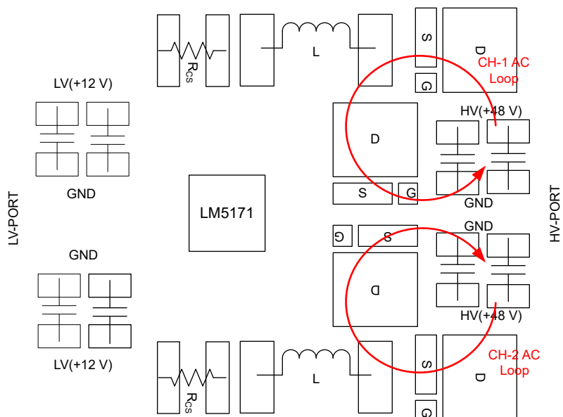
图 7-33. 双通道电源电路放置的布局示例
