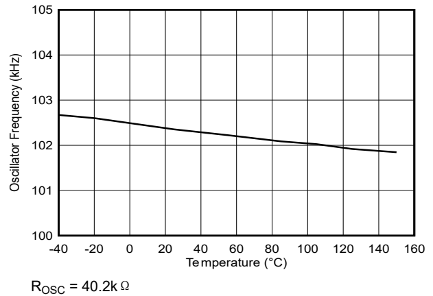
图 5-4. 振荡器频率与温度间的关系
