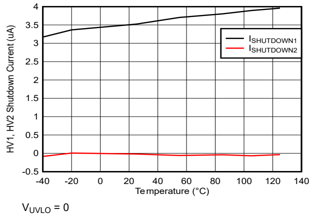
图 5-1. 关断电流与温度间的关系
