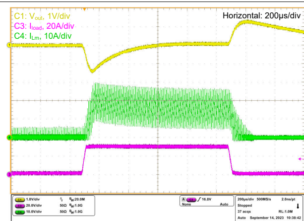
图 7-17. 阶跃负载响应：降压模式；DEM；1A 至 30A 负载阶跃；1A/µs
