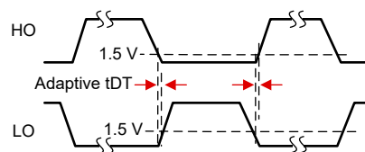
图 6-18. 自适应死区时间 ( 仅显示一个通道 )
