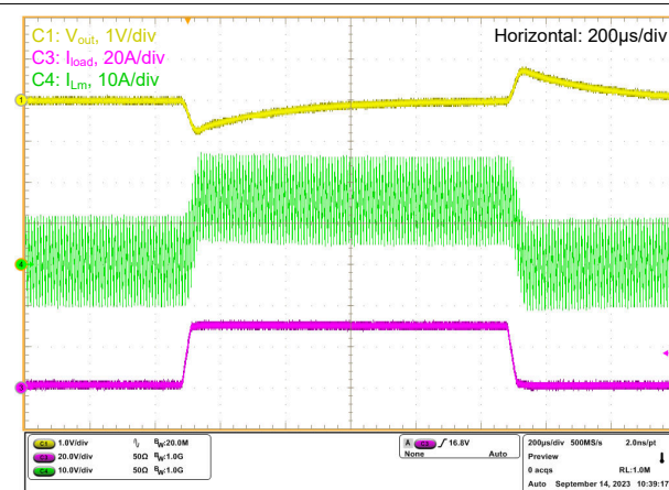
图 7-18. 阶跃负载响应：降压模式；FPWM；1A 至 30A 负载阶跃；1A/µs
