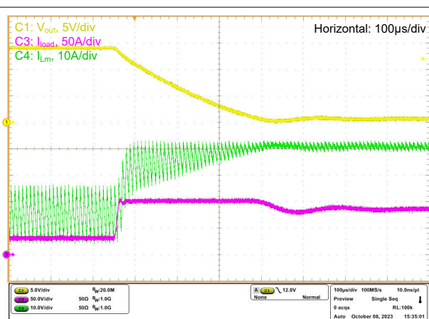
图 7-31. 输出短路：降压模式
