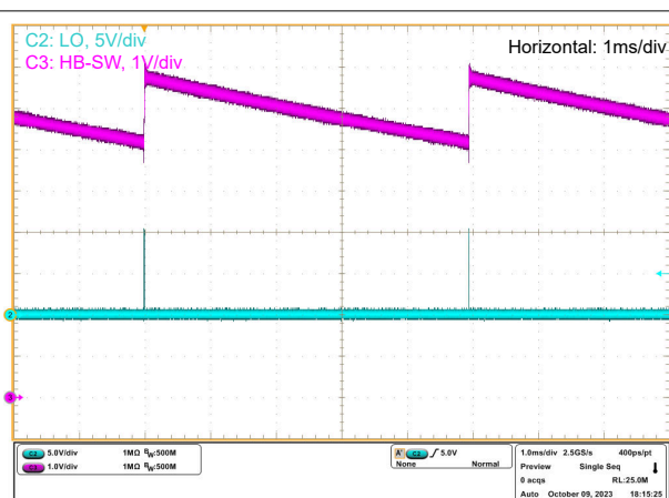
图 7-29. 预充电：降压模式， I_{load} = 0A
