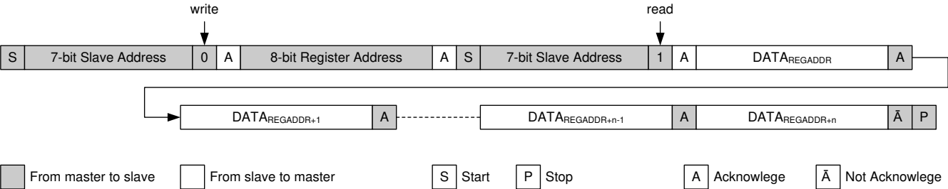
图 6-37. 从定义的寄存器地址开始进行顺序读取
