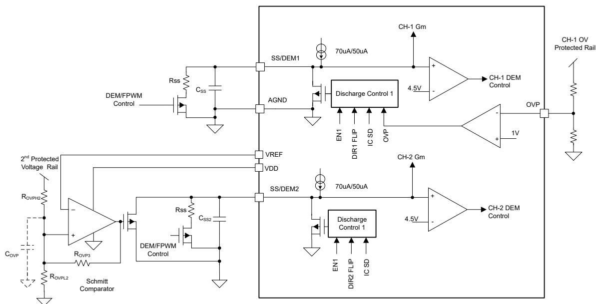
图 6-24. 独立通道运行模式下的 OVP 实现方式
