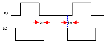
图 6-16. 栅极驱动死区时间 (仅显示一个通道)
