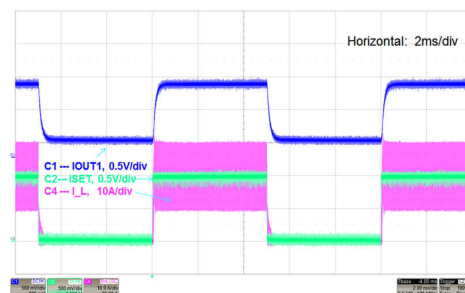
通道电流跟踪 ISETA 命令
