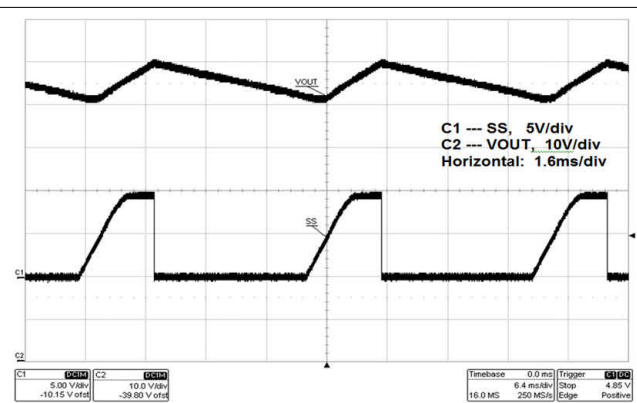
图 9-23. HV-Port OVP: Boost Mode
