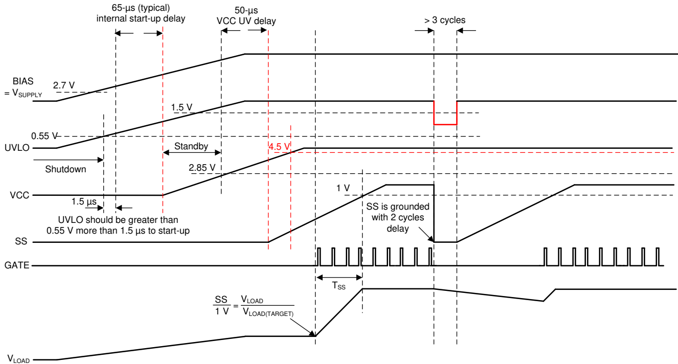
图 9-2. 升压启动波形情况 1：通过 2.85\text{V} VCC UVLO 启动，启动后进行 UVLO 切换
