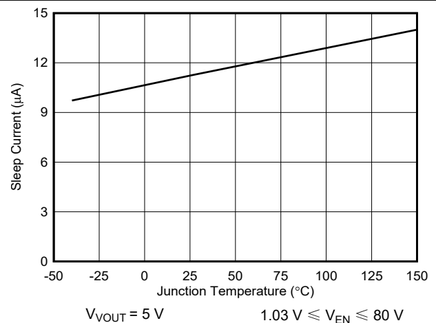
图 7-6. Sleep Current vs Temperature
