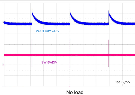
图 9-33. PFM Switching
