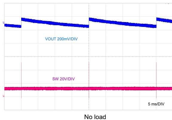
图 9-21. PFM Switching
