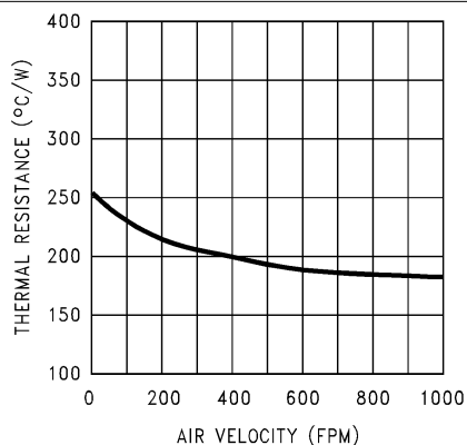
图 6-1. 结至环境热阻 (旧芯片)
