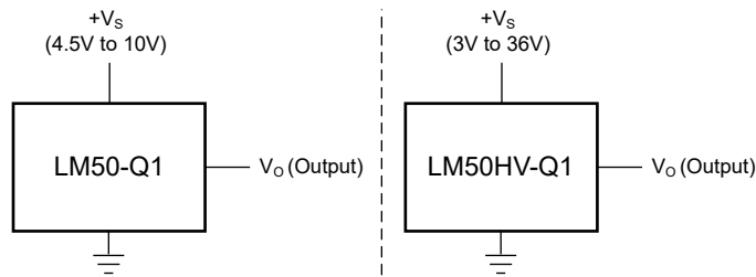
图 8-1. 全范围摄氏温度传感器 LM50-Q1 ( -40°C 至 125°C ) 和 LM50HV-Q1 ( -40°C 至 150°C )
