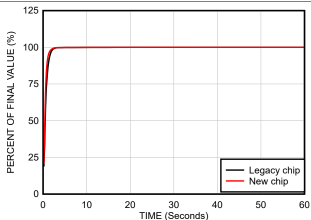
图 6-6. 不带散热器时搅拌油浴中的热响应
