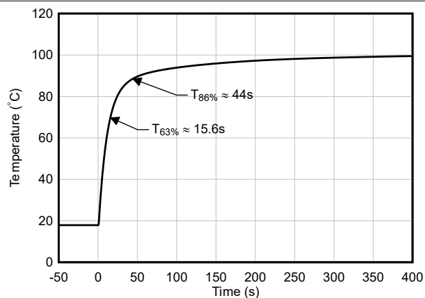
图 6-32. 静止空气中的热响应 (0.5 英寸 × 0.5 英寸 PCB 板)
