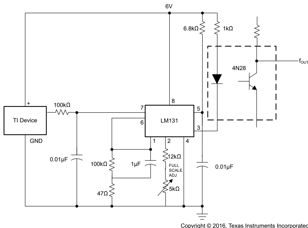
图 8-12. 具有压频转换器和隔离式输出的 LM50-Q1 和 LM50HV-Q1
