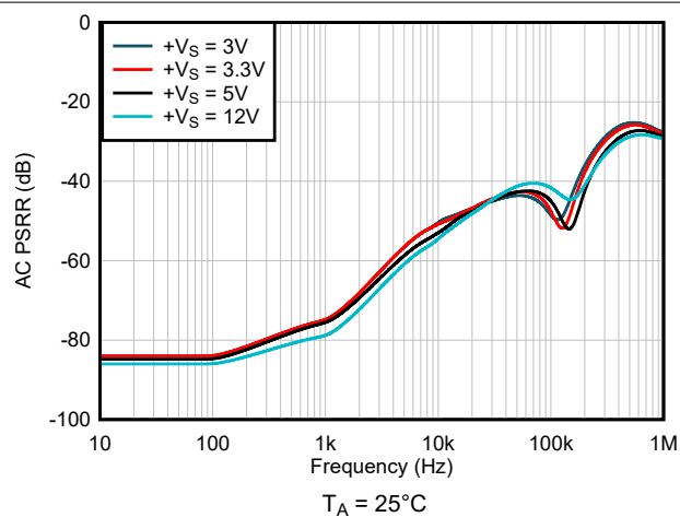
图 6-34. 电源抑制比与频率间的关系
