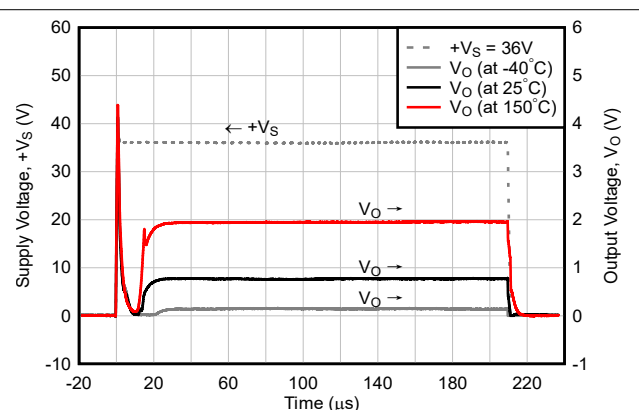
图 8-5. +V_S = 36V 阶跃时的启动响应（当 t_r = 1\mu s ，无 C_{Load} 和 C_{By-pass} 时）
