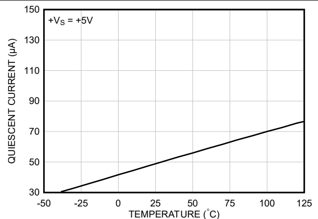
图 6-12. 静态电流与温度之间的关系 ( 新芯片 )
