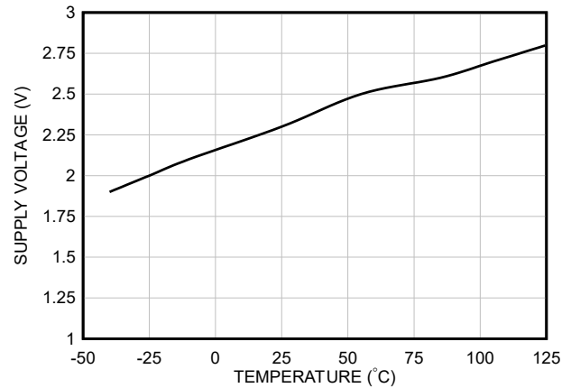
图 6-10. 启动电压与温度之间的关系 ( 新芯片 )
