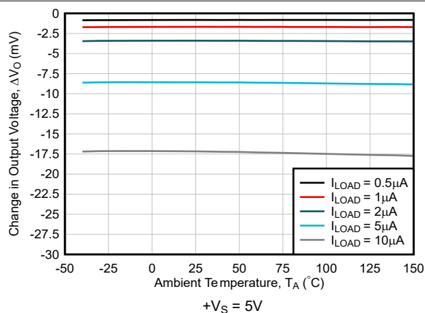
图 6-27. 负载调节与环境温度间的关系
