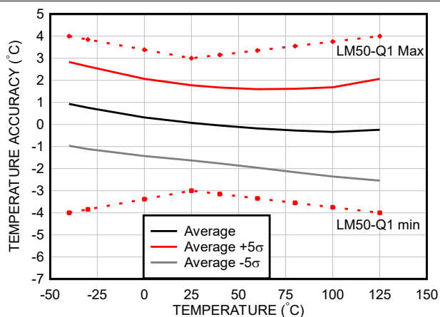
图 6-14. 精度与温度之间的关系 ( 新芯片 )
