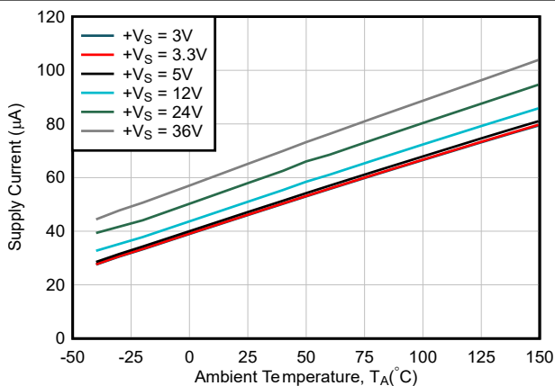
图 6-25. 电源电流与环境温度间的关系
