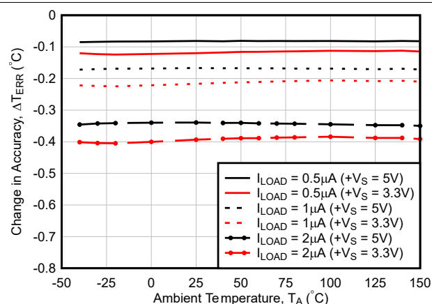
图 6-24. 精度与温度变化间的关系
