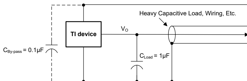
图 8-3. 具有滤波器且适用于噪声环境的 LM50-Q1 和 LM50HV-Q1
