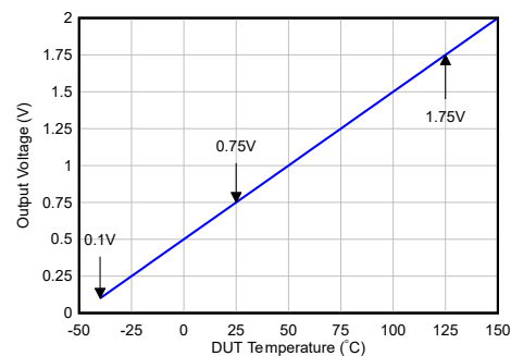
图 3-2. 全范围 LM50-Q1 ( -40^{\circ}\text{C} 至 125^{\circ}\text{C} ) 和 LM50HV-Q1 ( -40^{\circ}\text{C} 至 150^{\circ}\text{C} )
