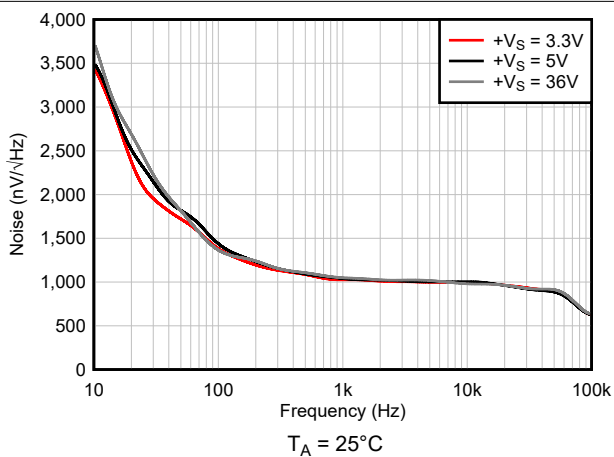
图 6-35. 输出噪声密度
