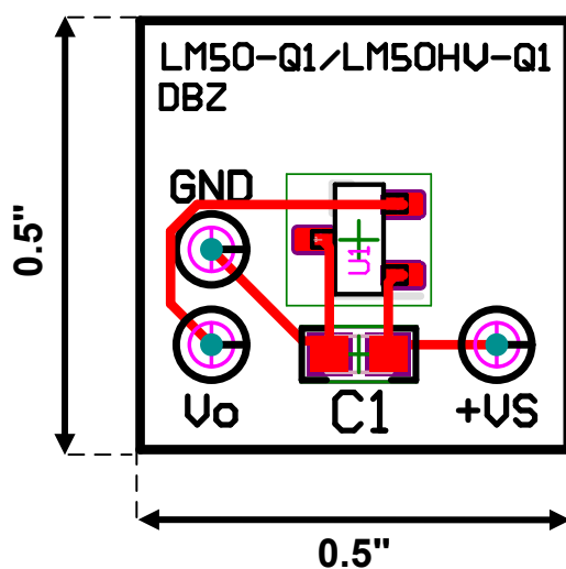
图 8-15. 用于生成热响应曲线的印刷电路板 [LM50-Q1 (新芯片和旧芯片) 和 LM50HV-Q1 的新测试设置]
