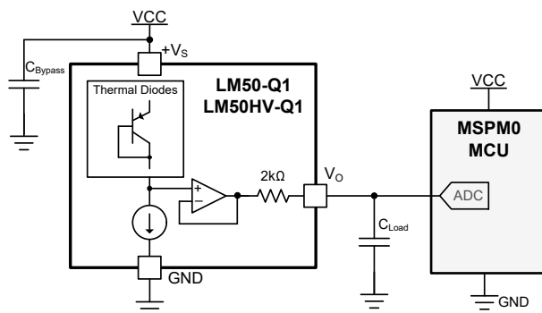
图 3-1. 简化版原理图
