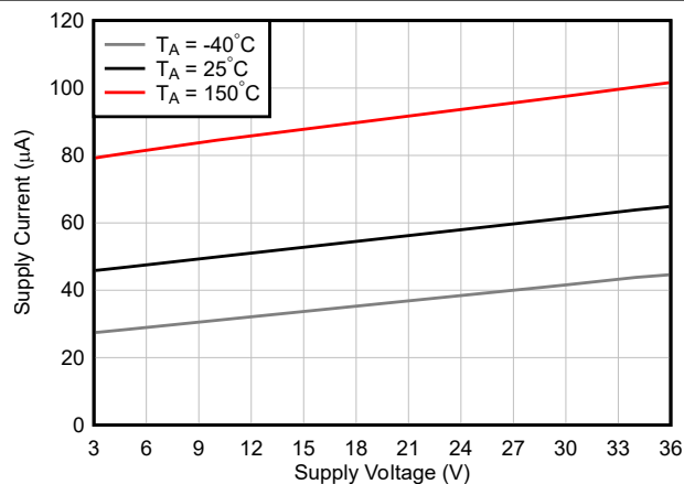
图 6-26. 电源电流与电源电压间的关系
