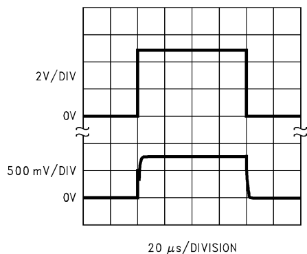
图 6-19. 启动响应 ( 旧芯片 )
