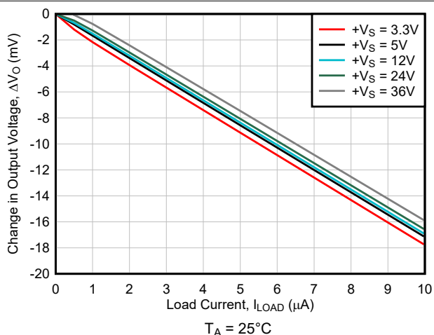
图 6-28. 输出电压与负载电流变化间的关系
