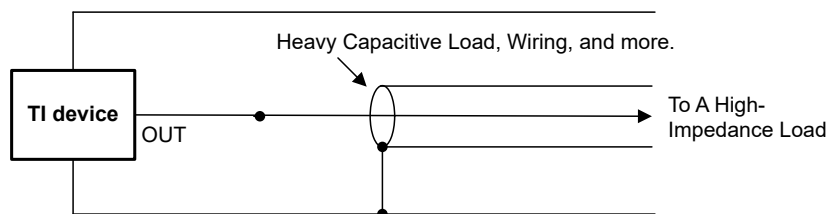
图 8-2. LM50-Q1 和 LM50HV-Q1 电容负载无需去耦
