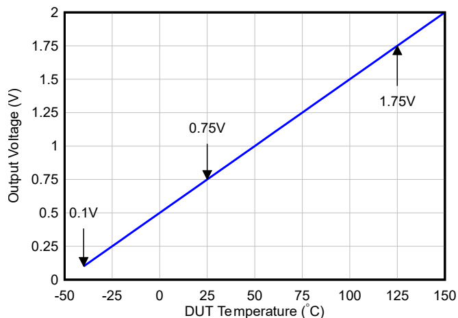
图 8-9. 输出传递函数
