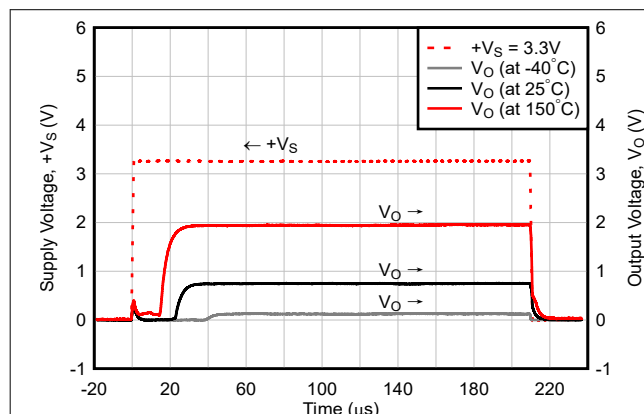
图 8-4. +V_S = 3.3V 阶跃时的启动响应（当 t_r = 1\mu s 、无 C_{Load} 和 C_{By-pass} 时）
