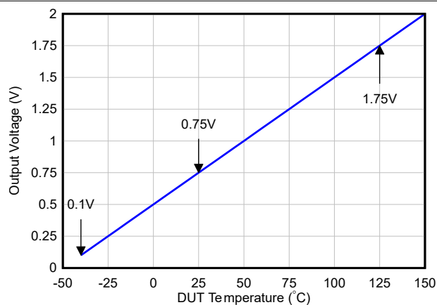
图 6-22. V_O 与环境温度间的关系
