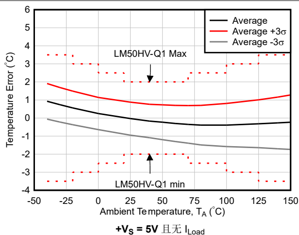
图 6-21. 精度与环境温度间的关系
