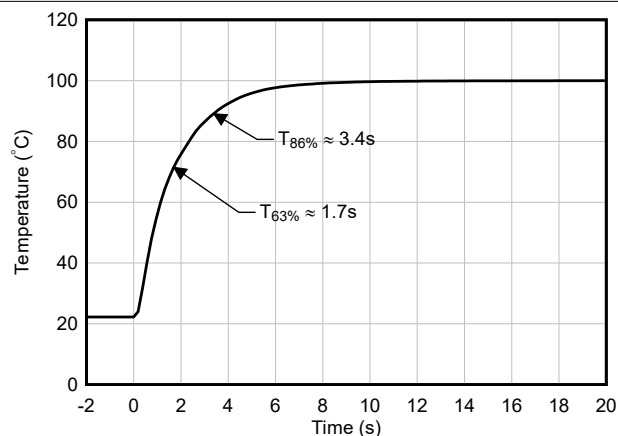
图 6-31. 搅拌油浴中的热响应 (0.5 英寸 × 0.5 英寸 PCB 板)
