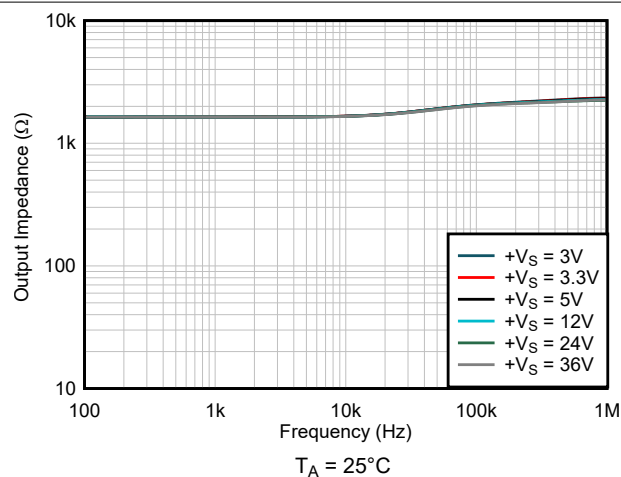
图 6-33. 输出阻抗与频率间的关系
