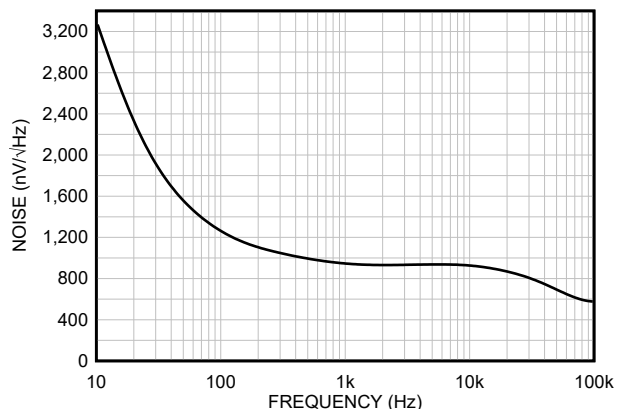
图 6-16. 噪声电压 ( 新芯片 )
