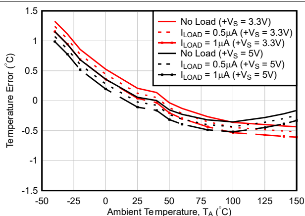
图 6-23. 不同负载下精度与环境温度间的关系
